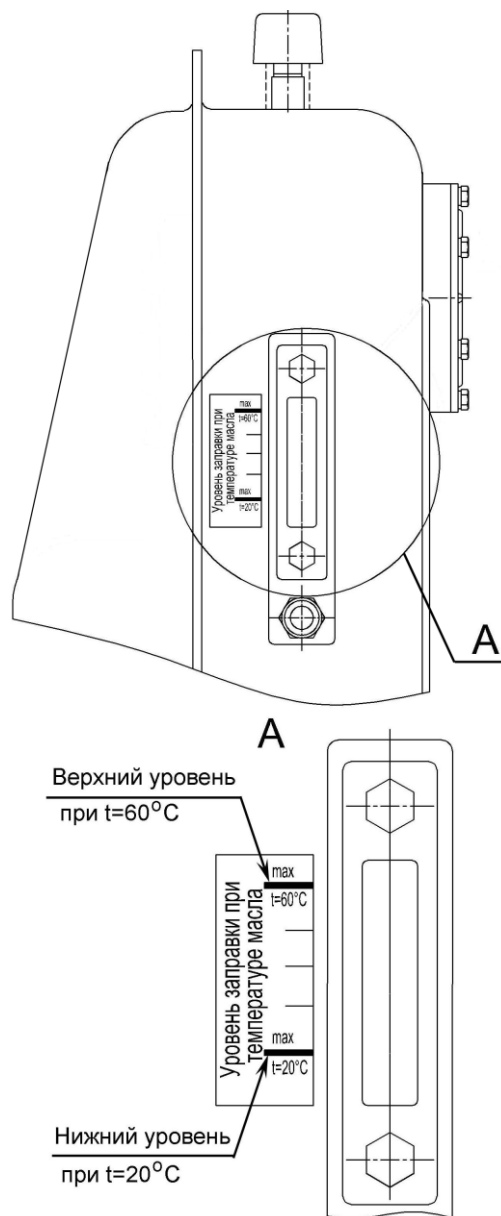
Рисунок 2.6 – Заправка гидросистем
