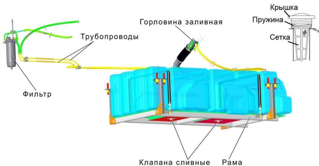
Рисунок 3.11 – Топливная система
