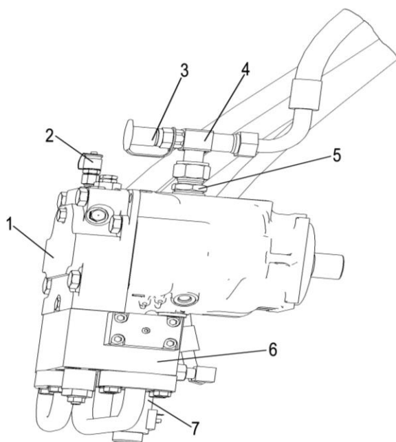
1 – гидромотор привода питающего аппарата; 2 – точка диагностики; 3 - полумуфта заправочная; 4 – тройник; 5 - штуцер; 6 – гидроблок экстренного останова
