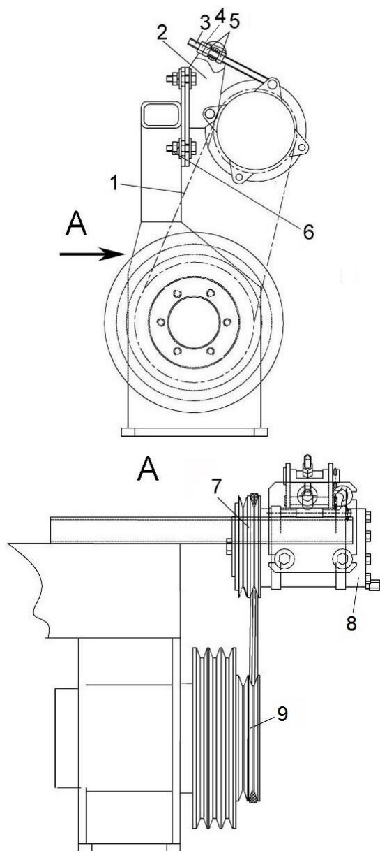
1 – ременная передача; 2 – кронштейн; 3 – тяга; 4 – контргайка; 5, 6 – гайки; 7, 9 – шкивы; 8 – компрессор
