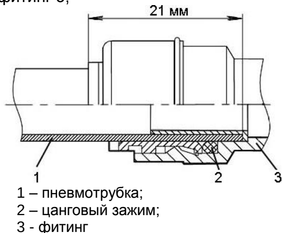
Рисунок 3.20 – Фитинг «цангового» типа
