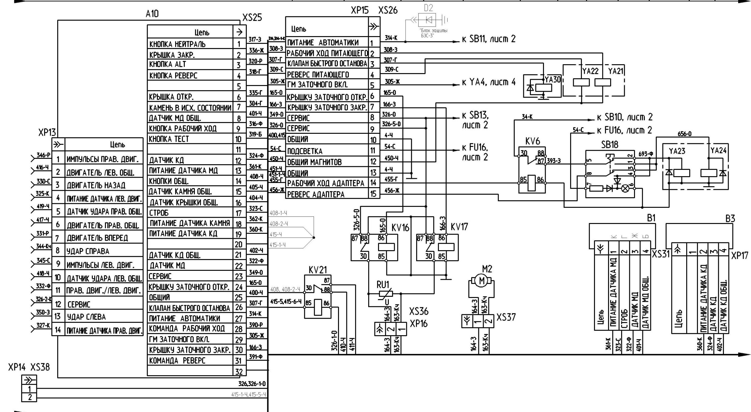
Рисунок Б.5 – Схема электрическая принципиальная комплекса (лист 2)
