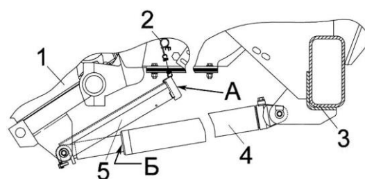
1 – питающе-измельчающий аппарат; 2 – пружина; 3 - балка моста; 4 – гидроцилиндр; 5 – упор; А и Б – опорные поверхности
