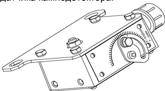
Рисунок 2.7 – Датчик камнедетектора
