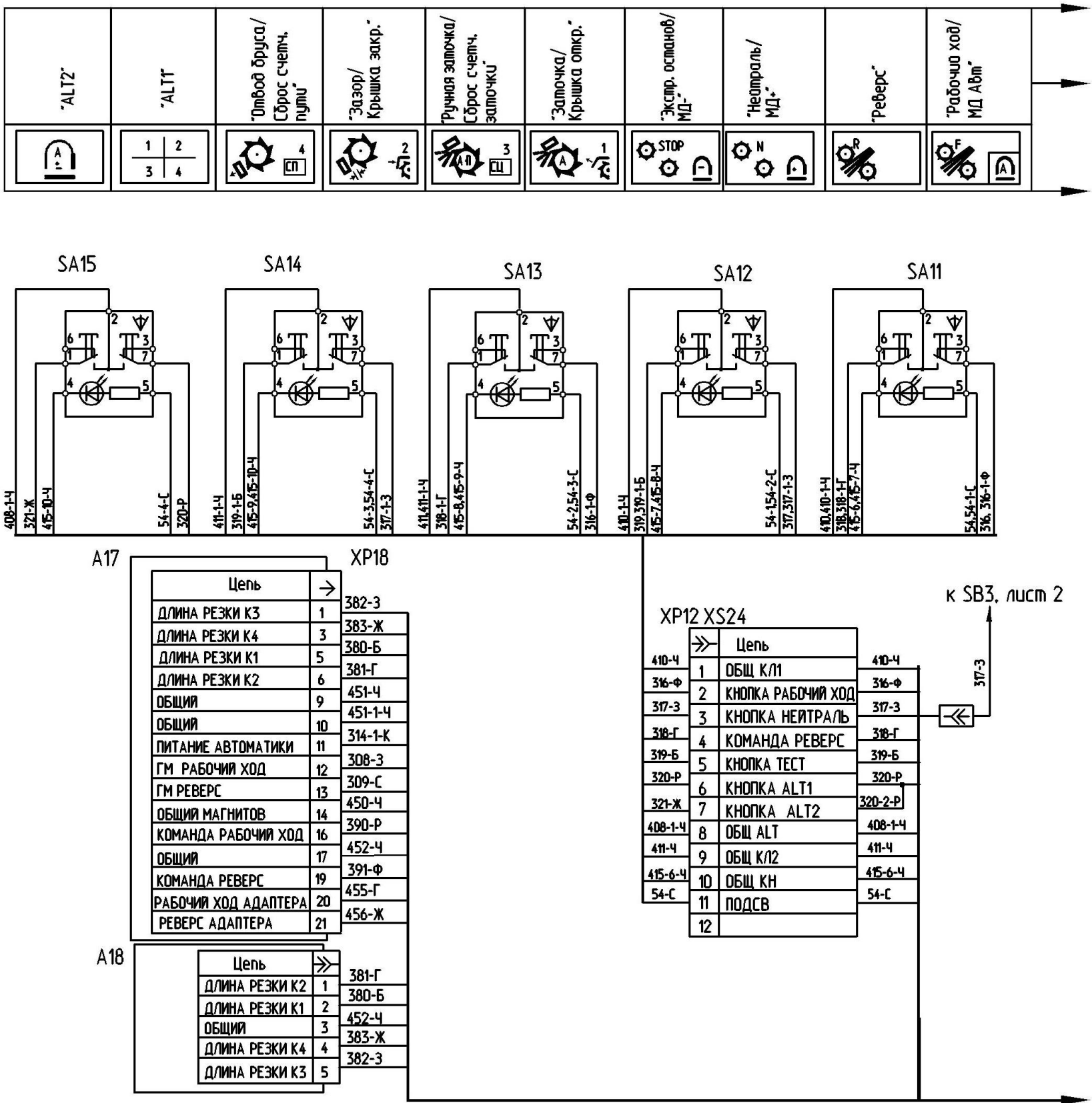
Рисунок Б.5 – Схема электрическая принципиальная комплекса (лист 1)
