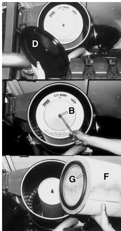
Рисунок 3.8 - Очистка или замена фильтр – патрона воздухоочистителя двигателя
