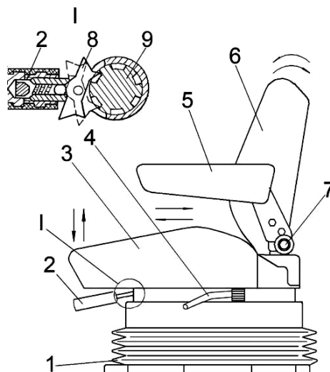
1 – чехол; 2 – рукоятка регулировки сиденья по массе оператора; 3 – подушка сиденья; 4 – рычаг фиксации продольного перемещения сиденья; 5 – подлокотник; 6 – подушка спинки; 7 – маховик регулировки спинки; 8 – собачка; 9 – винт
