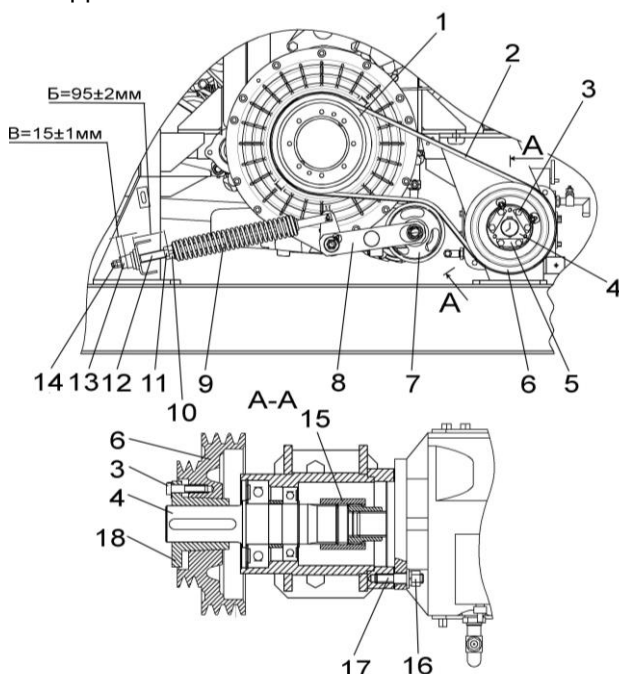
Рисунок 2.19 – Регулировка привода вентилятора
