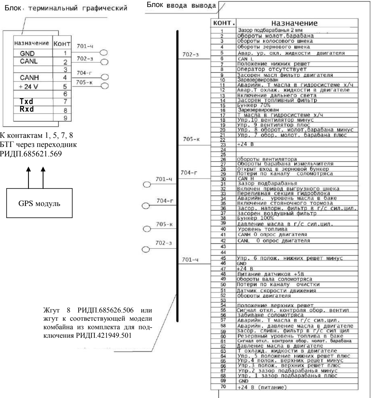
Рисунок 1.146 – Схема подключения БТГ, БВВ и GPS модуля комбайна
