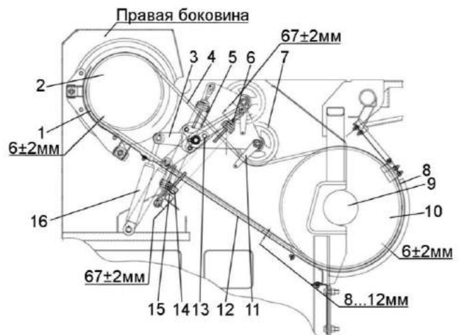
1, 8, 12 – щитки; 2, 10 – шкивы; 3 – рычаг; 4 – ремень; 5 – опора; 6, 13, 15 – гайки; 7 – ролик натяжной; 9 – вал; 11 – кронштейн; 14 – пружина; 16 – гидроцилиндр
