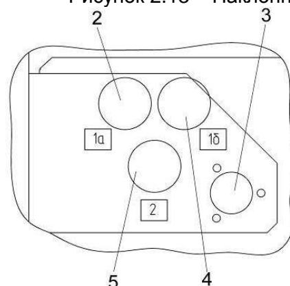
Подсоединение электро и гидровыводов
