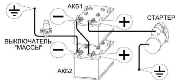
Рисунок 2.2 - Подключение аккумуляторных батарей
