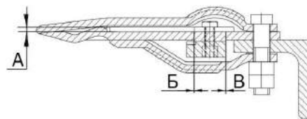
Рисунок 2.42 – Режущий аппарат
