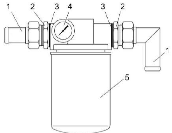
Рисунок 1.28 – Гидросистема привода ходовой части
