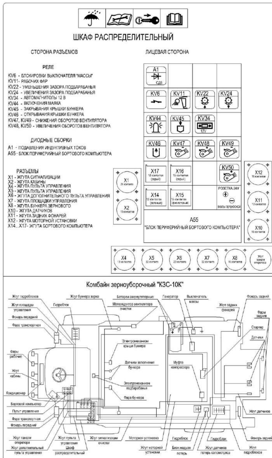
Схема соединений шкафа распределительного представлена на рисунке 1.31
