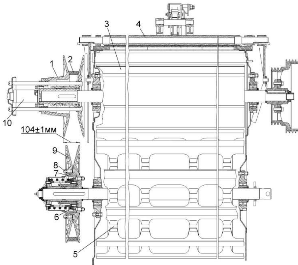
Рисунок 3.11 – Привод молотильного барабана
