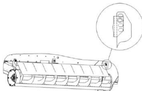
Рисунок 2.21 – Регулировка ограждения над горизонтальным шнеком бункера
