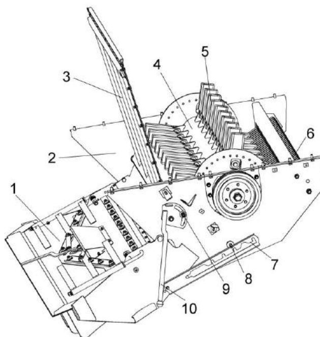
1 – дефлектор; 2 – корпус измельчителя; 3 – заслонка; 4 – ротор измельчителя; 5 – нож; 6 – ножевая опора; 7 – полз; 8, 9 – гайки; 10 - рукоятка сектора
