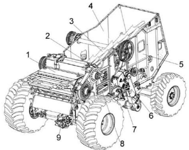
1 - аппарат молотильный; 2 - верхний решетный стан; 3 - соломотряс; 4 - боковина правая; 5 - боковина левая; 6 - элеватор колосовой; 7 - устройство домолачивающее; 8 - стрясная доска; 9 - шасси
