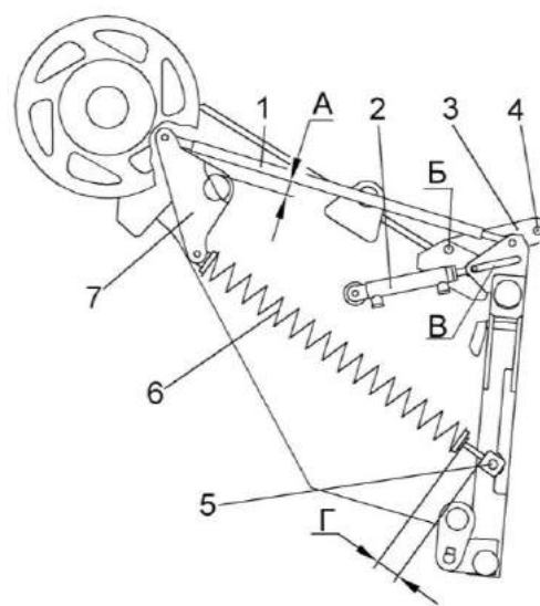
Рисунок 2.9 – Регулировка сферических роликов переходной рамки наклонной камеры
