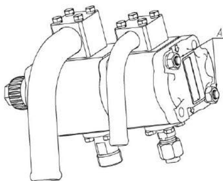
Рисунок 4.1 – Демонтаж гидронасоса
