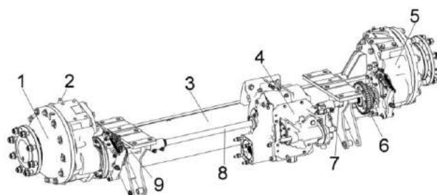
Рисунок 1.15 – Мост управляемых колес.
