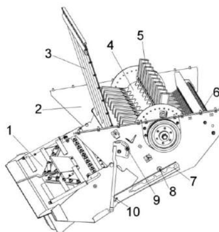
1 – дефлектор; 2 – корпус измельчителя; 3 – заслонка; 4 – ротор измельчителя; 5 – ножи; 6 – ножевая опора; 7 – полоз; 8, 9 – гайки; 10 – рукоятка сектора
