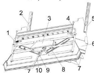
1, 4 – граблины; 2, 5 – полозы; 3 – щиток; 6 – кожух; 7 – лопатки; 8 – планка регулировочная; 9 – планка; 10 – сектор
