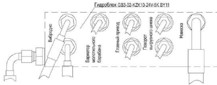
Рисунок 1.25 - Установка гидроблока пятисекционного ГБЗ
