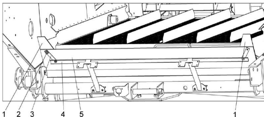
Рисунок 2.19 – Установка дополнительных щитков на нижнем решетном стане
