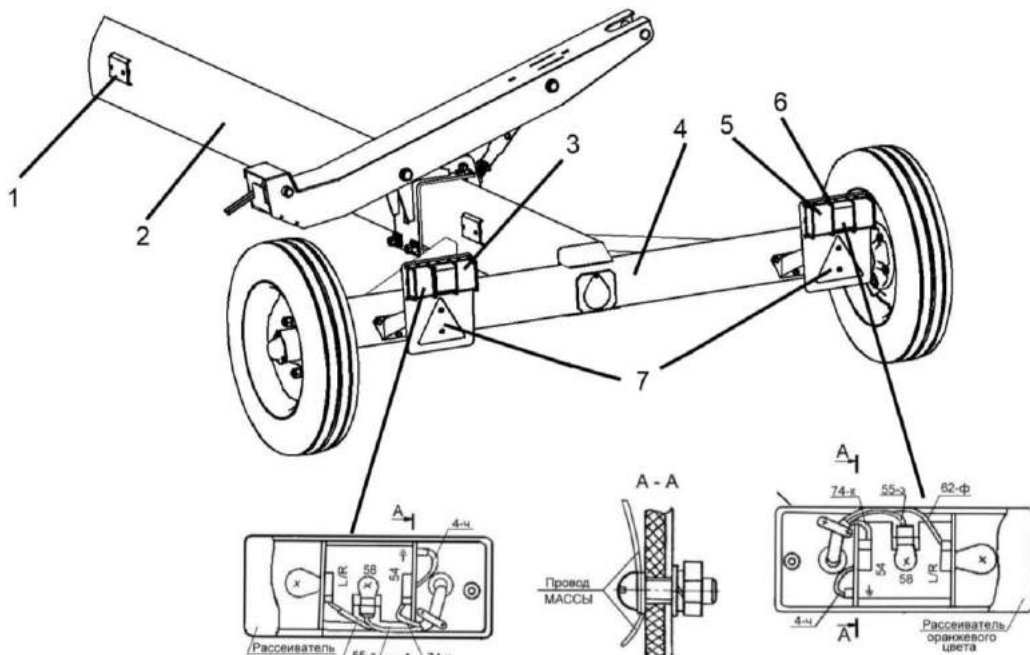
1, 7 - световозвращатели; 2 – рама тележки; 3, 5 - фонари; 4 – балка габаритная; 6 - решетка Условные обозначения цветов проводов: 3 – зеленый; К – красный; Р – розовый; Ф – фиолетовый; Ч - черный фиолетовый; Ч - черный
