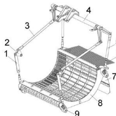
Рисунок 1.12 – Камнеуловитель
