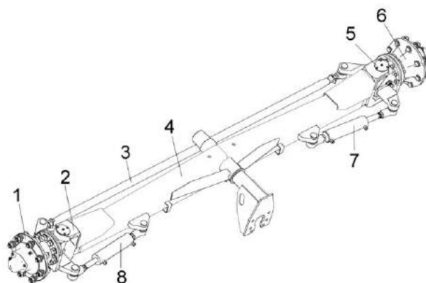
Рисунок 1.14 – Шасси
