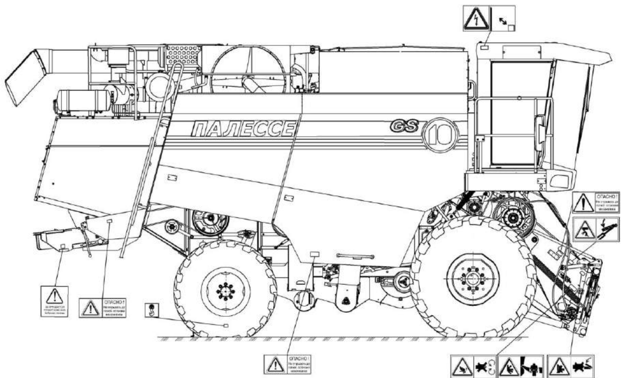
Молотилка самоходная (вид справа)
