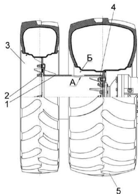
Рисунок 1.17 – Установка спаренных колес
