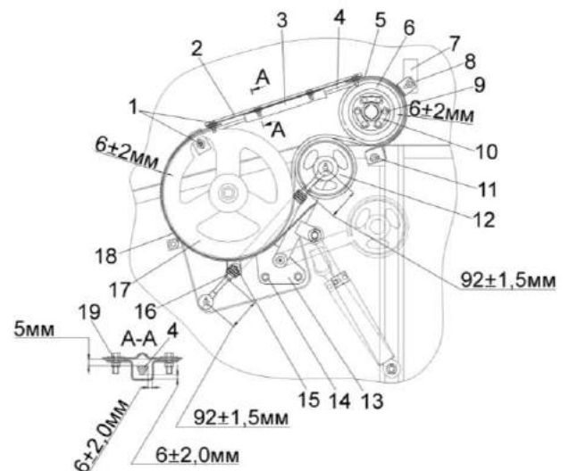
1, 8, 9, 11, 15 – болты; 2, 10 – пластины; 3, 7 – кронштейны; 4 – ремень; 5, 18 – щитки; 6, 17 – шкивы; 12 – рычаг; 13 – опора; 14 – гайка; 16 – пружина; 19 – шайба
