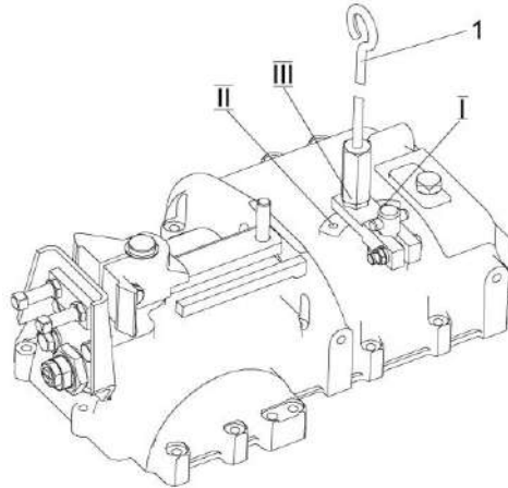
Рисунок 2.22 – Трехскоростная коробка
