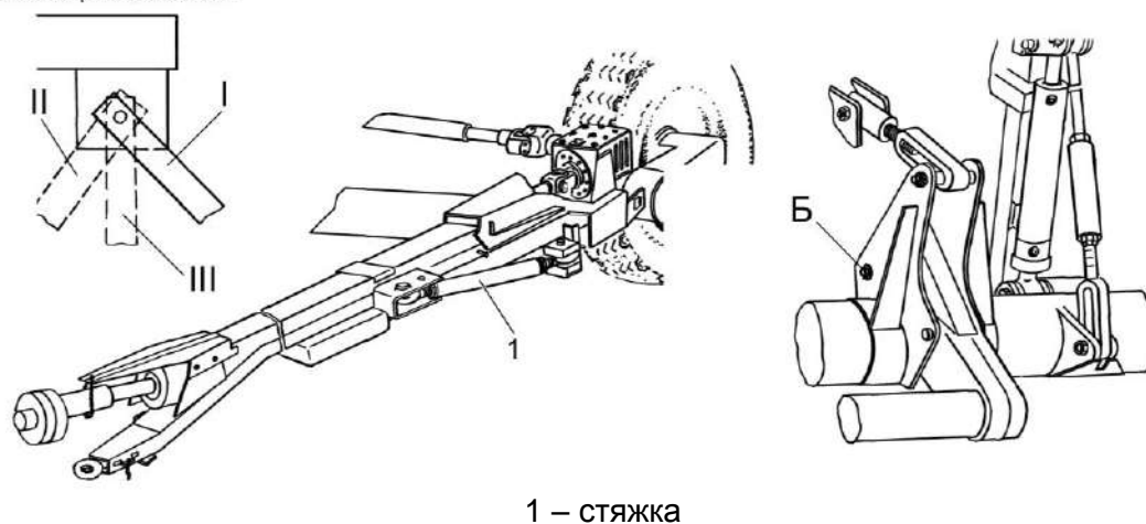
Рисунок 2.21 – Перевод сницы в рабочее положение
