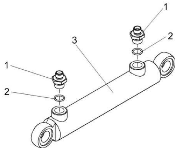
Рисунок 244 – Гидроцилиндр КЗК-12-0602310
