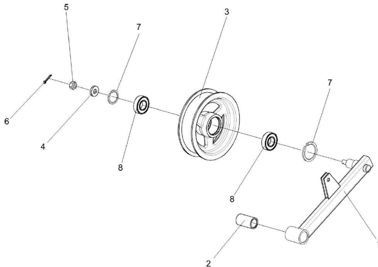
Рисунок 124 – Рычаг КЗК-10-0290260
