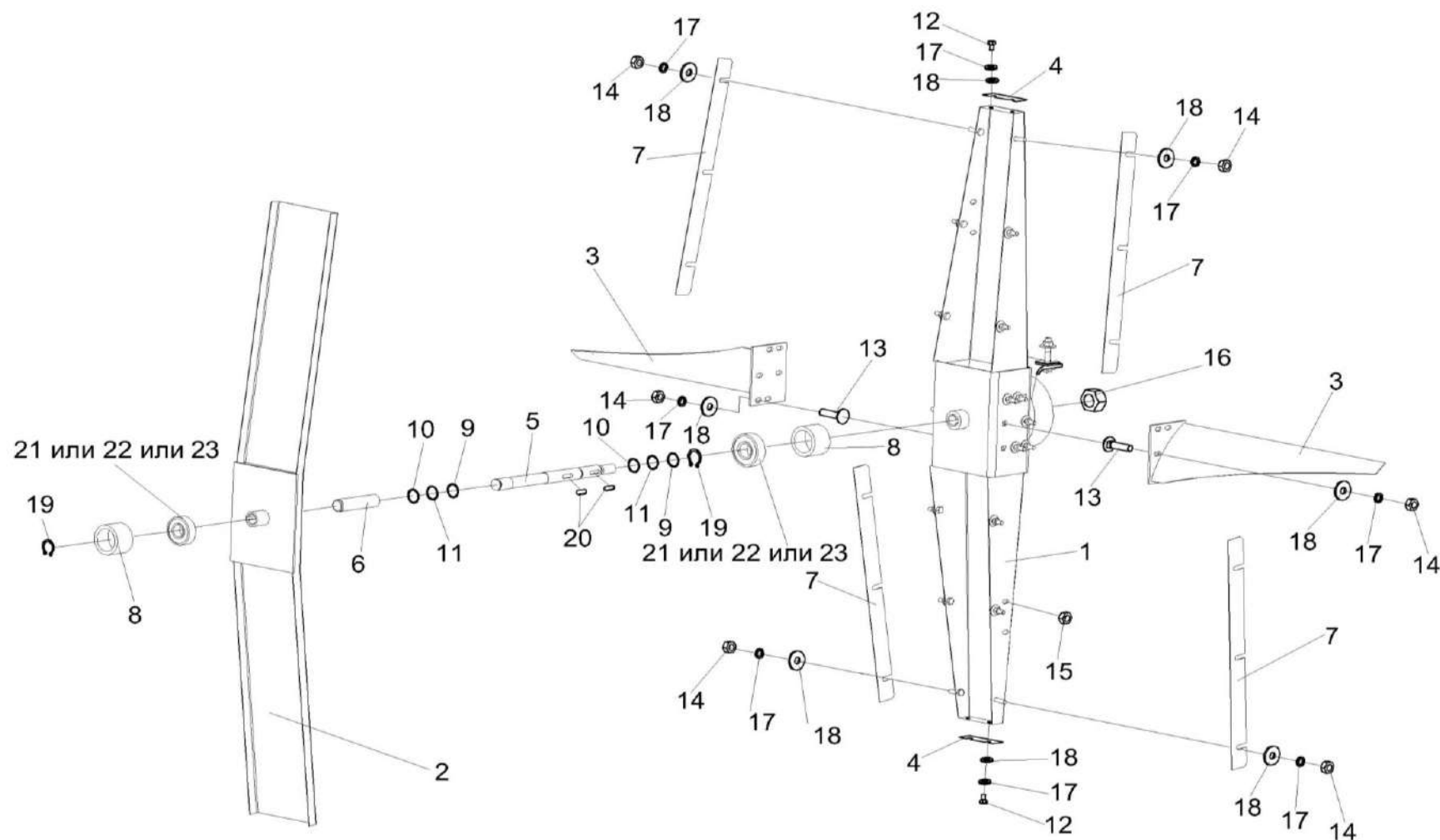
Рисунок 192 – Пылесъемник КЗК-12-3-0112130А
