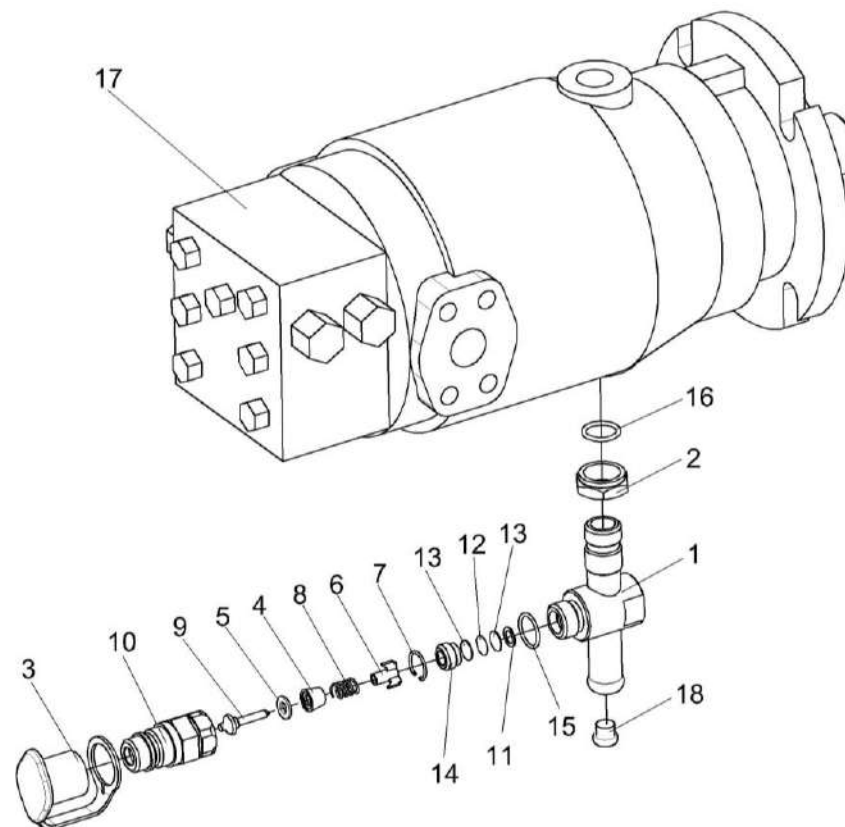
Рисунок 240 – Гидромотор КЗК-12-0601500-01
