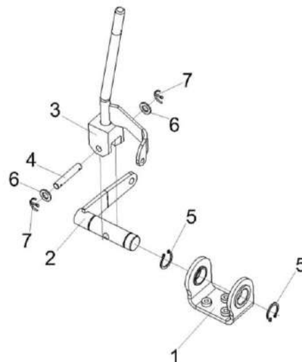
Рисунок 158 – Привод КЗК-3219-0119380
