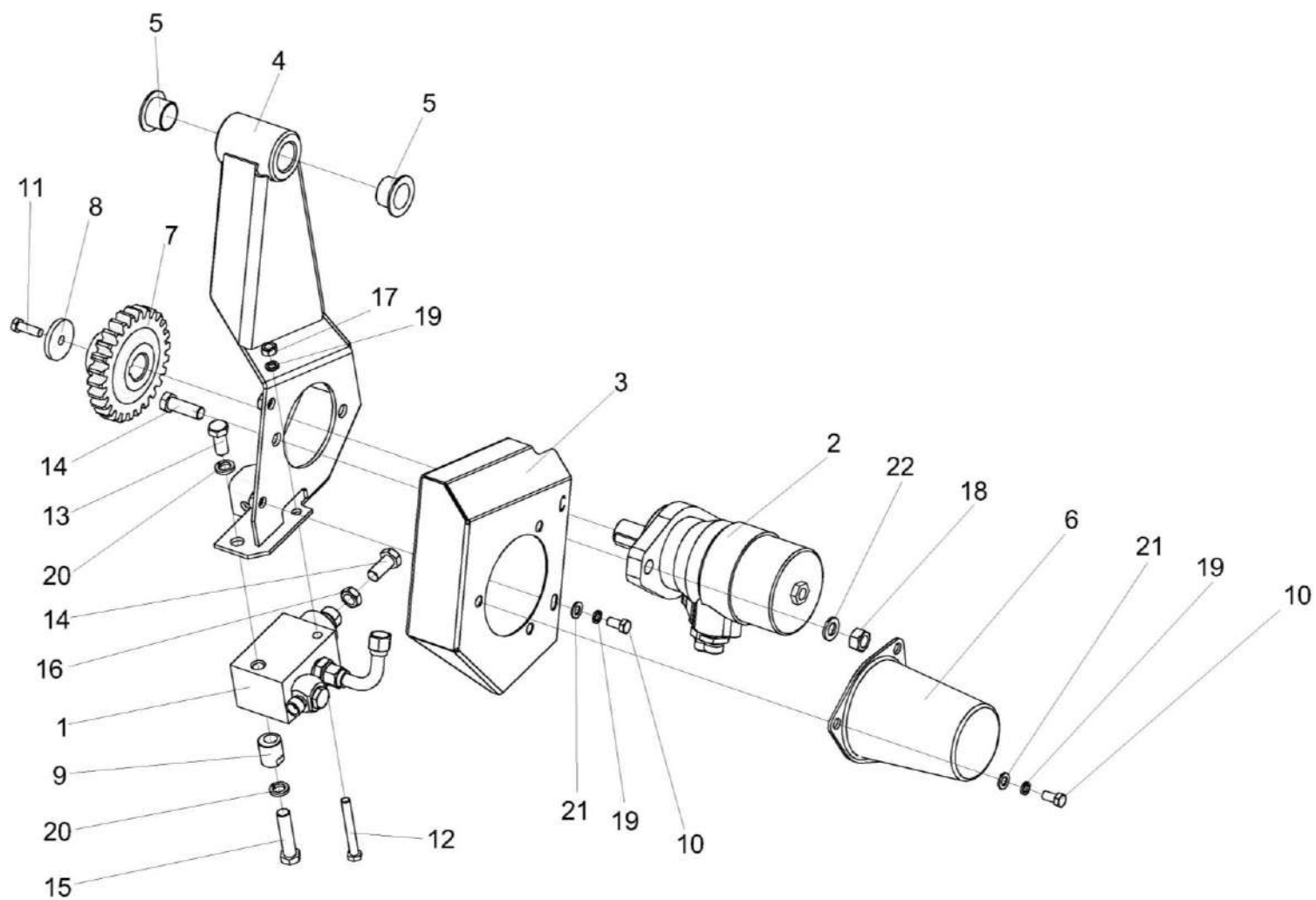
Рисунок 14 – Гидрореверс КЗК-12-1804100
