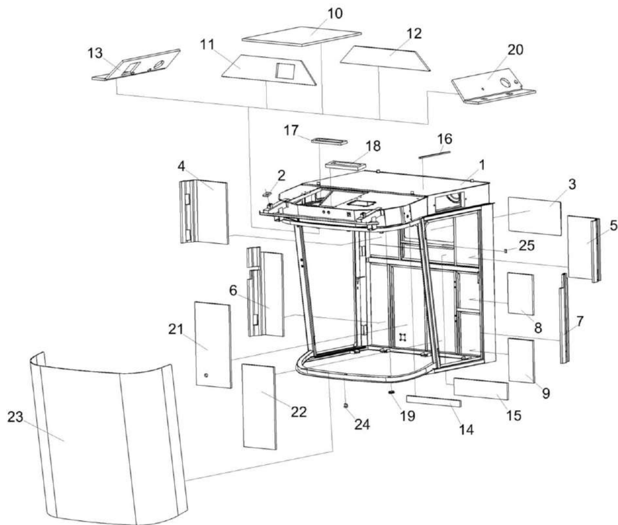
Рисунок 131 – Каркас КЗК-3219-0120020
