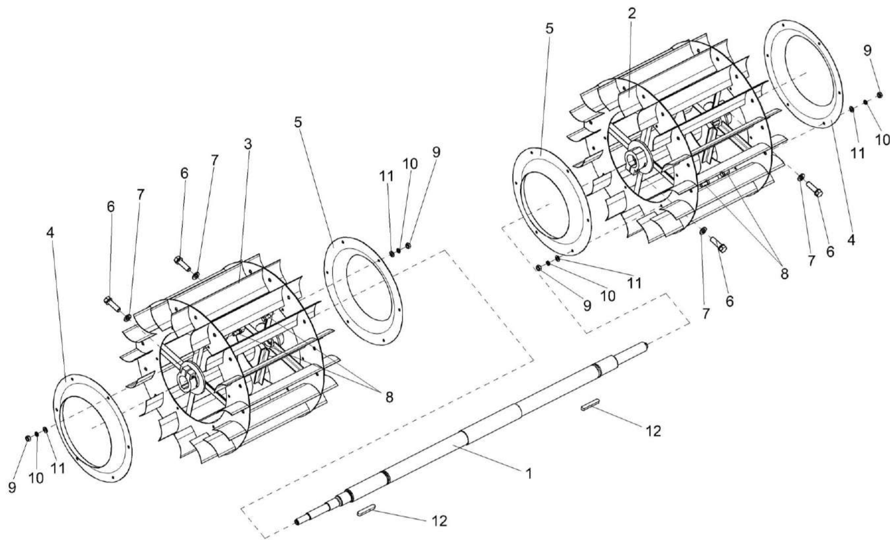
Рисунок 75 – Крылач КЗК-10-0217020А
