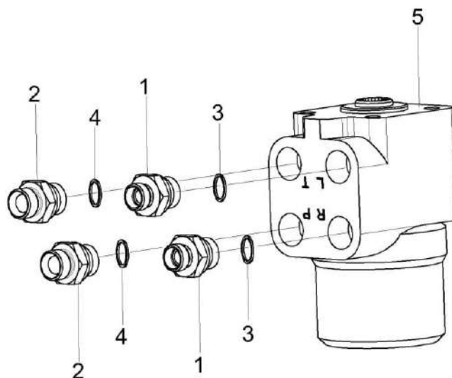
Рисунок 243 – Насос-дозатор КЗК-12-16-0602100
