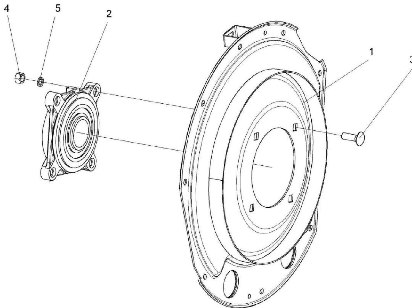
Рисунок 32 – Фланец КЗК-12-0102200
