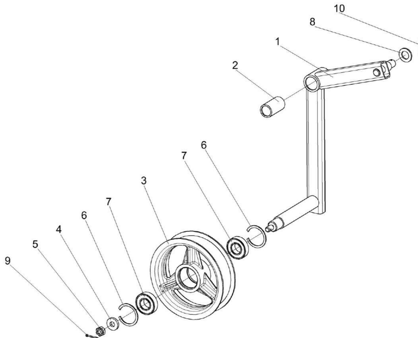
Рисунок 49 – Рычаг КЗК-10-0202440
