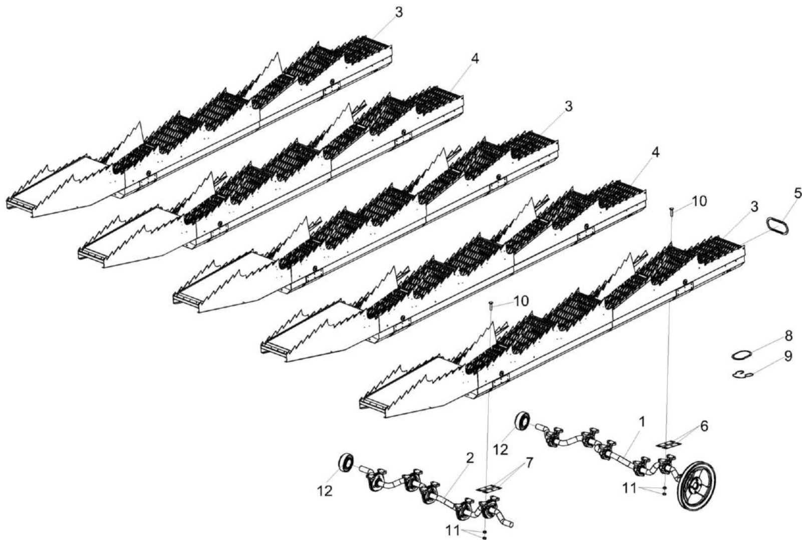
Рисунок 41 – Соломотряс КЗК-12-0212040-01
