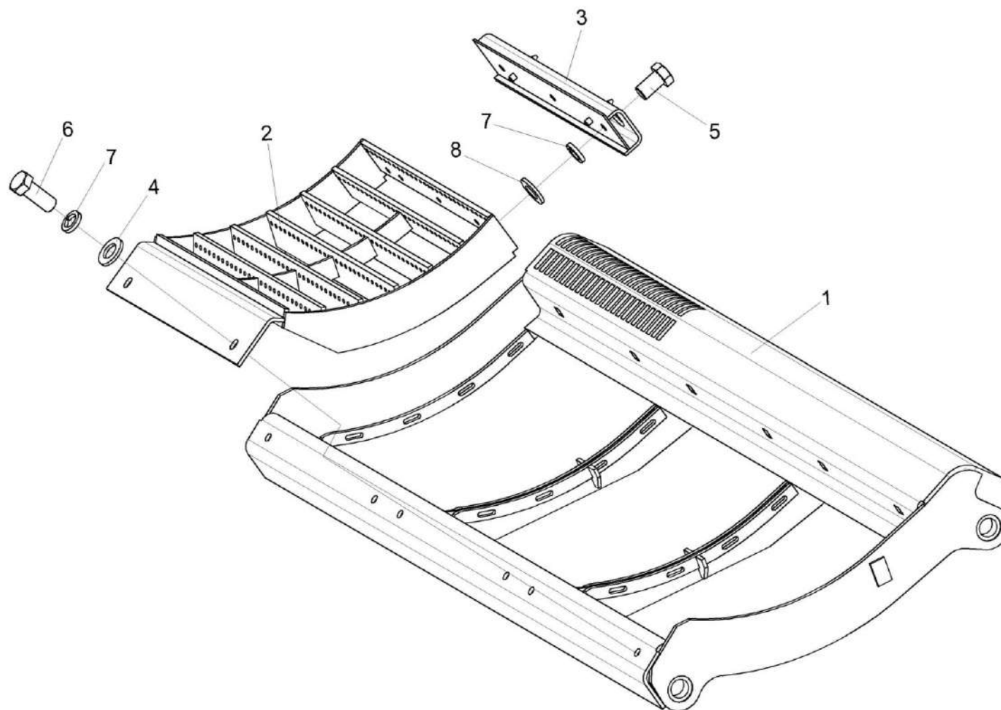
Рисунок 35 – Подбарабанье КЗК-12-0103030-01
