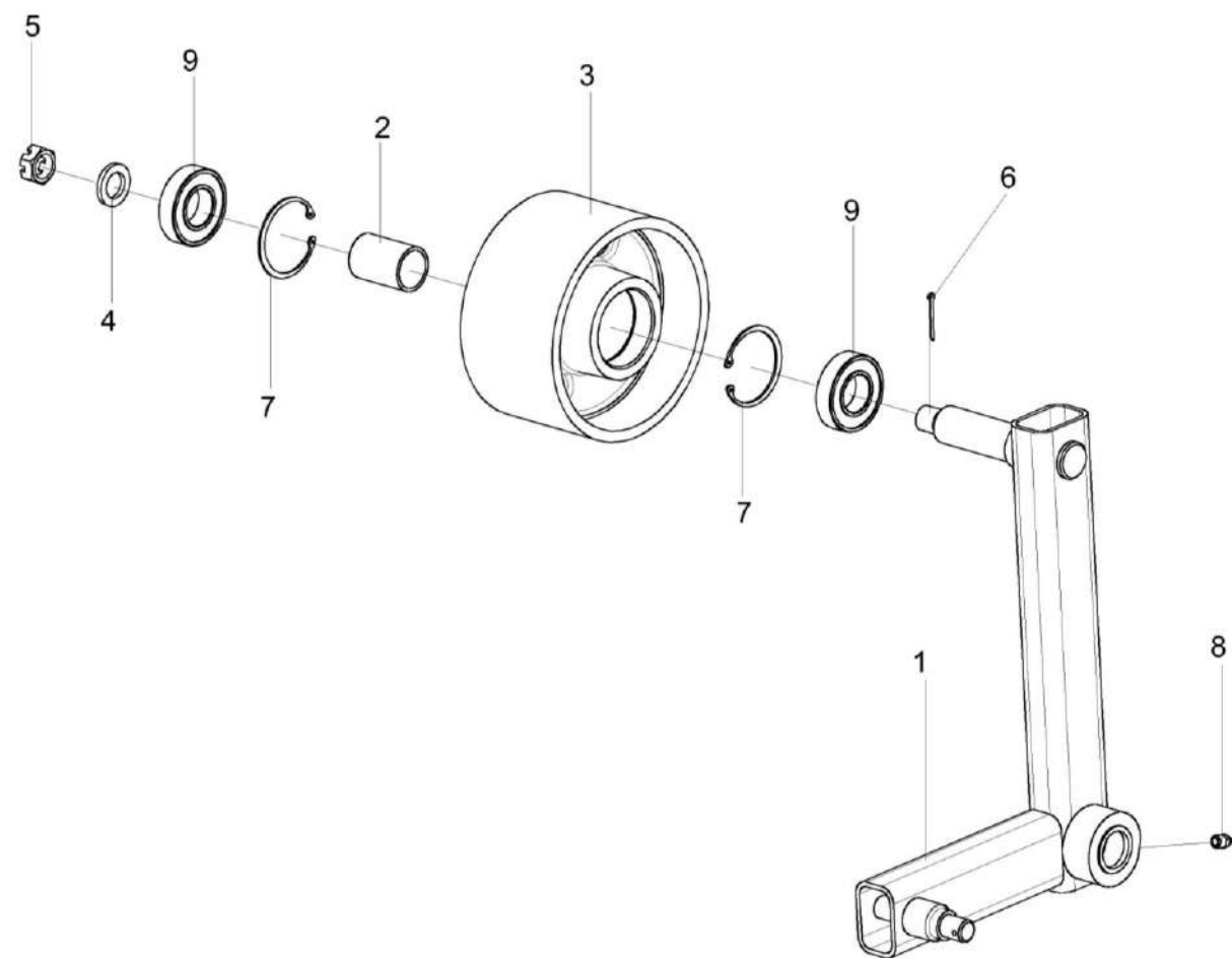
Рисунок 231 – Рычаг КЗК-10-0100590
