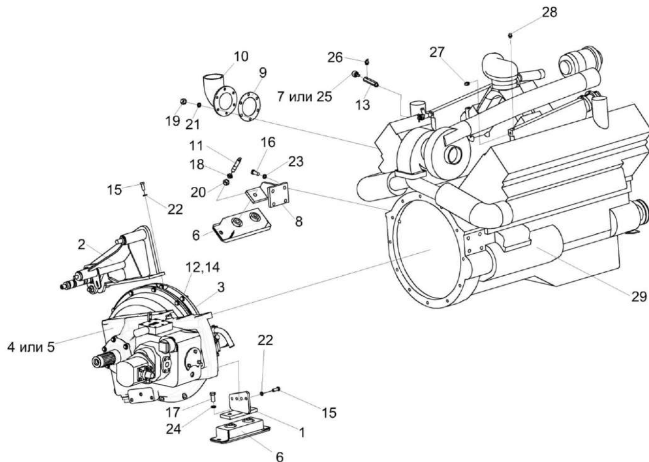
Рисунок 176 – Двигатель КЗК-12-3-0106010Б-01 (лист 2)
