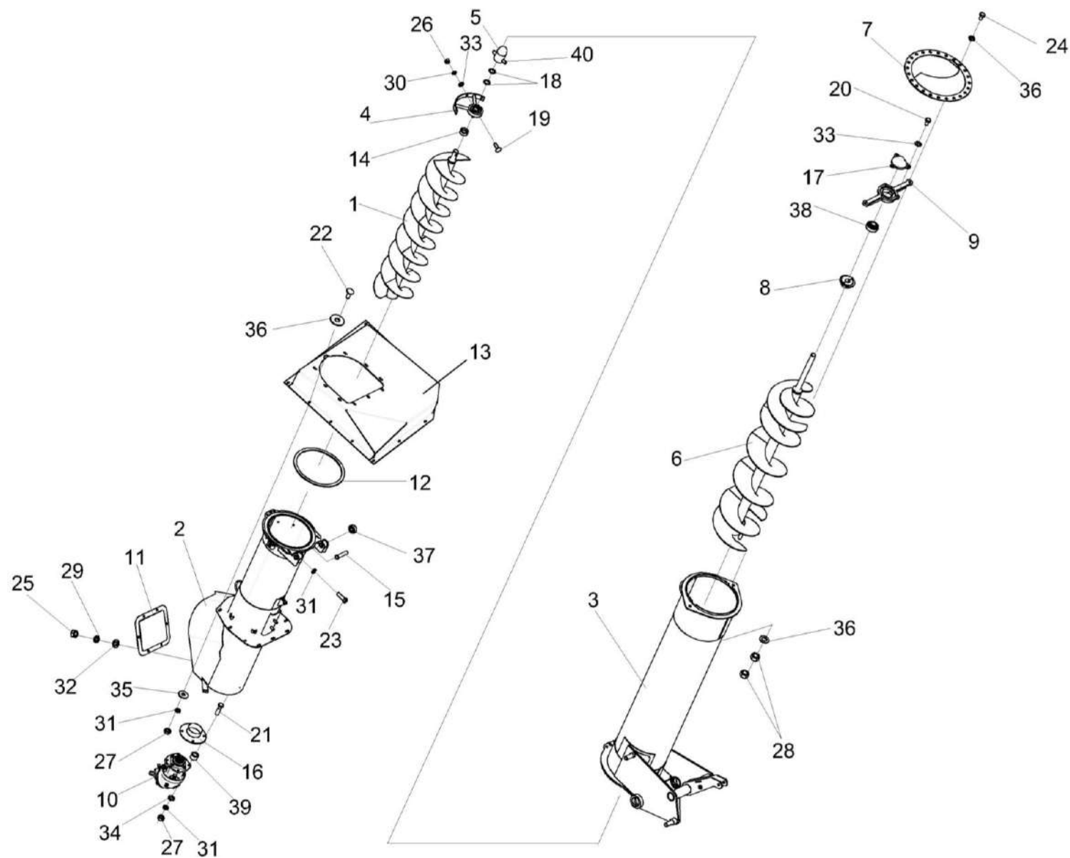
Рисунок 94 – Шнек загрузной КЗК-3321-1-0216010
