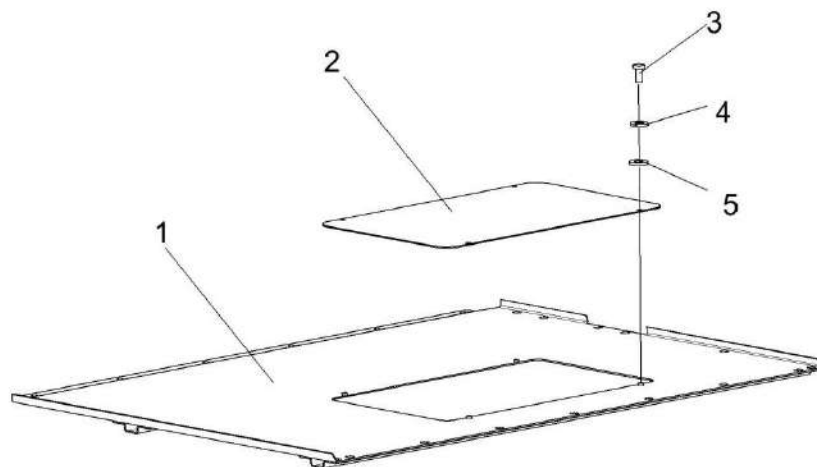
Рисунок 217 – Настил КЗК-12-0100320А
