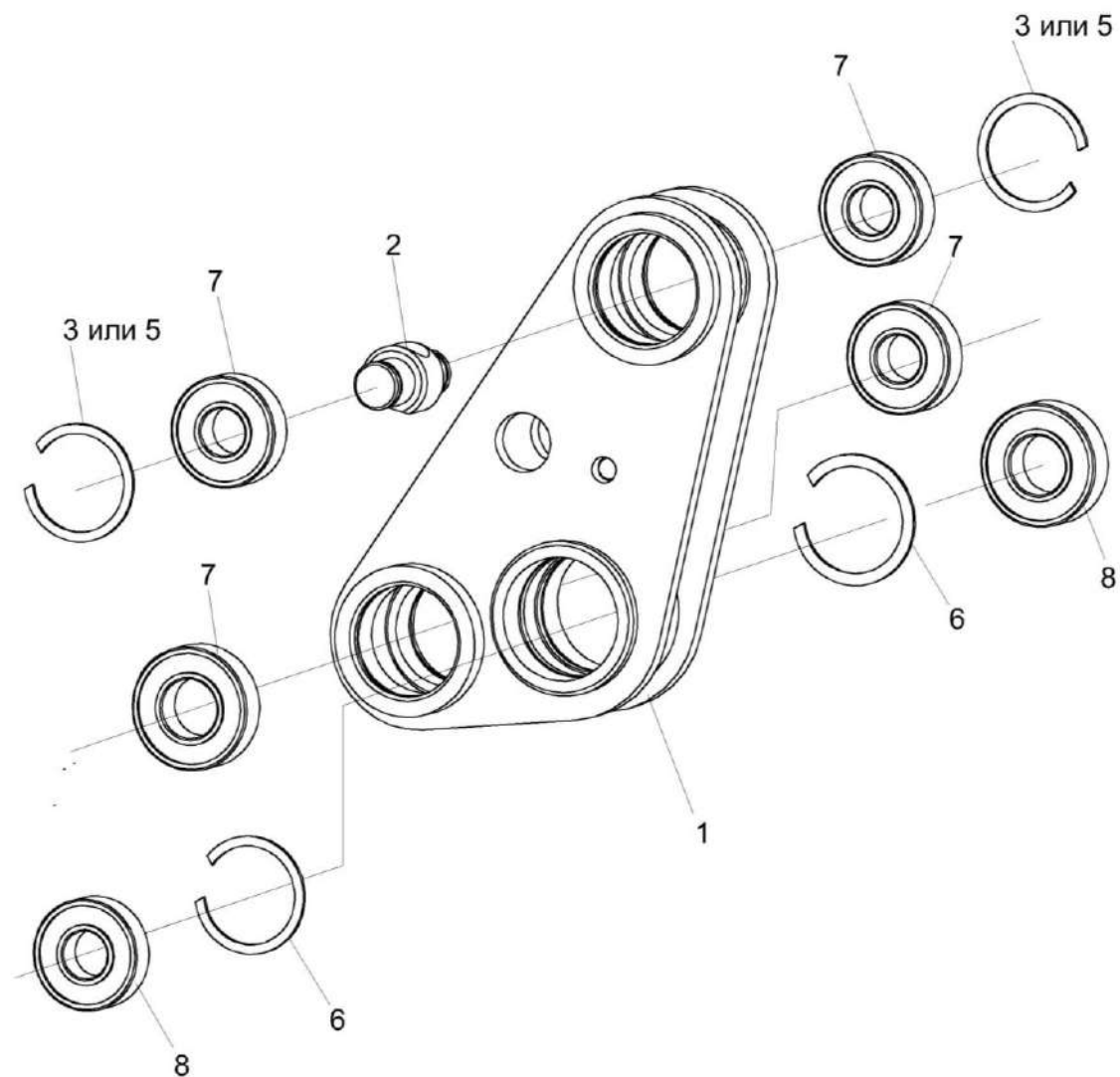
Рисунок 24 – Рычаг КЗК-12-1808500
