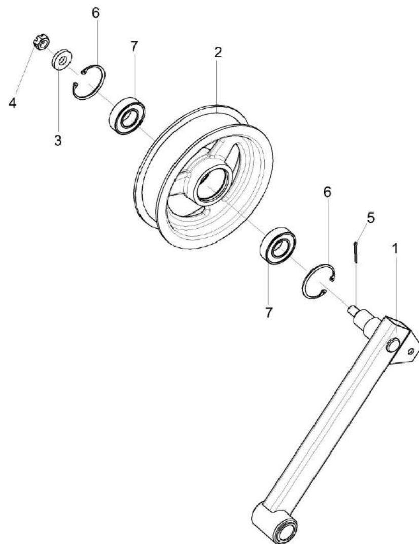
Рисунок 232 – Рычаг КЗК-10-0100620
