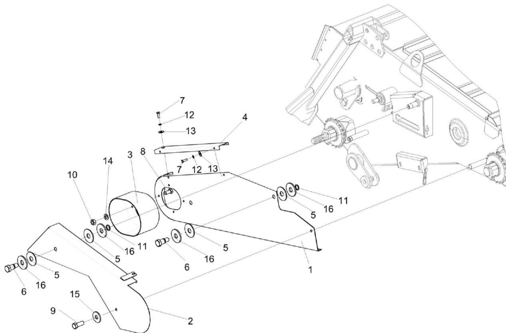
Рисунок 12 – Установка ограждений КЗК-12-1800140 и КЗК-12-1800160
