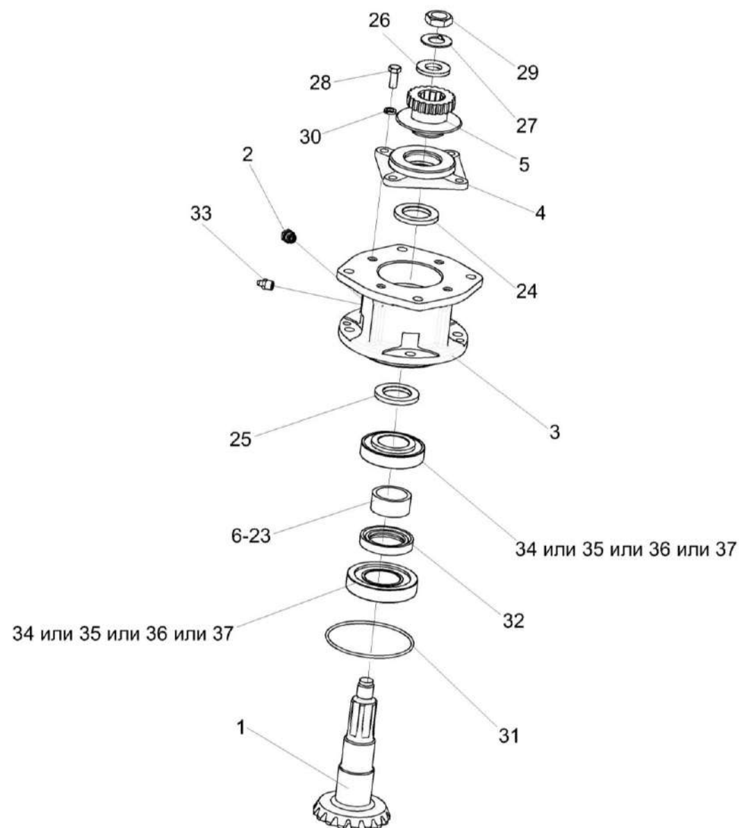
Рисунок 96 – Стакан КЗК-3321-1-0245010
