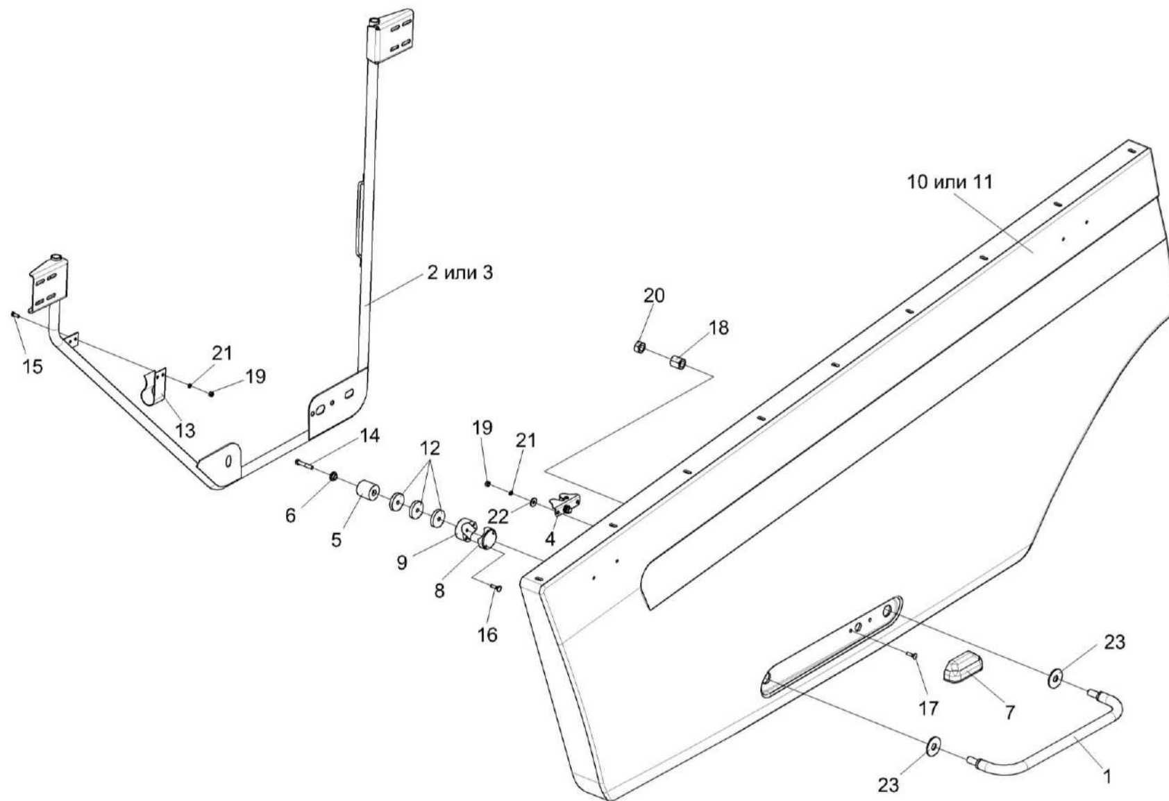
Рисунок 213 – Кожух боковой КЗК-12А-1-0128530 и КЗК-12А-1-0128530-01
