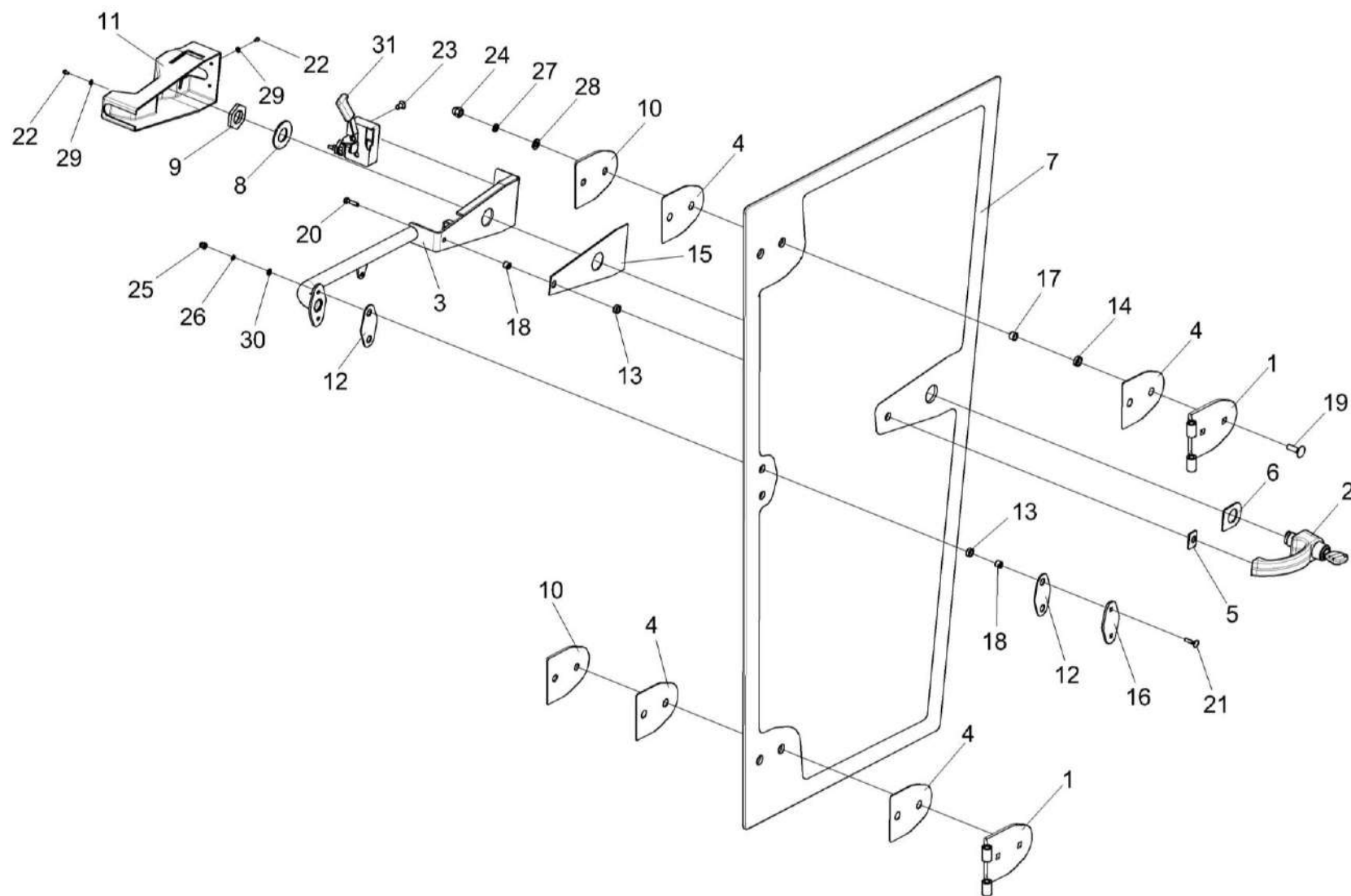
Рисунок 132 – Дверь КЗК-12-0131070
