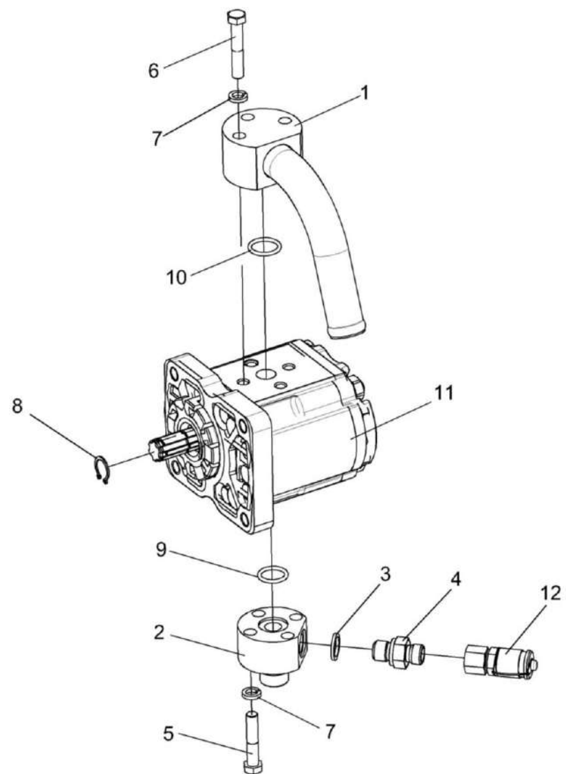
Рисунок 183 – Насос КЗК-12-0602890
