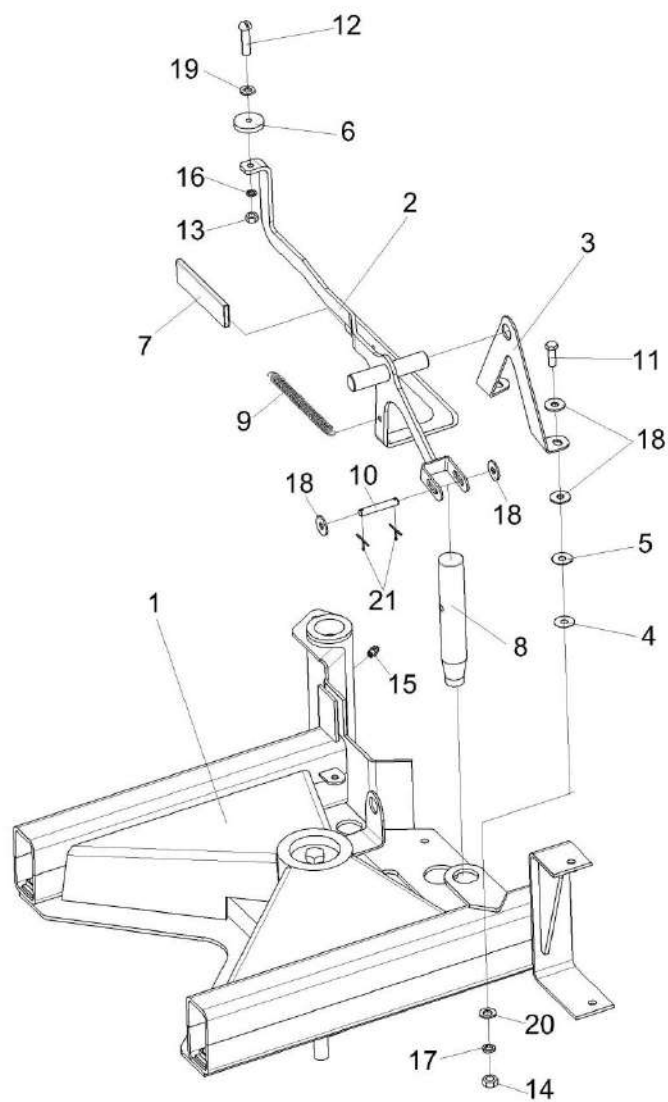
Рисунок 169 – Рама КЗК-12-0117010Б
