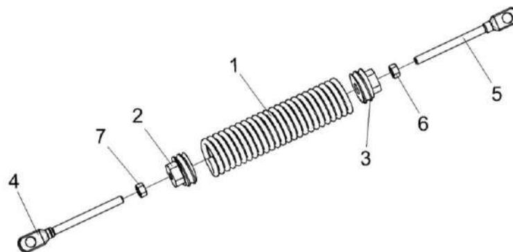
Рисунок 206 – Пружина КЗК-12-3-0220050
