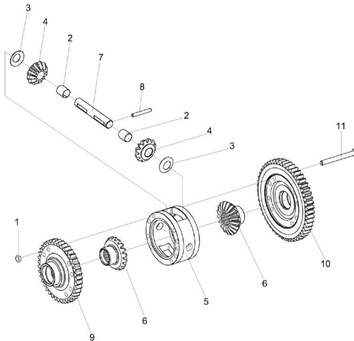
Рисунок 66 – Дифференциал КЗК-12-0107540
