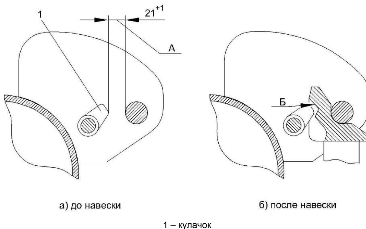
Рисунок 2.3 – Перекрывание кулачка и упора гидроцилиндра в зафиксированном верхнем ловителе жатки
