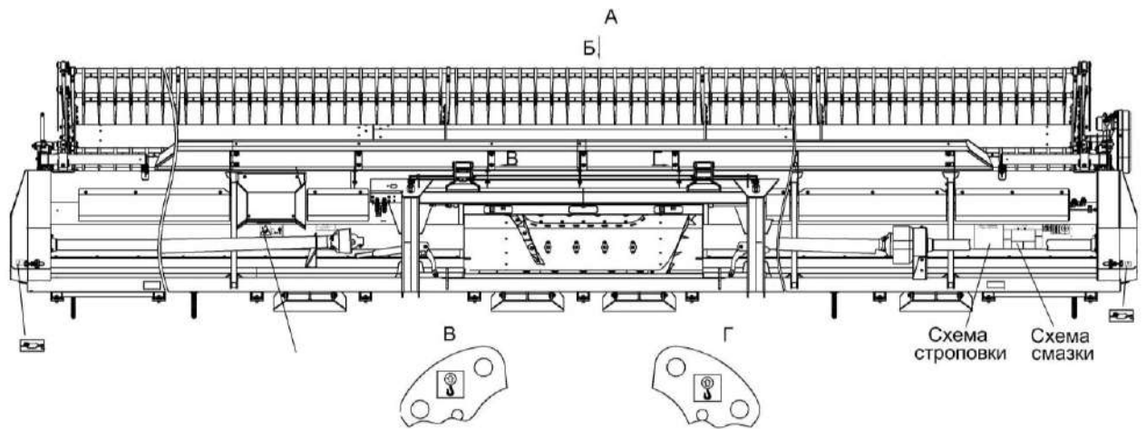
Жатка (вид слева)
