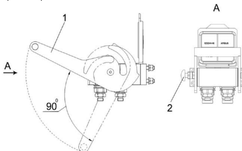
Рисунок 2.7 – Положение рукоятки разъёма гидравлического многофункционального
