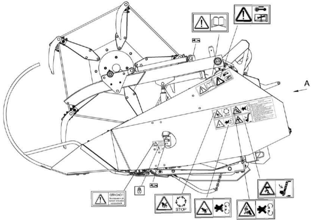
Жатка (вид слева)
