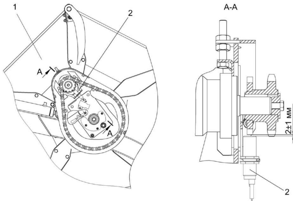
Рисунок 2.20 – Регулировка датчика оборотов мотовила
