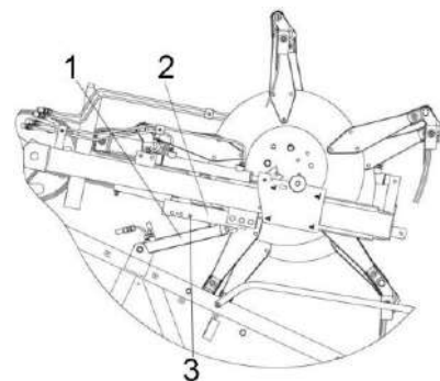
Рисунок 2.36 – Схема установки мотовила
