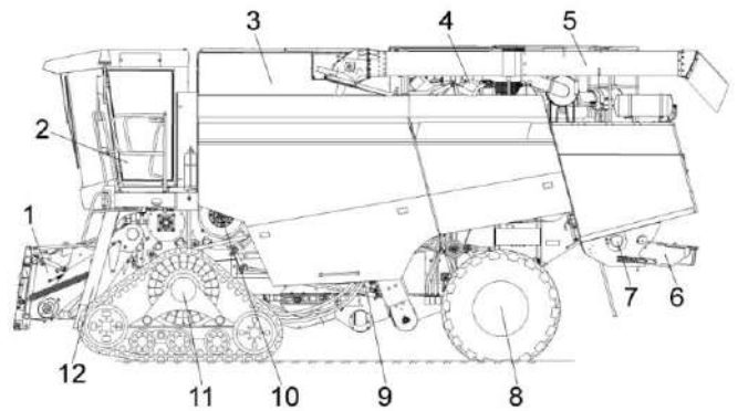
1 – наклонная камера; 2 - кабина; 3 – бункер зерновой; 4 - установка двигателя; 5 – шнек выгрузной; 6 - дефлектор; 7 - соломоизмельчитель; 8 – мост управляемых колес; 9 - очистка; 10 – молотильный аппарат; 11 – ведущий гусеничный ход; 12 - трап
