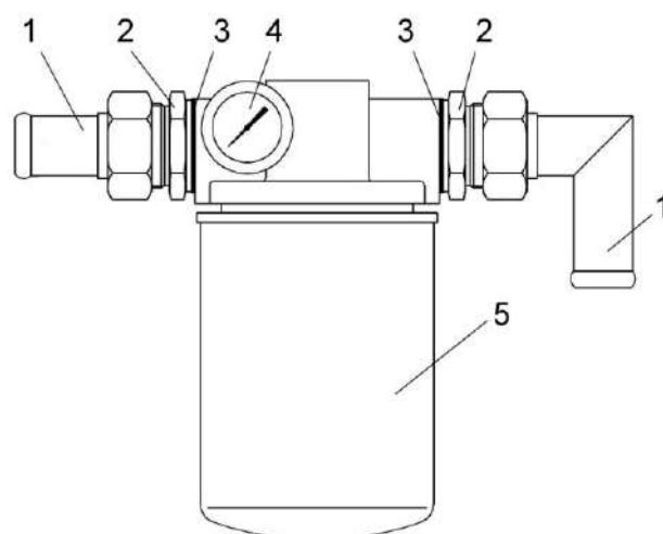
Рисунок 1.26 – Фильтр всасывающий
