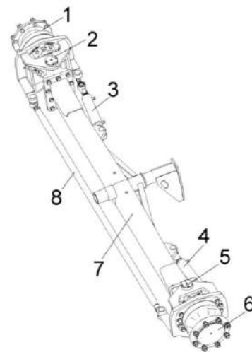
1, 6 – ступицы; 2, 5 - поворотные кулаки; 3, 4 – гидроцилиндры; 7 – балка; 8 – рулевая тяга
