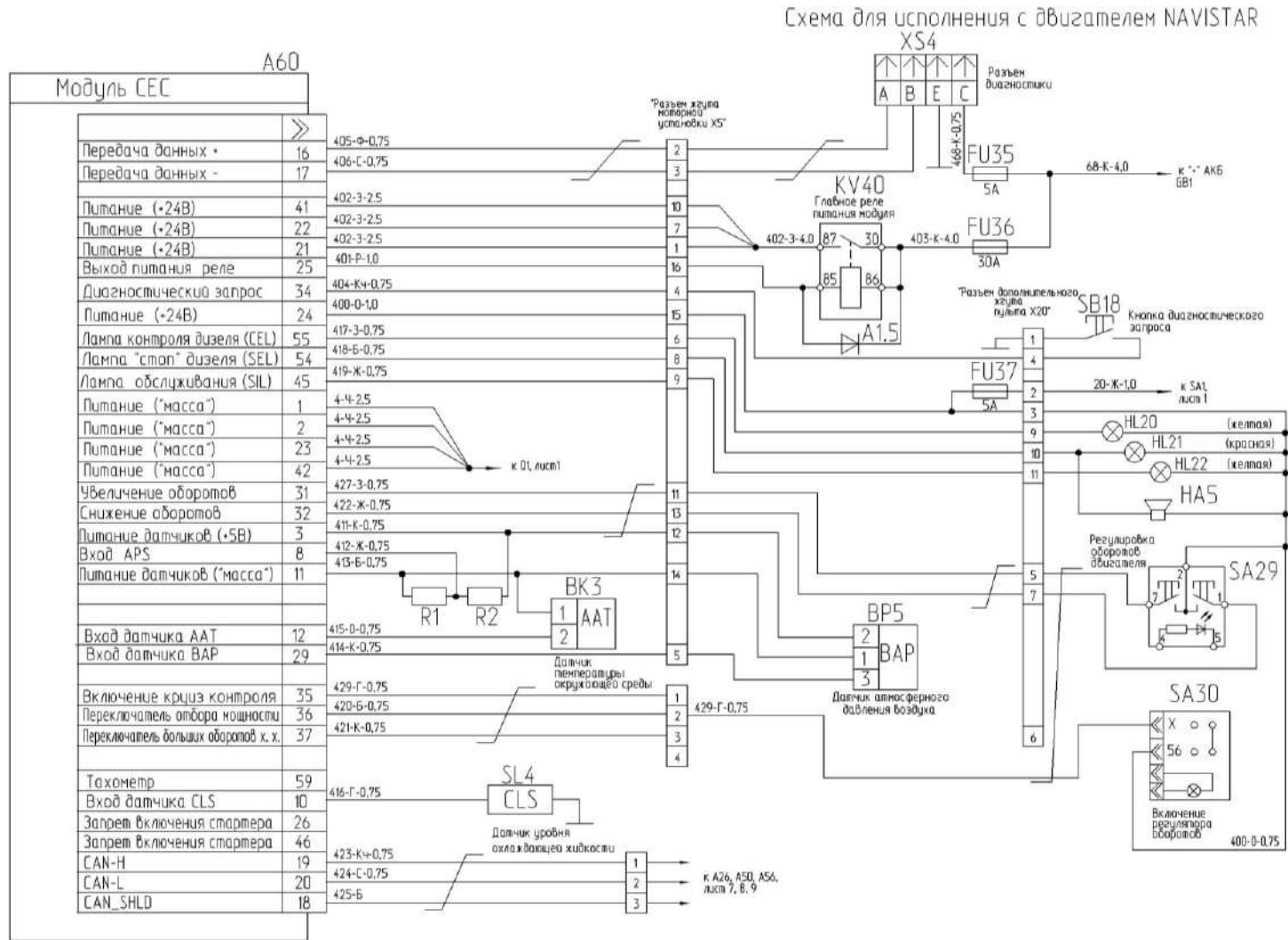
Рисунок Б.6 – Схема электрическая принципиальная комбайна (лист 6)
