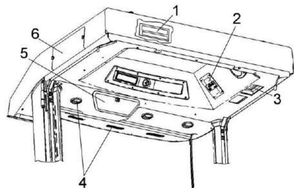
1 – крышка блока предохранителей; 2 – панель управления кондиционером; 3 – фильтр рециркуляции воздуха; 4 – дефлекторы; 5 – охлаждаемый бокс; 6 – место установки воздушного фильтра
