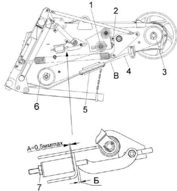
1, 3, 6 – звездочки; 2 – винт; 4 – цепная передача; 5 – успокоитель; 7 - гайка В - стрела провисания ветви цепи
