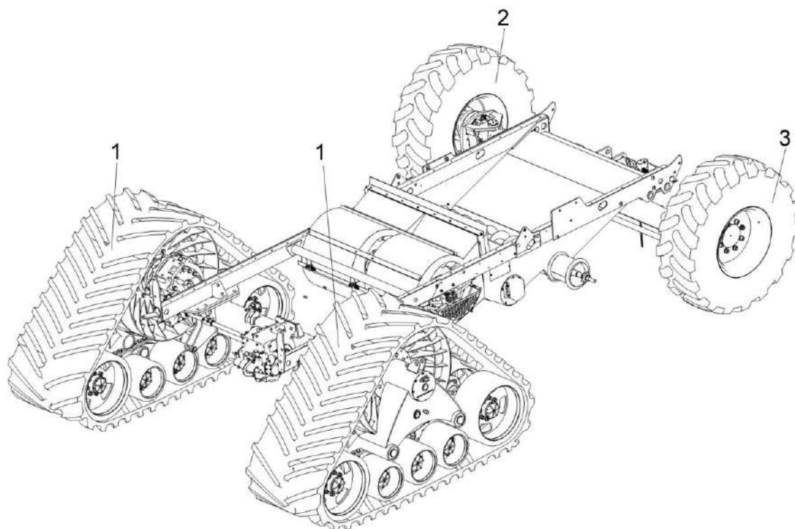
Рисунок 1.17 – Установка гусеничного хода
