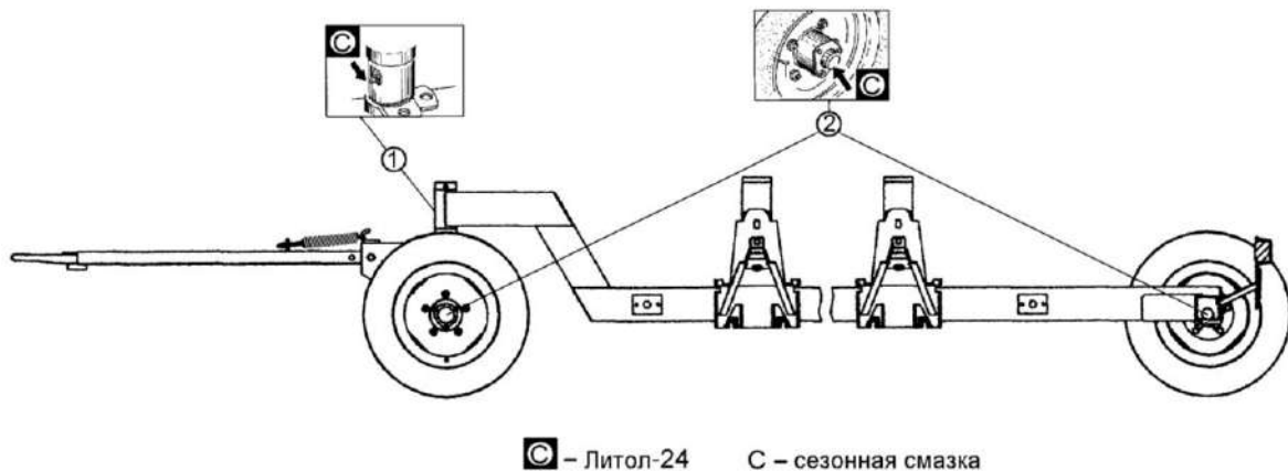
Рисунок 3.5 – Схема смазки транспортной тележки
