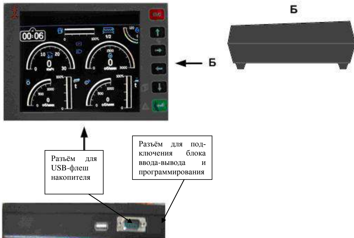
Рисунок К.1 – Внешний вид лицевой панели БТГ
