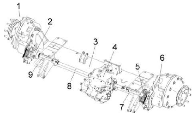
1, 6 – бортовые редуктора; 2, 5 – муфты; 3 – балка; 4 – коробка передач; 7, 8, 9 - полуоси
