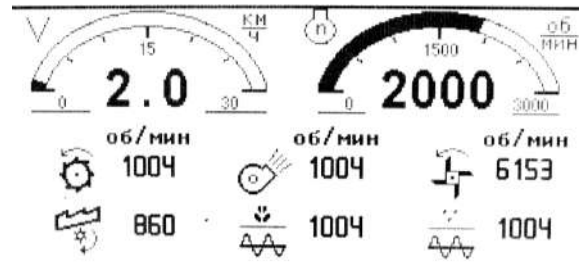
Рисунок И.5 – Экран оборотов рабочих органов
