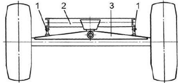
1 – болты; 2 – труба рамы; 3 – балка моста управляемых колес
