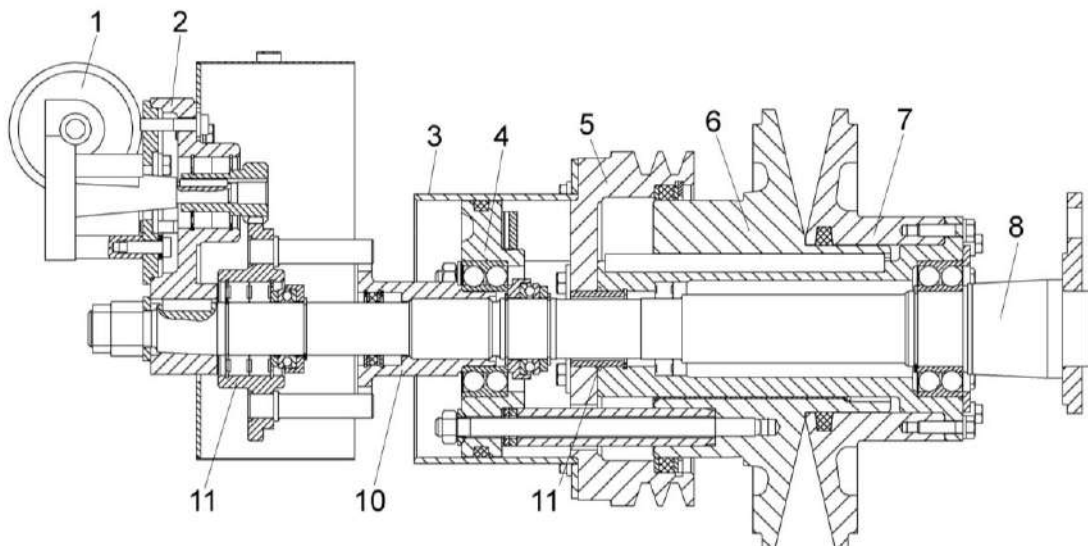
1, 2 – привод; 3 - кожух; 4 – упор; 5, 6, 7 – шкивы; 8 – ось; 9, 10 – втулки; 11 – колесо
