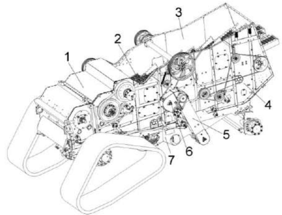
1 – молотильный аппарат; 2 – соломотряс; 3 – боковина правая; 4 – боковина левая; 5 – элеватор колосовой; 6 – устройство домолачивающее; 7 – шасси
