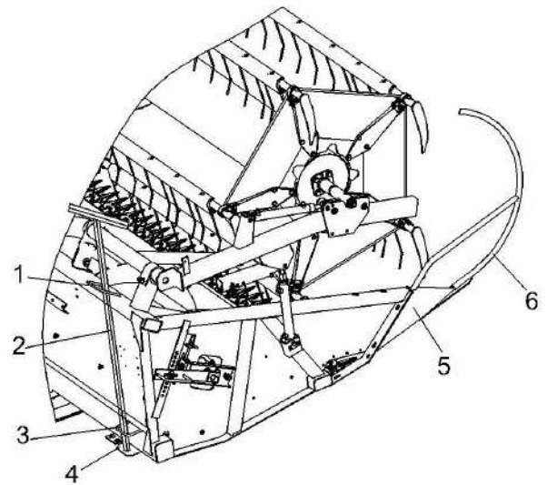
1- верхняя скоба; 2 - швабры; 3 - нижняя скоба; 4 - площадка; 5 - носок; 6 - делитель прутковый
