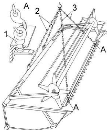
Рисунок 6.1 – Схема строповки молотилки самоходной
