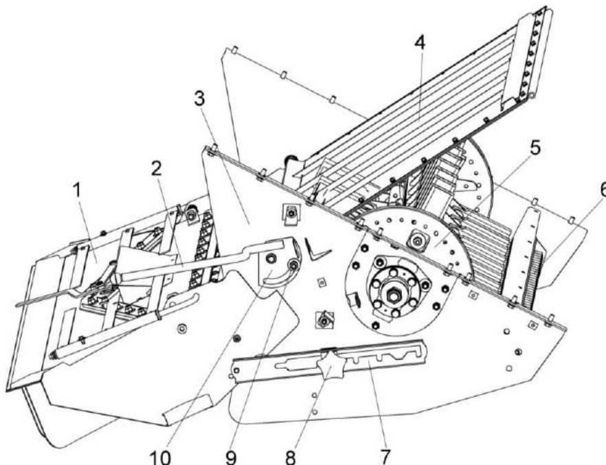
Рисунок 1.20 – Соломоизмельчитель
