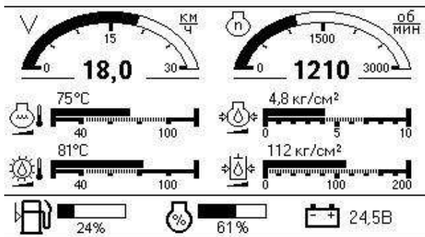
Рисунок И.4 – Экран транспортного режима
