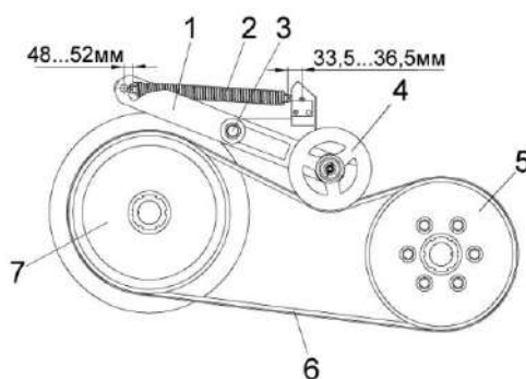
Рисунок 2.34 – Привод отбойного бitera
