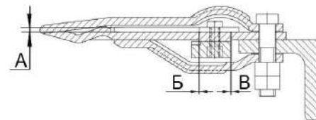
Рисунок 2.43 – Режущий аппарат
