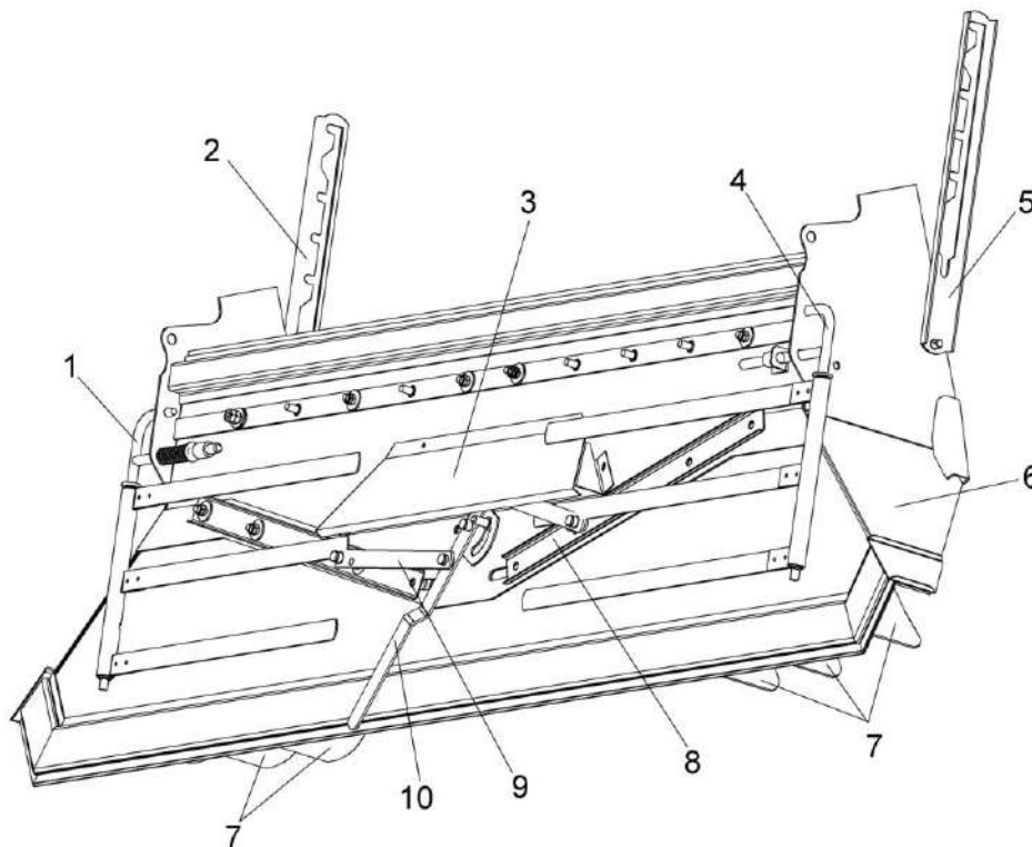
Рисунок 2.18 – Установка дефлектора
