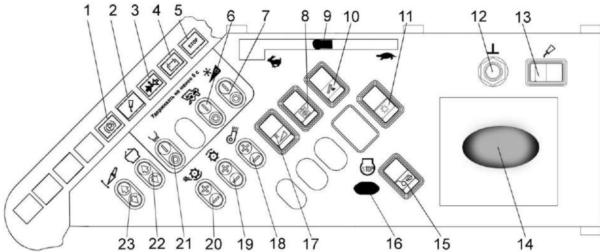
Рисунок 1.30 – Пульт управления комбайна с двигателем ЯМЗ
