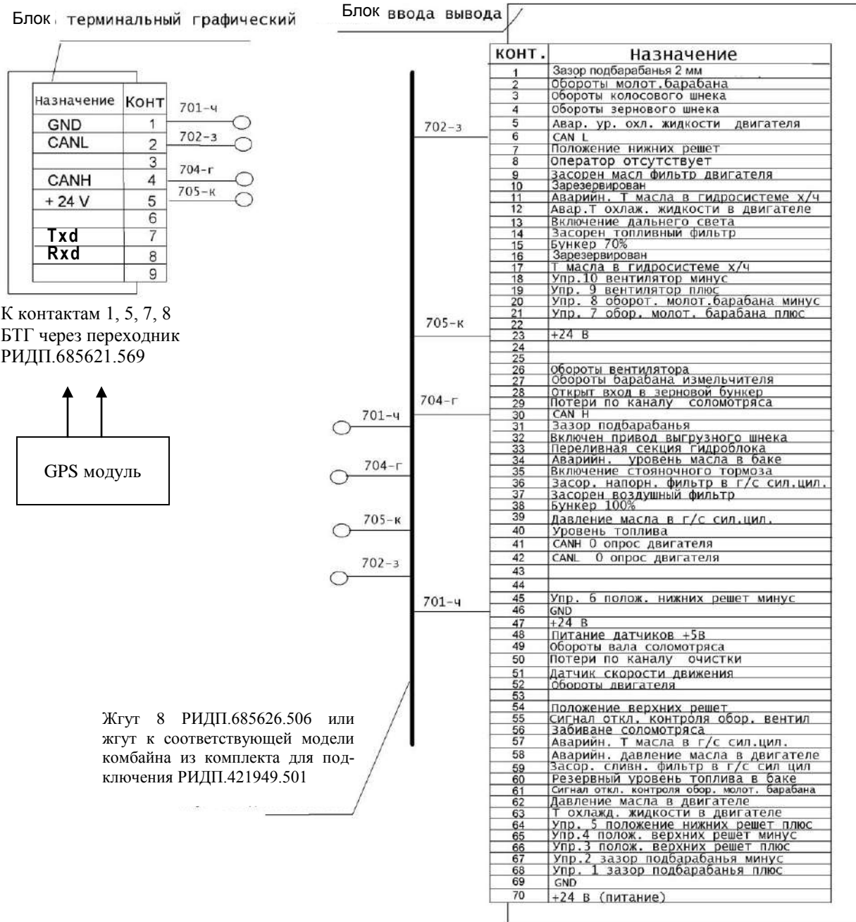
Рисунок К.38 – Схема подключения БТГ, БВВ и GPS модуля комбайна
