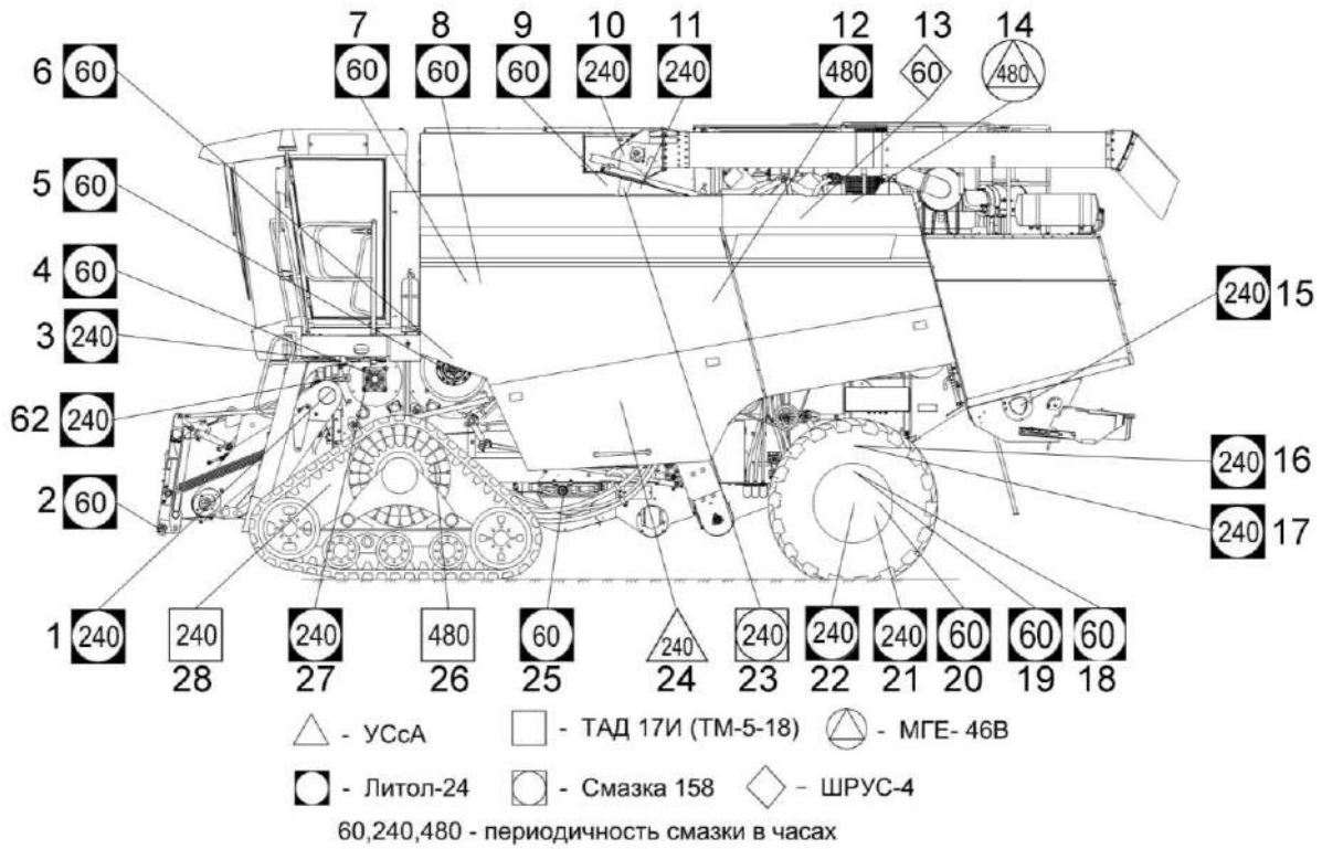
Рисунок 3.2 – Смазка молотилки (вид слева)
