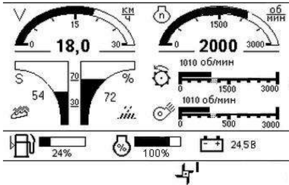
Рисунок И.3 – Экран технологического режима уборки (комбайнирования)
