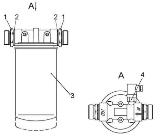
1 – штуцер; 2 – прокладки; 3 – фильтр; 4 – электронный датчик фильтроэлемента
