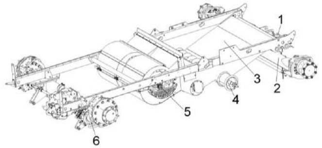
1 – устройство прицепное; 2 – мост управляемых ведущих колес; 3 – стан решетчатый нижний; 4 – блок шнеков; 5 – вентилятор; 6 – мост ведущих колес
