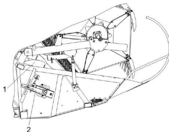
1 - шнек; 2 - рычаг Рисунок 1.5 – Жатка
