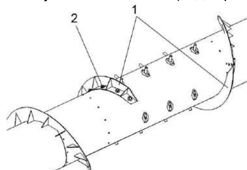
1 - витки; 2 – крепеж Рисунок 2.40 – Расположение витков
