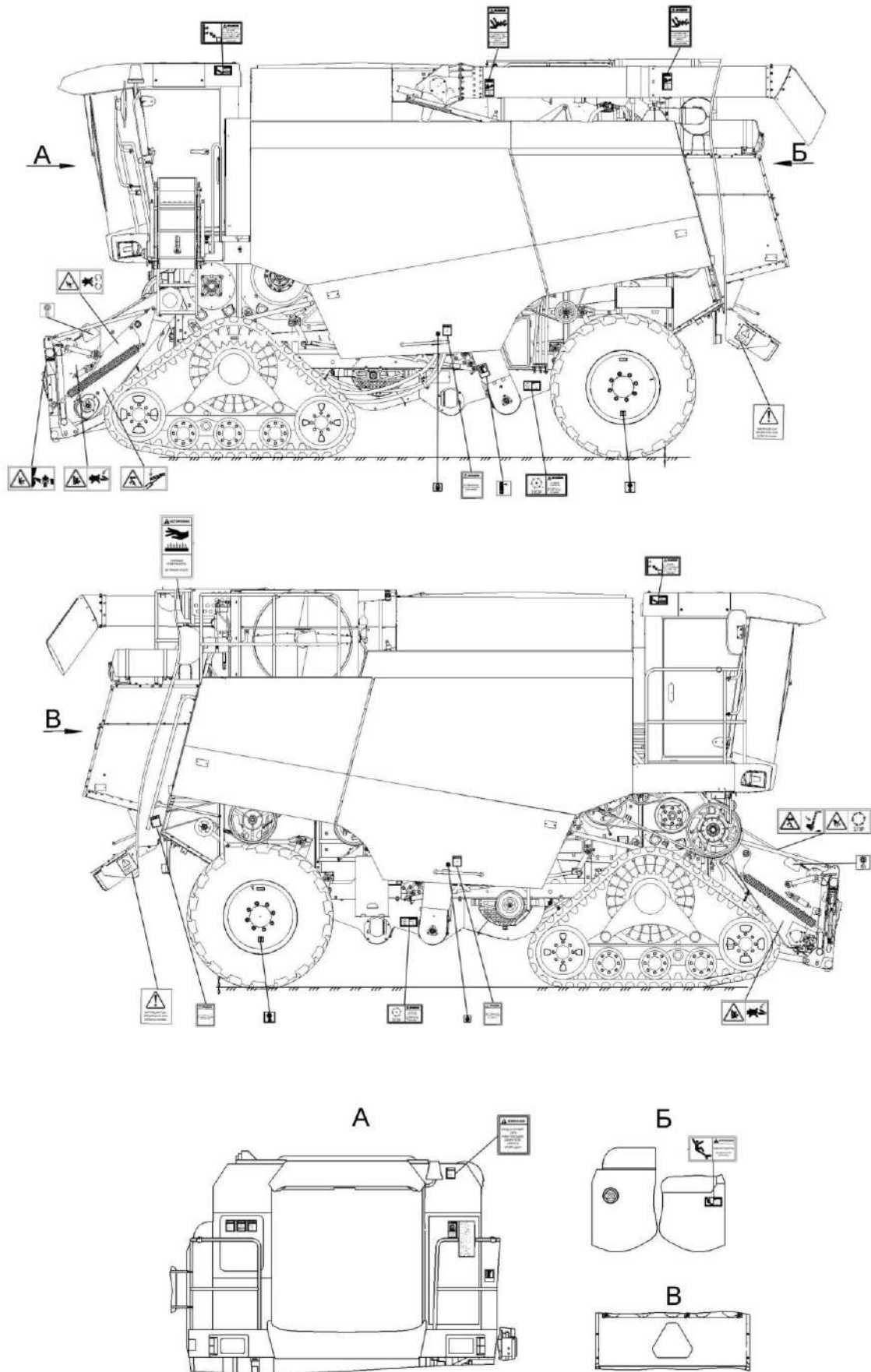
Молотилка самоходная
