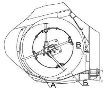
А – зазор между витками шнека и днищем жатки; Б – зазор между пальцами шнека и днищем жатки В – зазор между витками шнека и чистиками Рисунок 2.38 – Схема расположения шнека и его пальчикового механизма при работе жатки
