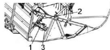
1 – рычаг; 2 – тяга; 3 – опоры шнека Рисунок 2.39 – Жатка (вид справа)
