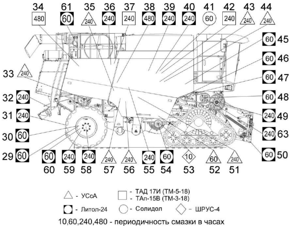
Рисунок 3.3 – Смазка молотилки (вид справа)
