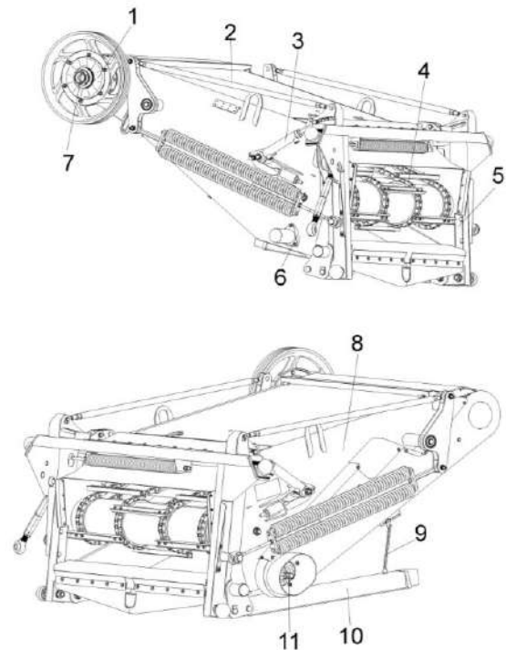
1 – муфта предохранительная; 2 – механизм продольного копирования; 3 - гидравлическая система; 4 - транспортер; 5 - рамка переходная; 6 - реверс; 7 – вал верхний; 8 – корпус; 9 - цепочка; 10 – упор; 11 – вал трансмиссионный
