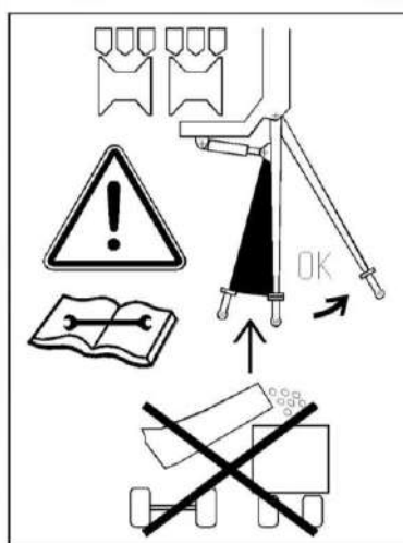
Рисунок 7.3 – Порядок выгрузки бункера
