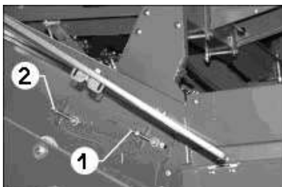
1, 2 - винты
