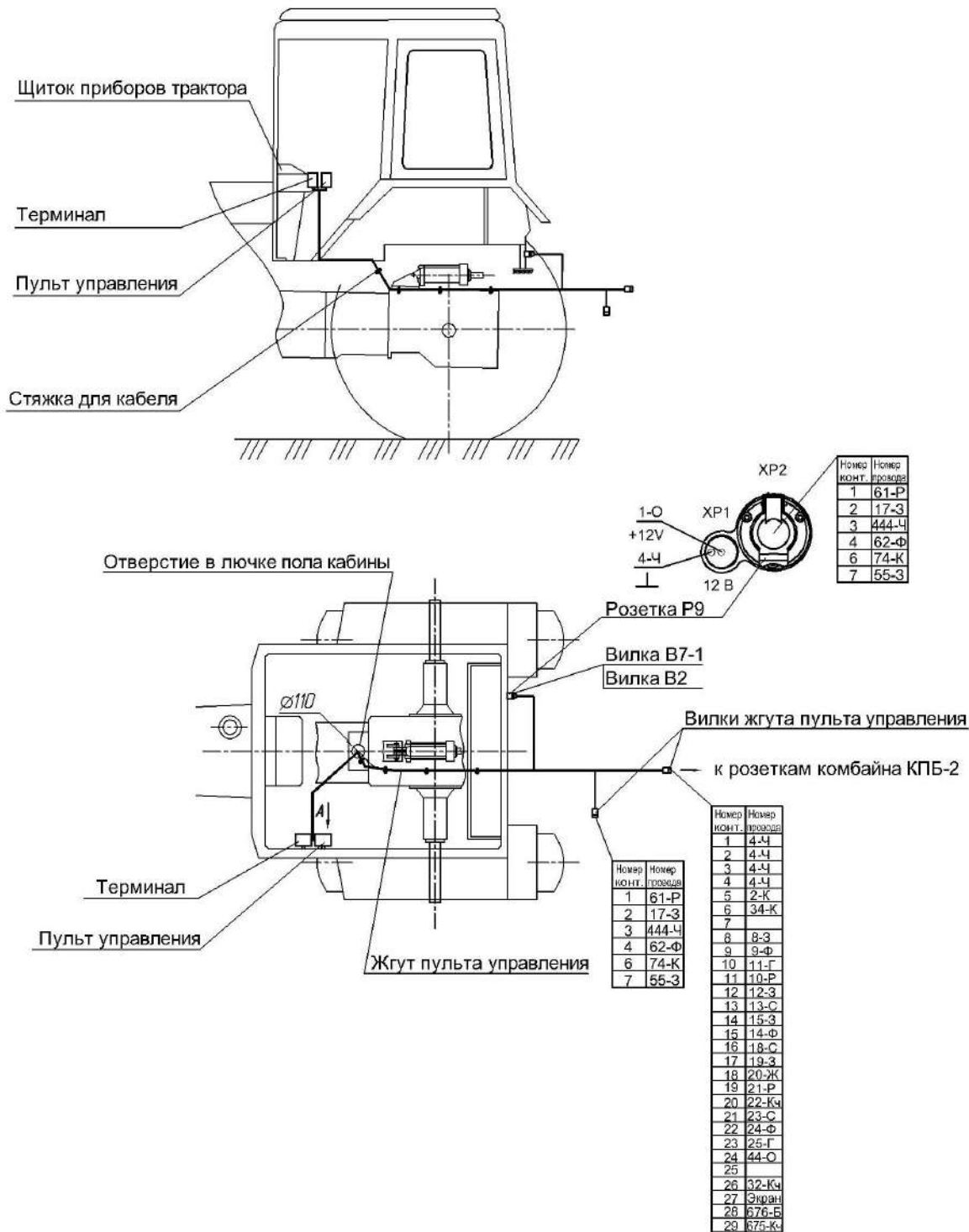
Рисунок 5.1 – Схема подключения электрооборудования комбайна в кабине трактора
