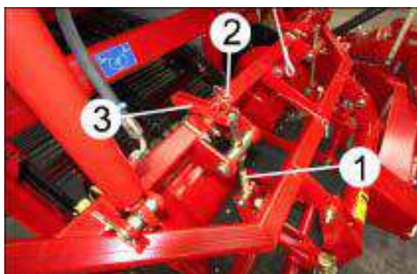
1 – шпильки; 2 – шплинт; 3 – рычаг
