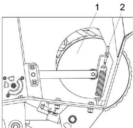
Рисунок 7.11 - Регулировка усилия прижатия ботвозатягивающих колес
