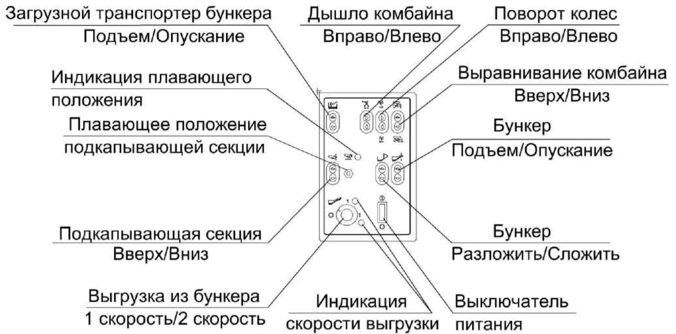
Рисунок 5.2 – Пульт управления
