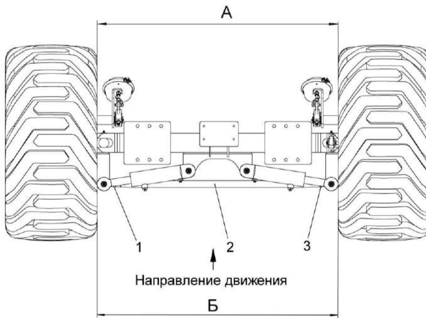
1, 3 – гайки; 2 – тяга рулевая
