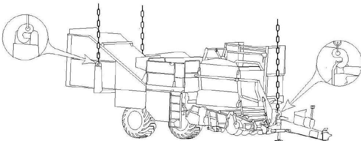
Рисунок 14.2 - Схема строповки комбайна
