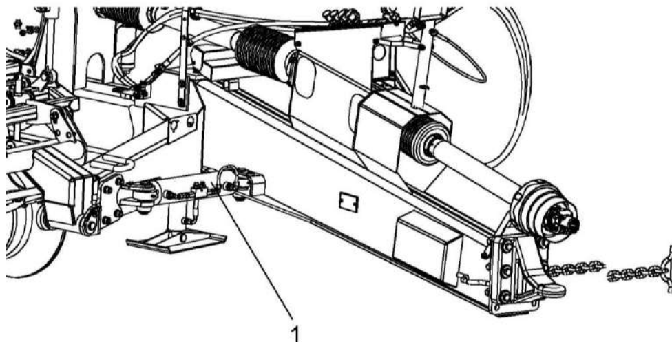
1 – дышло
