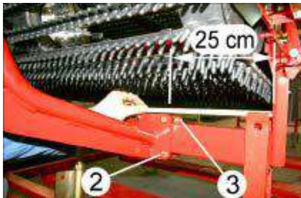
2 – болты; 3 – прижимная пластина
