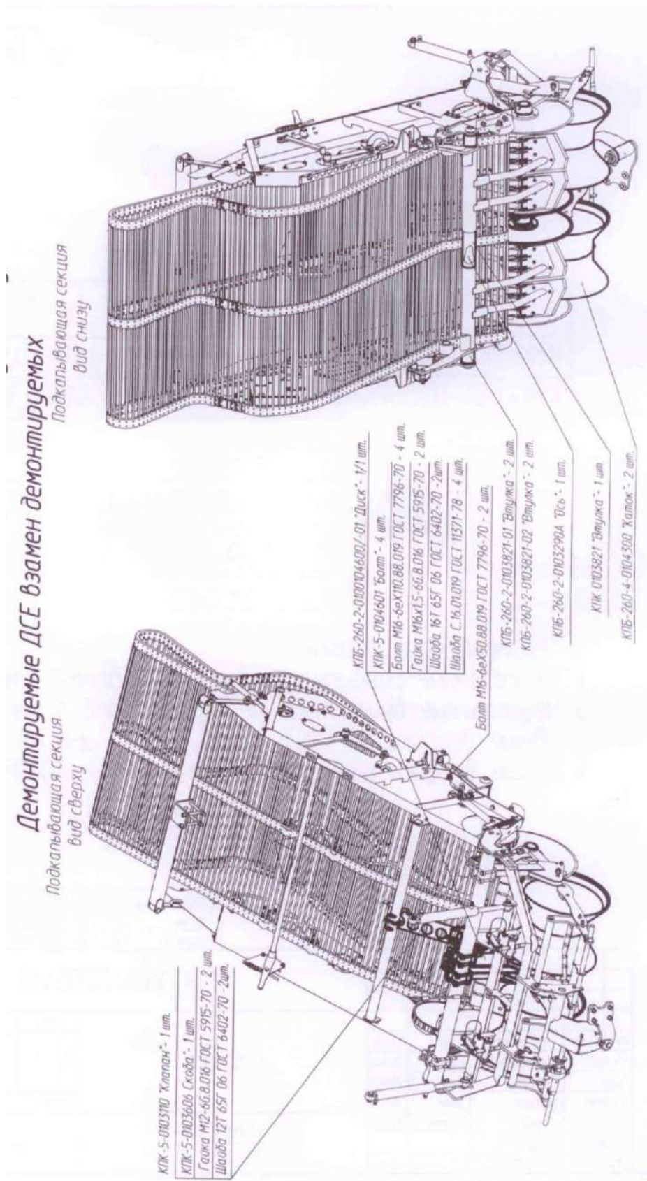
Рисунок 6.7 – Комплект балки с центральным лемехом КПБ-260-20001440 и сменными катками КПБ-260-20014700 (поставляется по отдельному заказу за отдельную плату)
