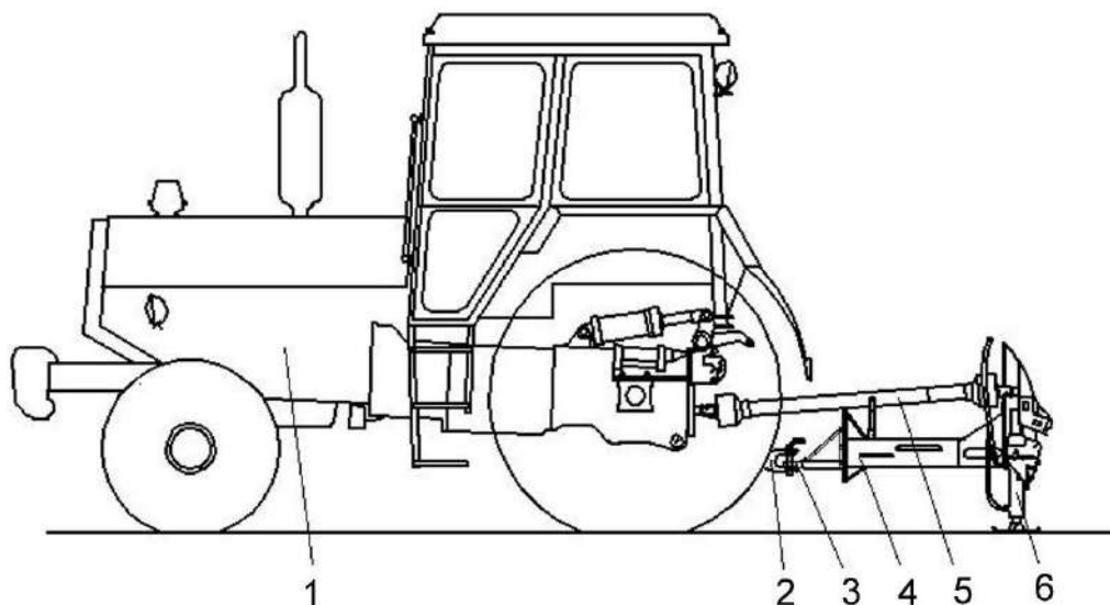
1 – трактор; 2 - вилка ТСУ-2В-01; 3 – сцепная петля; 4 – дышло; 5 – карданный вал; 6 – стояночная опора
