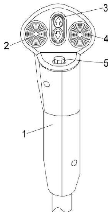
1 – рукоятка управления скоростью движения; 2 – кнопка управления жаткой; 3 – резерв; 4 – кнопка управления мотовилом; 5 – кнопка звукового сигнала
