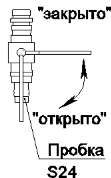
Рисунок 3.4 – Сливной кран
