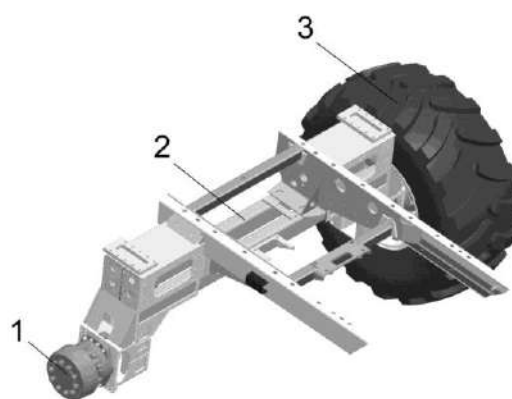
Рисунок 1.13 – Шасси
