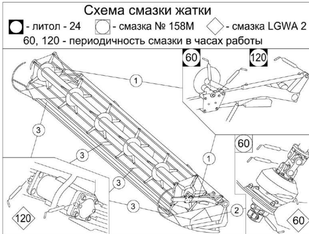
Рисунок 3.3 – Схема смазки жатки
