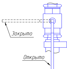
Рисунок 1 – Кран всасывающего фильтра
