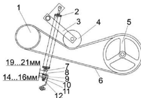
Рисунок 2.32 – Привод гидронасоса
