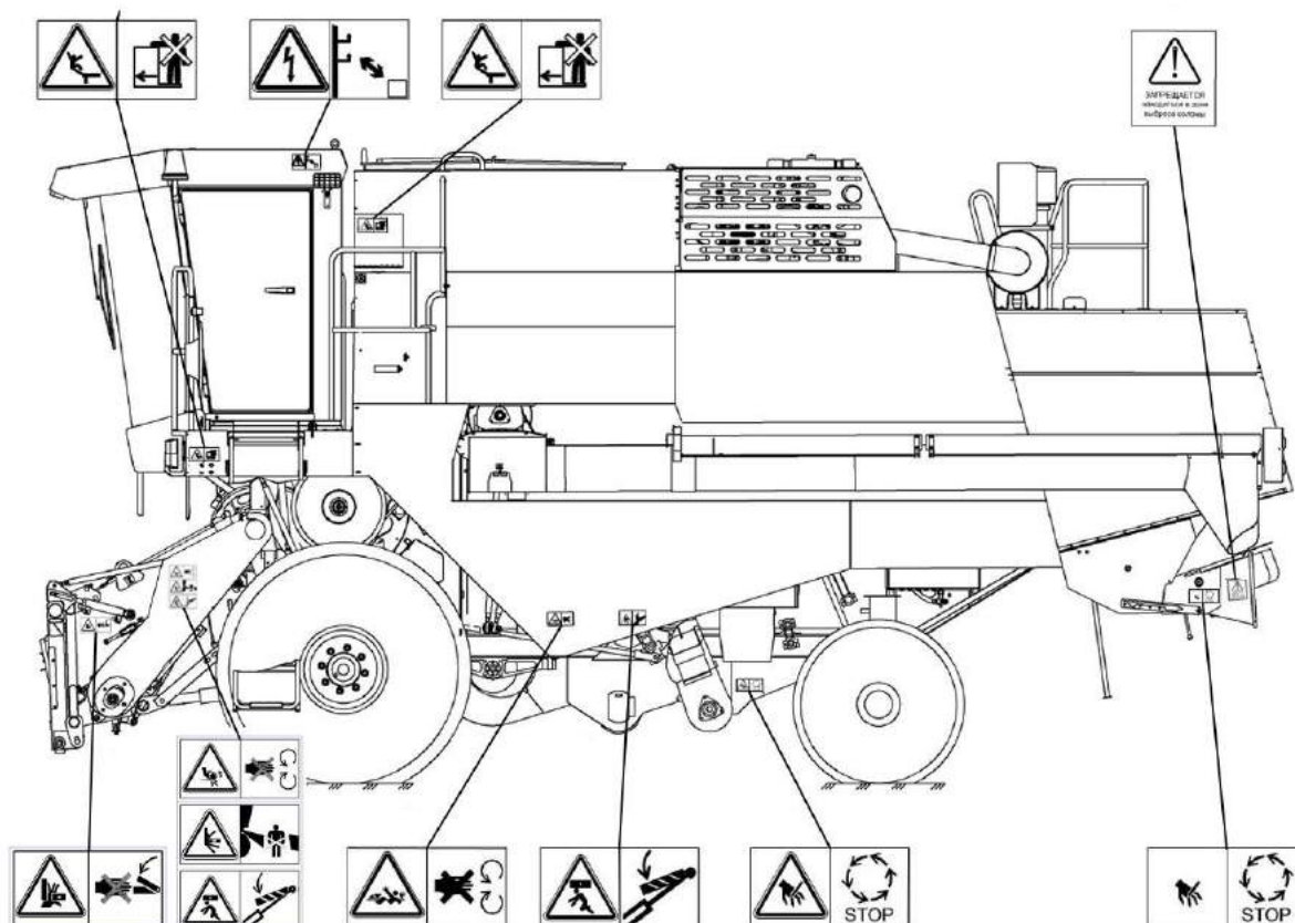
Молотилка самоходная (вид слева)
