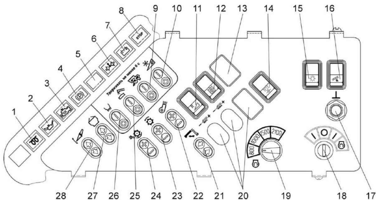
Рисунок 1.35 – Пульт управления
