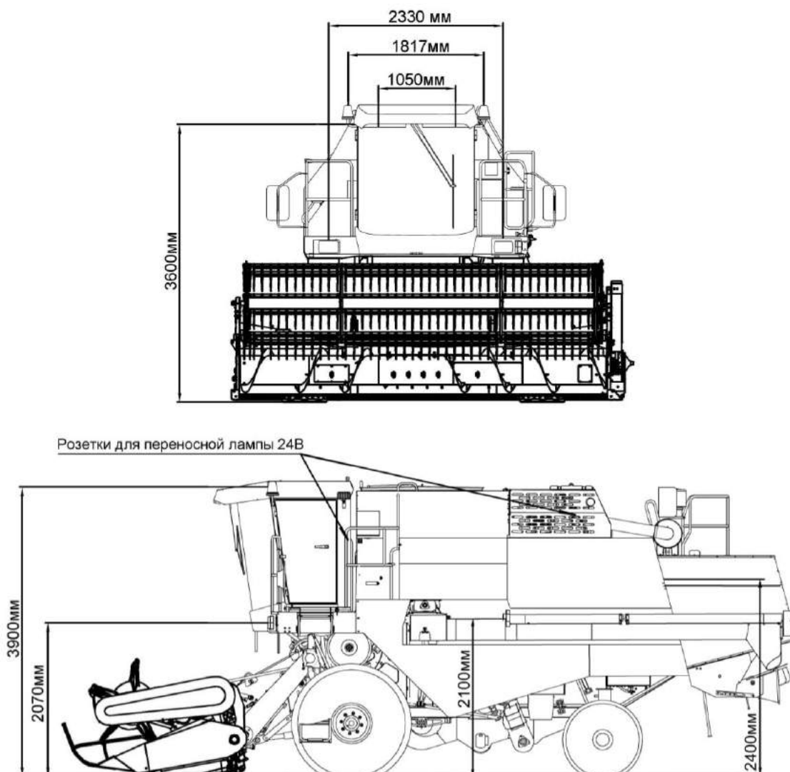
Рисунок 1.32 – Расположение наружного освещения и световой сигнализации комбайна
