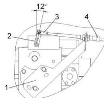
1 – кронштейн; 2 – флажок гидронасоса; 3 – ось; 4 – трос
