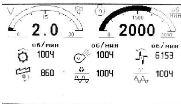
Рисунок 1.95 – Экран оборотов рабочих органов
