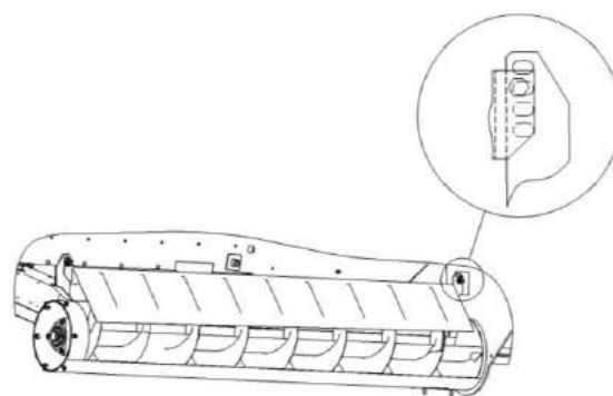
Рисунок 2.18 – Регулировка ограждения над горизонтальным шнеком бункера
