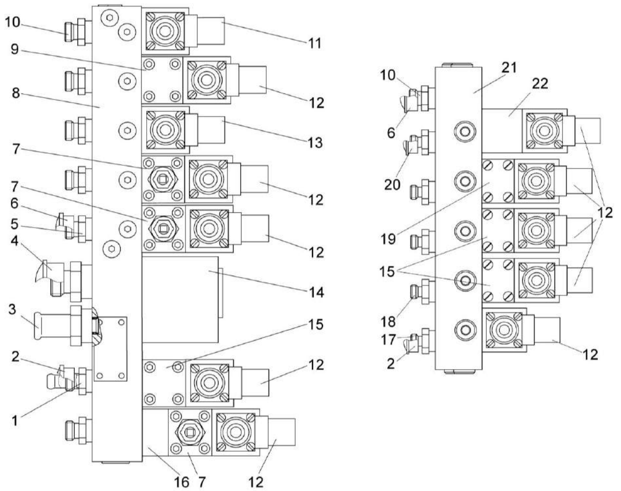
1, 5, 10, 17, 18 – штуцера; 2, 6, 20 – заглушки; 3 – ниппель; 4, – крышки; 7, 22 – клапана редукционные; 8, 21 – плиты; 9, 15, 19 – гидрозамки; 11, 12, 13 – гидрораспределители; 14 – клапан предохранительный; 16 – гидродроссель с обратным клапаном
