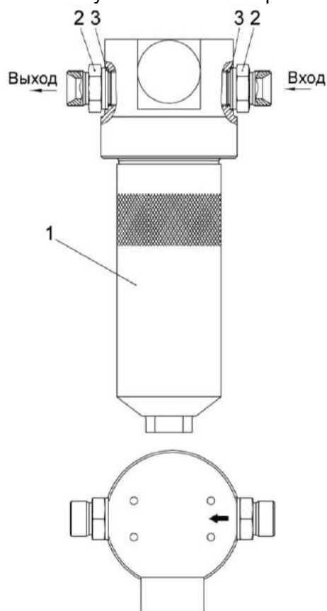
Рисунок 1.26 – Фильтр
