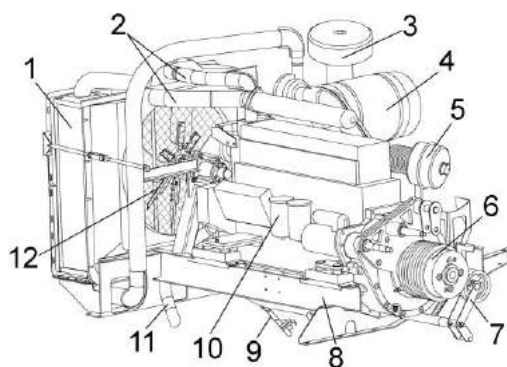
1 – блок радиаторов; 2 - трубы воздушные; 3 – воздухозаборник вращающийся; 4 – воздухозаборник; 5 - глушитель; 6 – главный привод; 7 - привод гидронасоса; 8 - рамка подмоторная; 9 - маслопровод сливной; 10 - двигатель; 11 – труба водяная; 12 – вентилятор
