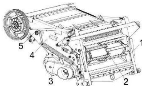
Рисунок 1.7 - Молотилка самоходная
