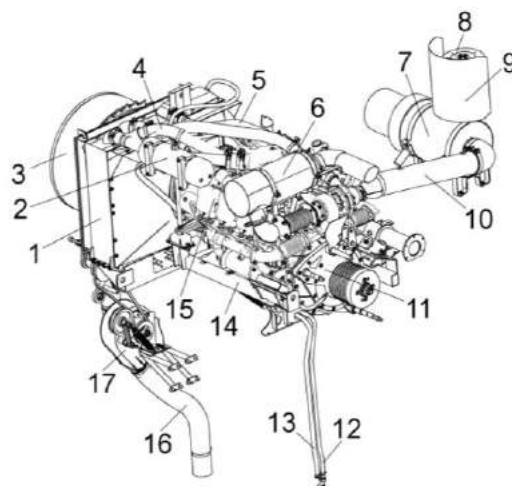
1 – блок радиаторов; 2 – бачок расширительный; 3 – воздухозаборник; 4, 10, 16 - трубы воздушные; 5 – труба водяная; 6 - глушитель; 7 – воздухоочиститель; 8 – воздухозаборник вращающийся; 9 – экран; 11 – главный привод; 12 – сливной рукав охлаждающей жидкости; 13 – сливной рукав масла; 14 - рама подмоторная; 15 - двигатель; 17 – вентилятор
