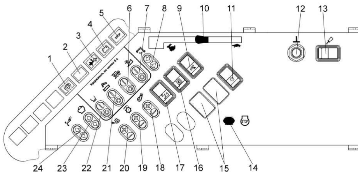
Рисунок 1.36 – Пульт управления
