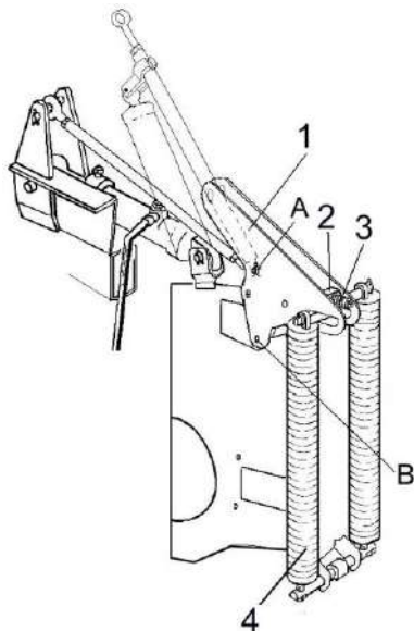
1 – рычаг механизма вывешивания; 2 – серьга; 3 – регулировочный болт; 4 – пружина
