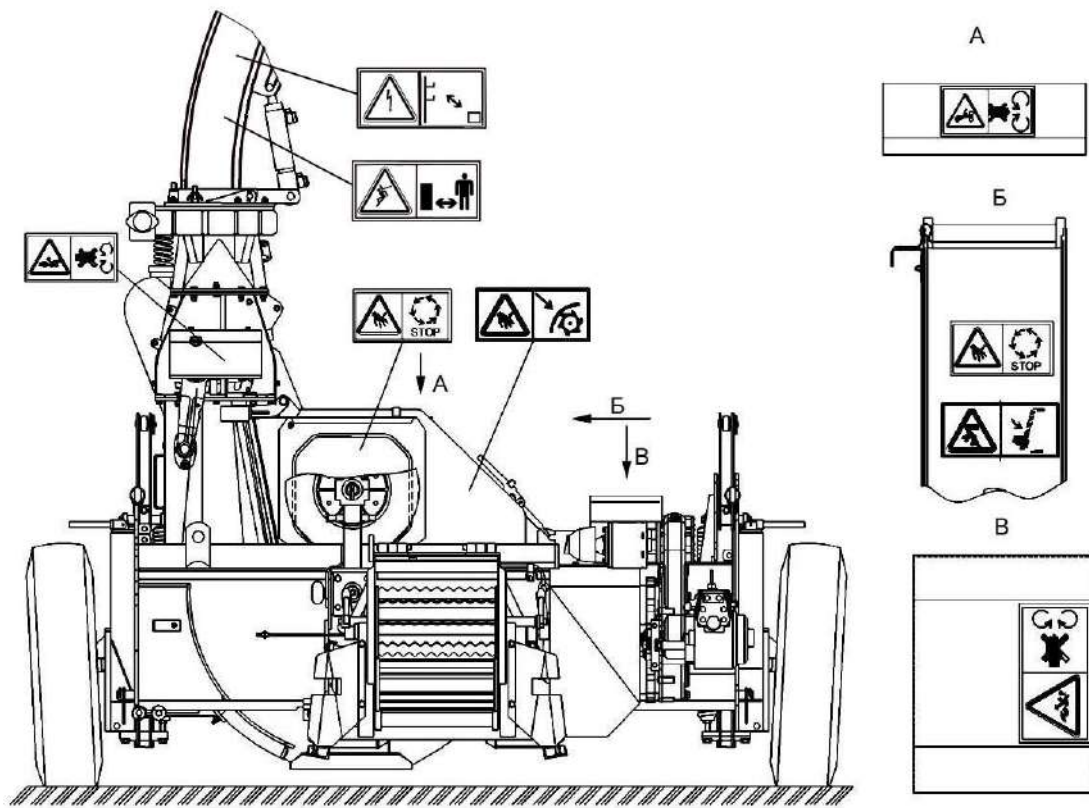
Измельчитель (вид спереди)
