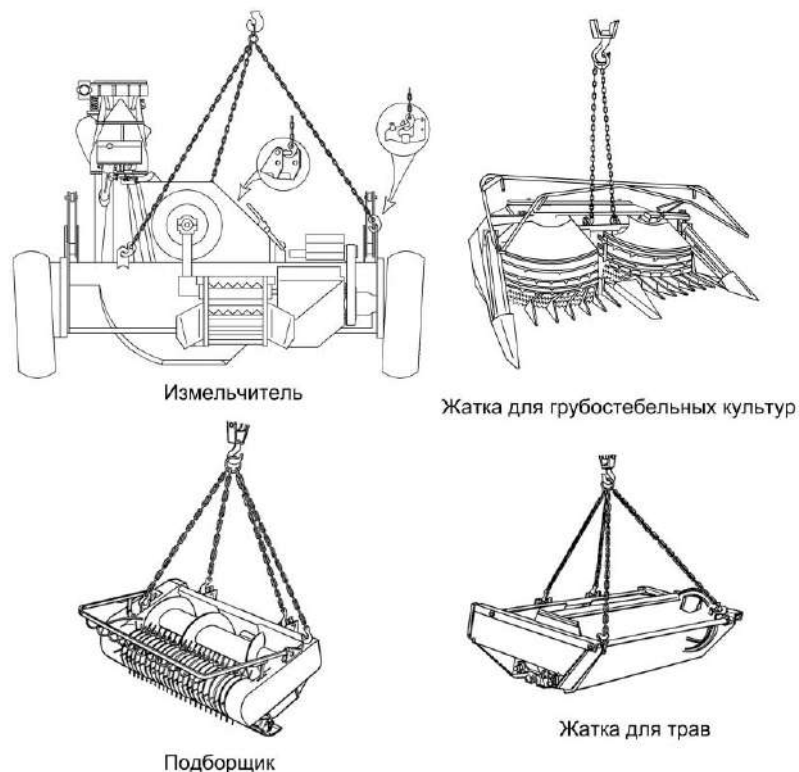
Рисунок 6.1 – Схемы строповок
