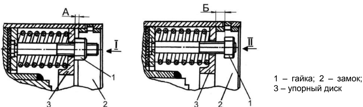
Рисунок 2.8 – Предохранительная муфта вала привода адаптеров
