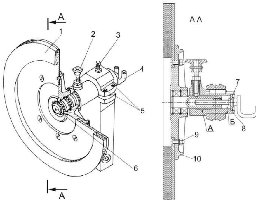
1 – заточной диск; 2 – стопор; 3 – фиксатор; 4 – винт; 5 – болты; 6 – шток; 7 – кольцо; 8 – корпус; 9 – гайка; 10 – диск
