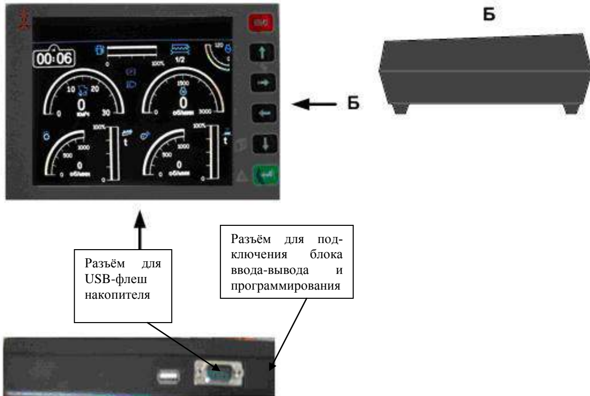
Рисунок 1.35 – Внешний вид лицевой панели БТГ
