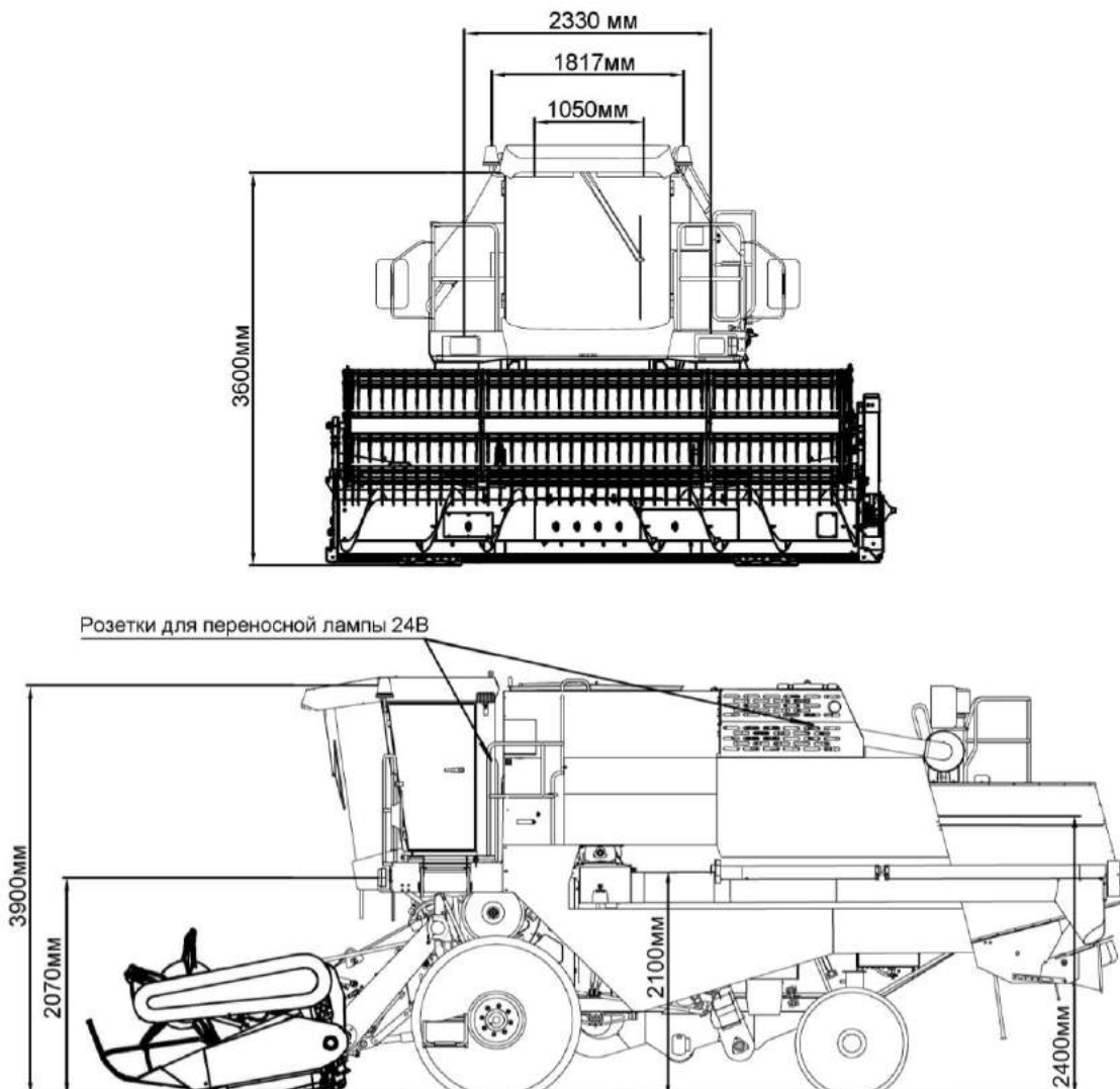
Рисунок 1.25 – Расположение наружного освещения и световой сигнализации комбайна
