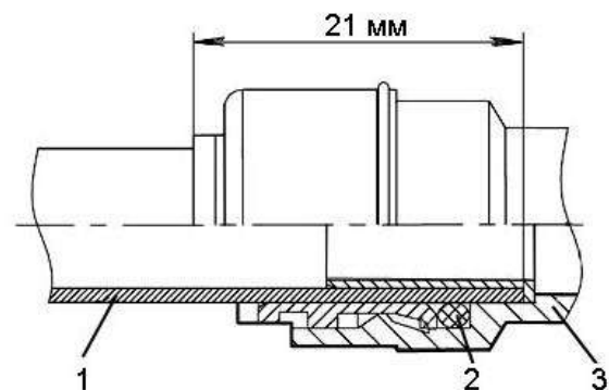
Рисунок 3.4 – Ресивер
