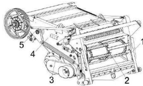
Рисунок 1.2 - Молотилка самоходная
