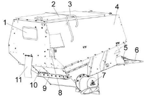
1 – смотровое окно; 2 – крыша бункера; 3 – поручень; 4 – проставка; 5 - вибропобудитель; 6 – настил; 7 – шнек горизонтальный; 8 – окно пробоотборника; 9 – балка; 10 – крышка; 11 - фартук
