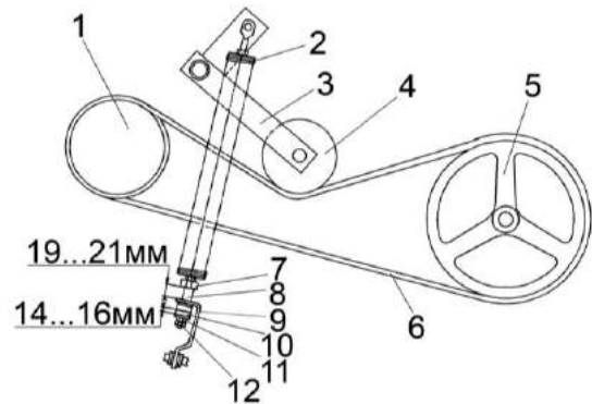
Рисунок 2.23 – Привод гидронасоса
