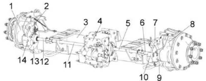
Рисунок 1.10 – Мост управляемых колес.
