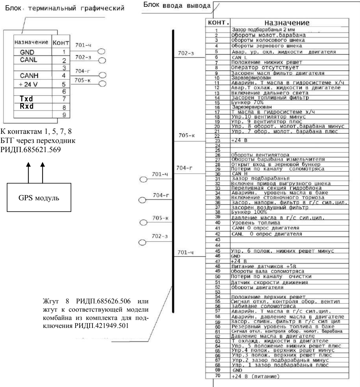
Рисунок 1.72 – Схема подключения БТГ, БВВ и GPS модуля комбайна
