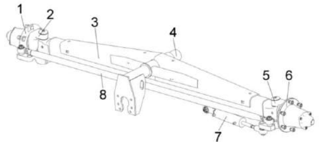
Рисунок 1.9 – Шасси
