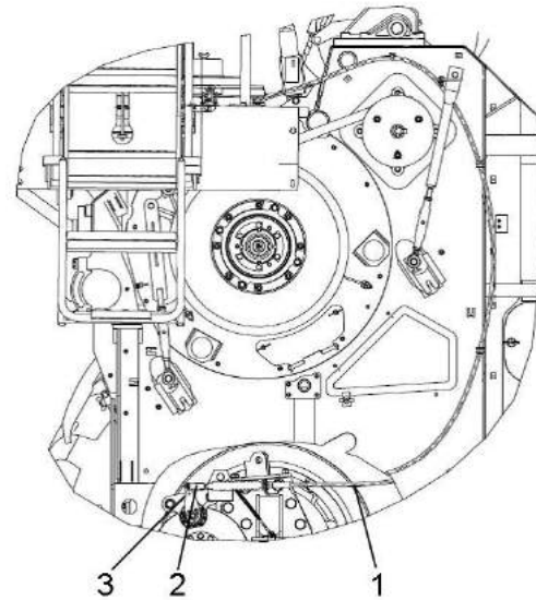
1 – трос; 2 – вилка; 3 - рычаг
