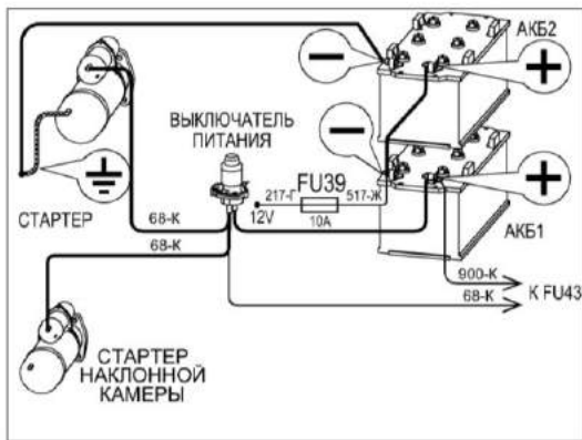
Рисунок 2.2 - Подключение аккумуляторных батарей
