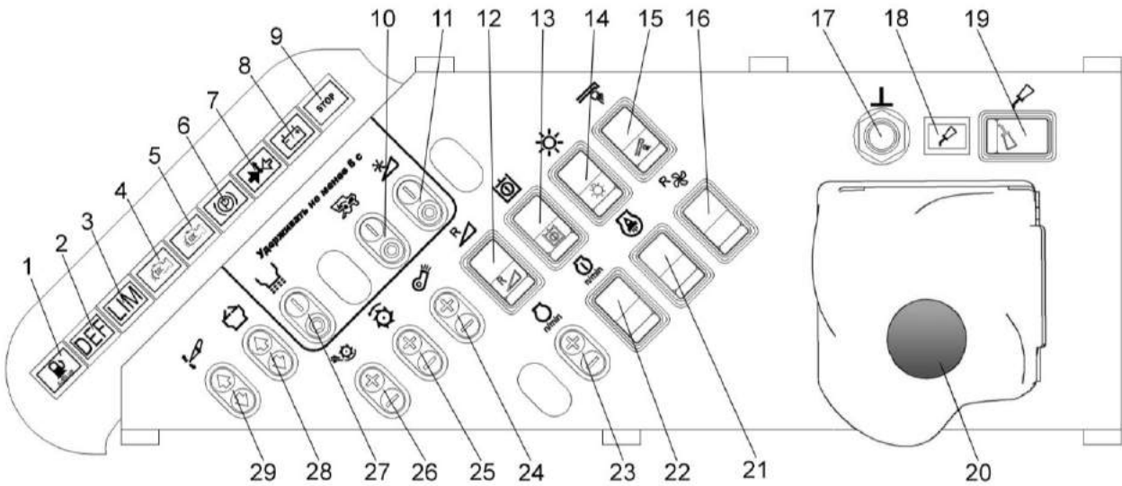
Рисунок 1.29 – Пульт управления комбайна
