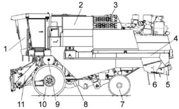
1 – кабина; 2 - бункер зерновой; 3 - установка двигателя; 4 – шнек выгрузной; 5 - дефлектор; 6 - соломоизмельчитель; 7 – мост управляемых колес; 8 - очистка; 9 - молотильный аппарат; 10 – мост ведущих колес; 11 – наклонная камера
