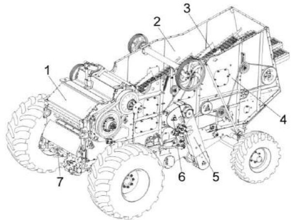
1 – аппарат молотильный; 2 – боковина правая; 3 – соломотряс; 4 – боковина левая; 5 – элеватор колосовой; 6 – устройство домолачивающее; 7 – шасси
