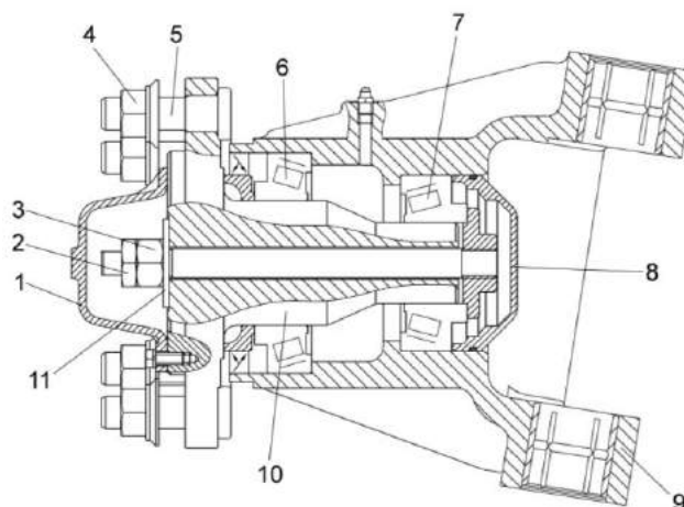
1, 8 – крышки; 2 – контргайка; 3, 4 – гайки; 5 - болт специальный; 6, 7 – подшипники; 9 – поворотный кулак; 10 - ось; 11 - шайба
