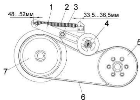
Рисунок 2.36 – Привод отбойного бitera
