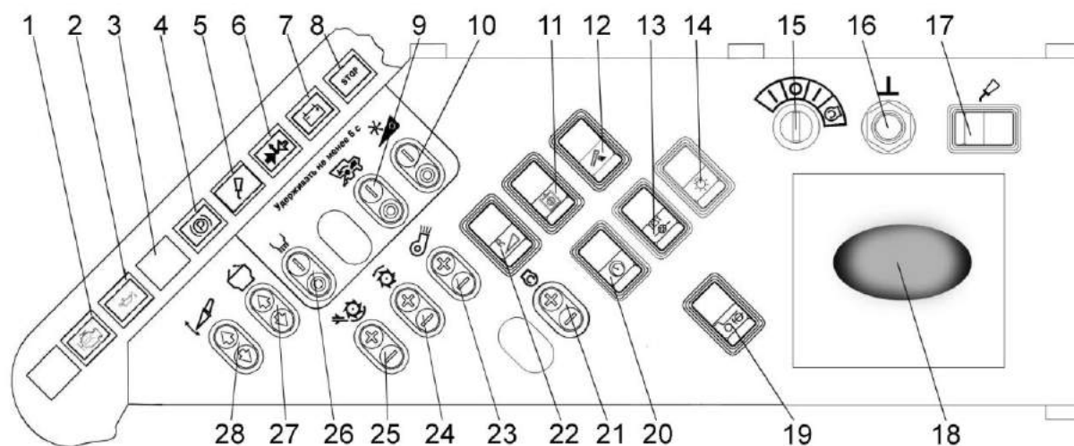
Рисунок 1.35 – Пульт управления комбайна с двигателем DTA
