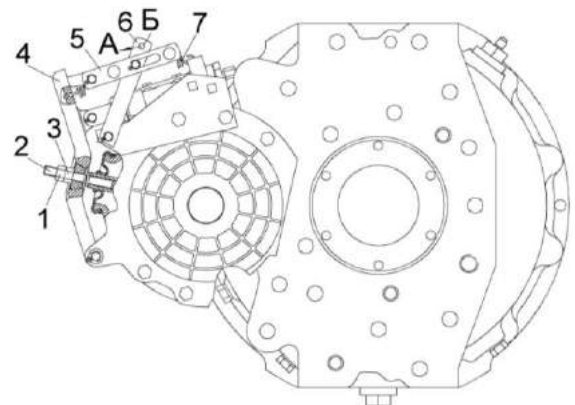
Рисунок 2.26 - Регулировка сходимости колес
