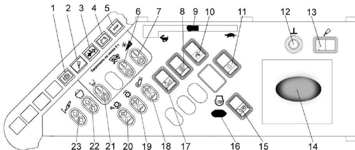
Рисунок 1.34 – Пульт управления комбайна с двигателем ЯМЗ
