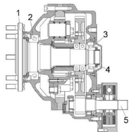
Рисунок 2.27 - Редуктор бортовой
