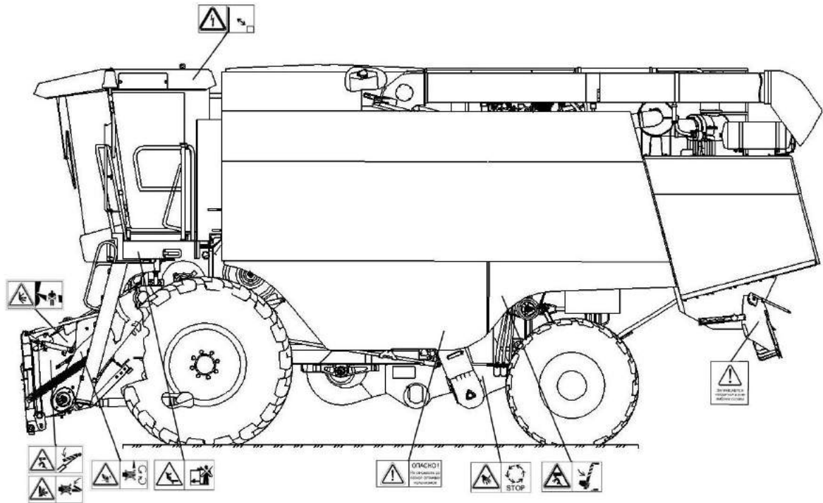
Молотилка самоходная (вид слева)
