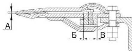
Рисунок 2.44 – Режущий аппарат
