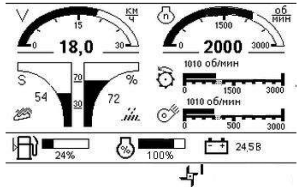
Рисунок 1.93 – Экран технологического режима уборки (комбайнирования)
