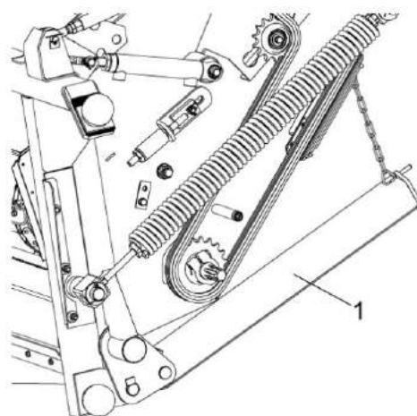
Рисунок 2.13 – Наклонная камера
