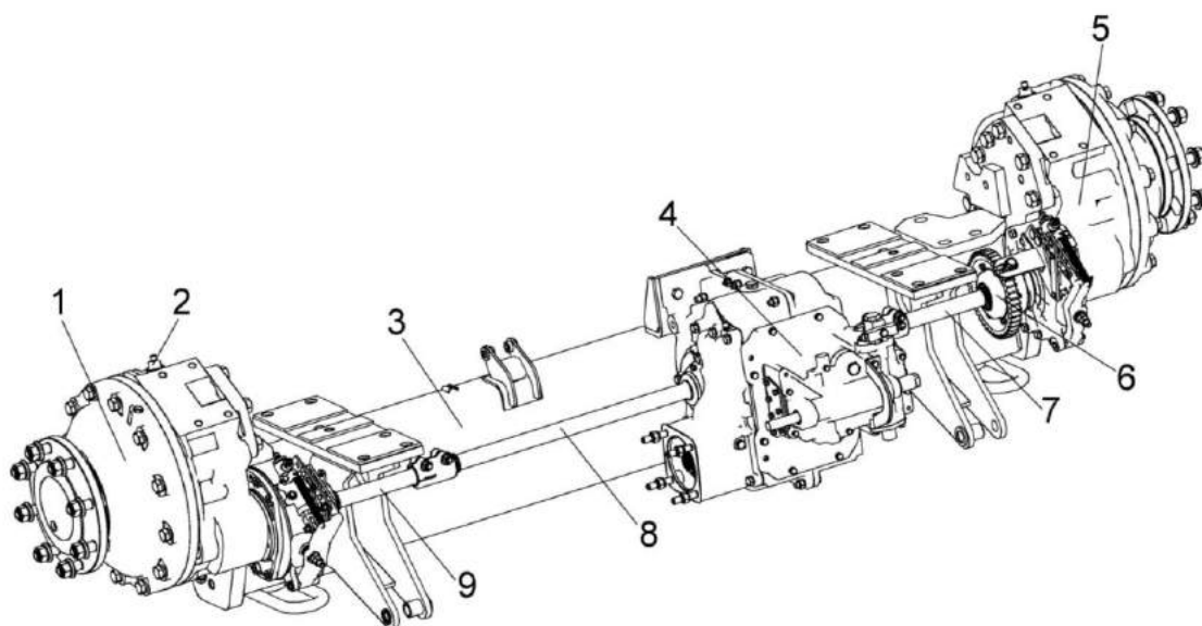
Мост ведущих колес
