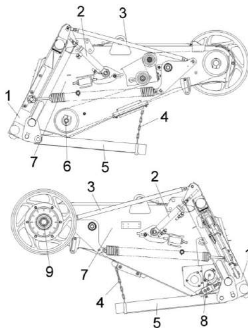
1 – рамка переходная; 2 – цепочно-планчатый транспортер; 3 – механизм реверса; 4 - рама; 5 – механизм продольного копирования; 6 - цепочка; 7 – упор; 8 – вал
