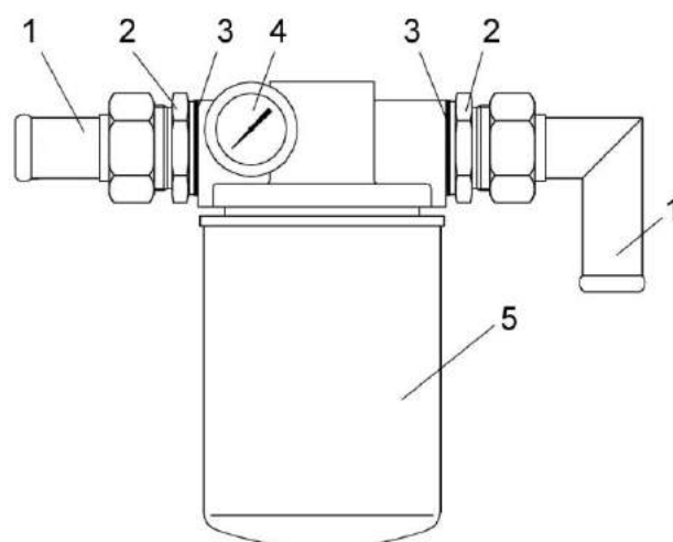
1 – хомут стяжной; 2 – штуцера; 3 – прокладки; 4 – вакуумметр; 5 – фильтр
