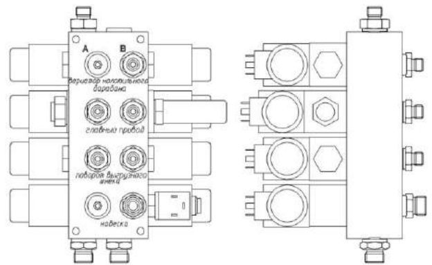
Рисунок 1.21 – Гидроблок четырехсекционный
