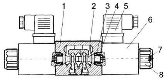
1 – корпус; 2 – золотник; 3 – толкатель; 4 – пружина; 5 – штепсельный разъем; 6 – катушка электромагнита; 7 – аварийная (контрольная) кнопка; 8 – гайка А, В – цилиндрические отводы; Р – подвод рабочей жидкости; Т – слив рабочей жидкости
