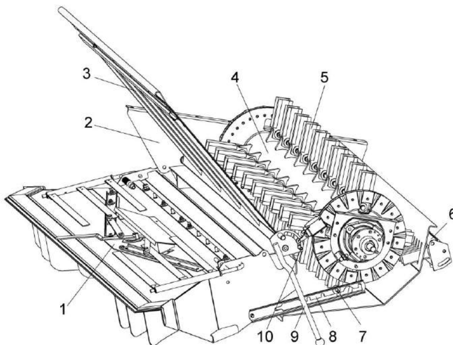
1 – дефлектор; 2 – корпус измельчителя; 3 – заслонка; 4 – ротор измельчителя; 5 – нож; 6 – ножевая опора; 7, 10 – гайки; 8 – ползоз; 9 - рукоятка сектора
