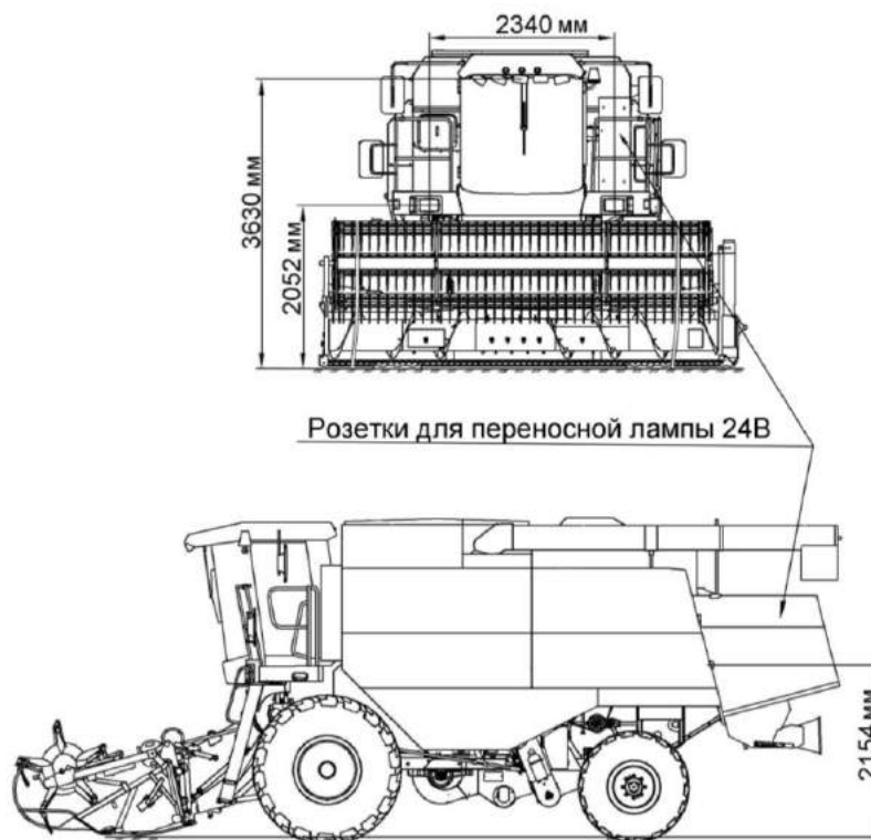
Рисунок 1.30 – Расположение наружного освещения и световой сигнализации комбайна
