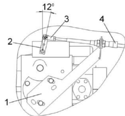
Рисунок 2.24 – Блок управления
