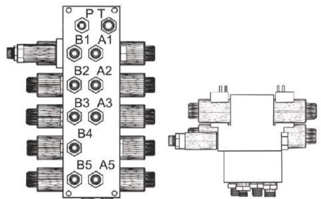
Рисунок 1.22 - Гидроблок пятисекционный
