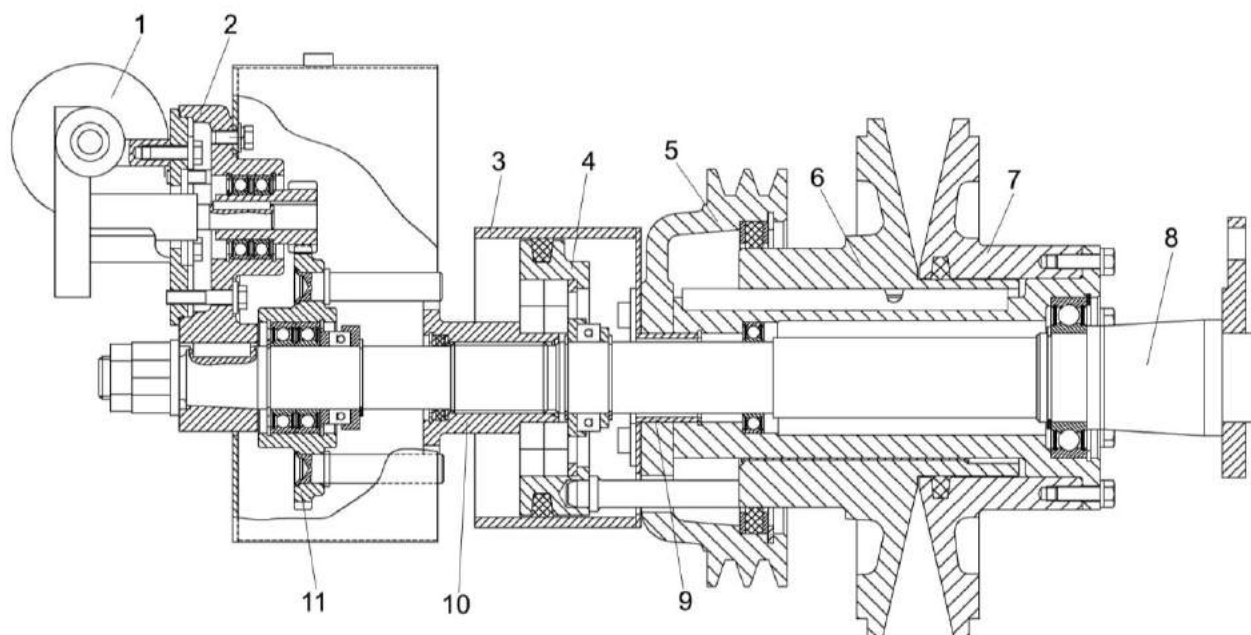
Рисунок 2.21 – Контрпривод вариатора
