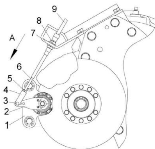
1 – стояночный тормоз; 2 – рычаг; 3 – ось; 4 – вилка; 5, 8 – гайки; 6 – шток; 7 – кронштейн; 9 – трос;
