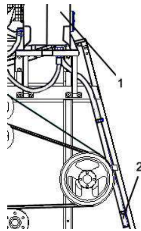
1 - маслобак; 2 - сливной рукав Рисунок 3.6
