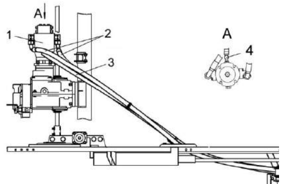
1 – гидромотор аксиально-поршневой нерегулируемый; 2 – рукава высокого давления; 3 - рукава; 4 – полумуфта заправочная
