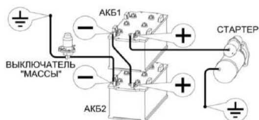
Рисунок 2.2 - Подключение аккумуляторных батарей
