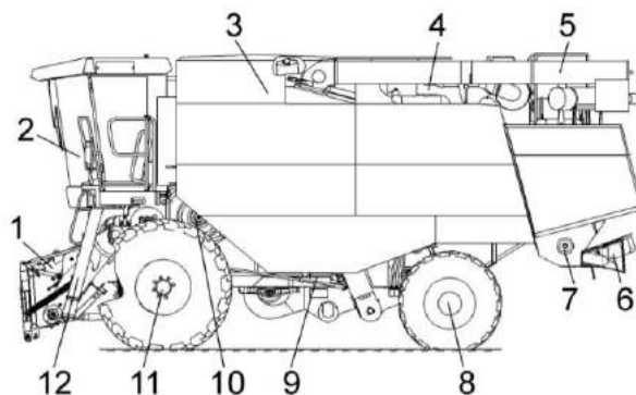
1 – наклонная камера; 2 - кабина; 3 – бункер зерновой; 4 - установка двигателя; 5 – шнек выгрузной; 6 - дефлектор; 7 - соломоизмельчитель; 8 – мост управляемых колес; 9 - очистка; 10 – молотильный аппарат; 11 – мост ведущих колес; 12 - трап
