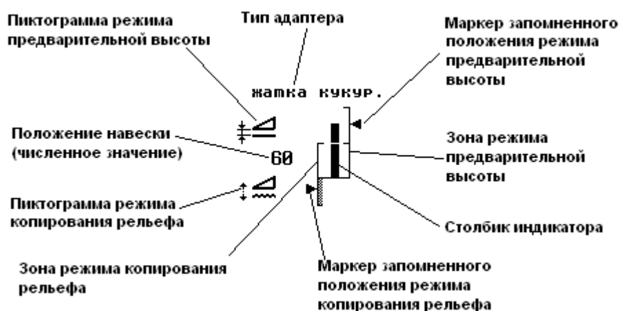
Рисунок Р.7 – Индикатор положения навески
