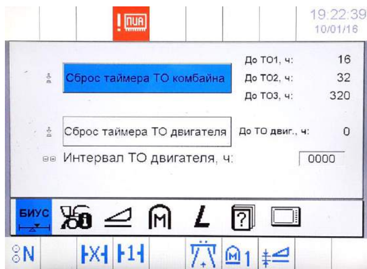
Рисунок Р.9 – Интервалы техобслуживания
