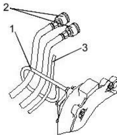
1 – держатель, 2 - разъемы гидросистемы, 3 – электрожгут
