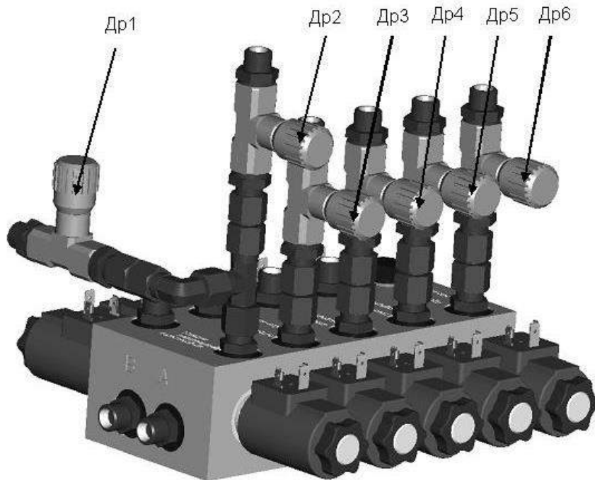
Рисунок 1.41 - Гидроблок пяти секционный ГБ2.2
