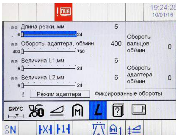
Рисунок Р.21 –Установка длин резок
