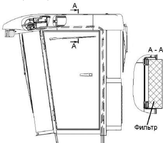
Рисунок 3.10 - Очистка кассетных фильтров кабины
