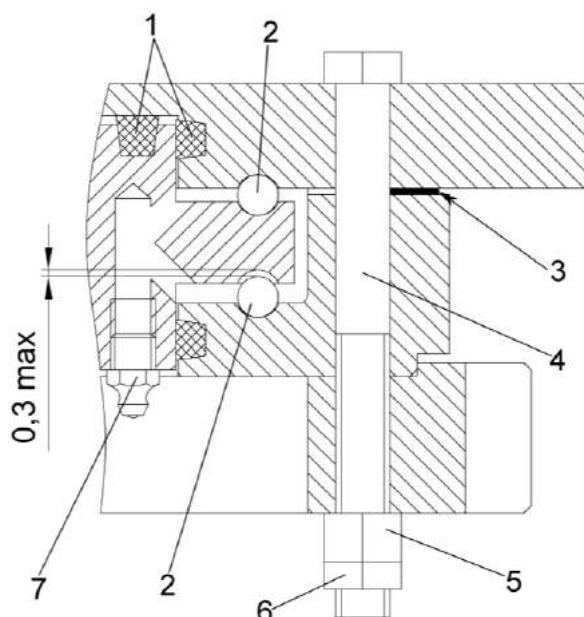
1 – уплотнения; 2 – шарики; 3 – прокладка регулировочная; 4 – болт; 5 – гайка; 6 – контргайка; 7 – масленка
