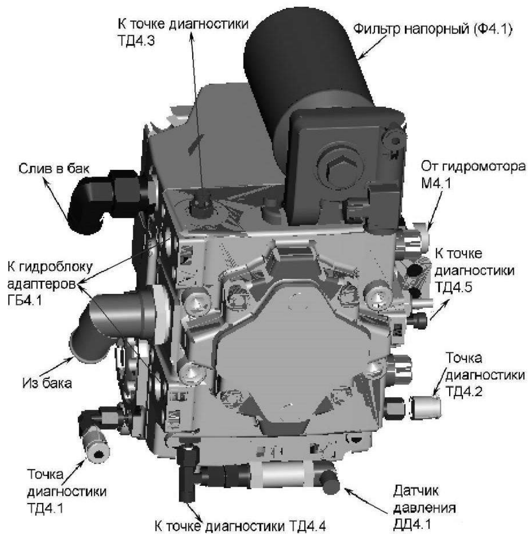
Рисунок 1.60 – Гидронасос привода адаптеров (Н4.1)
