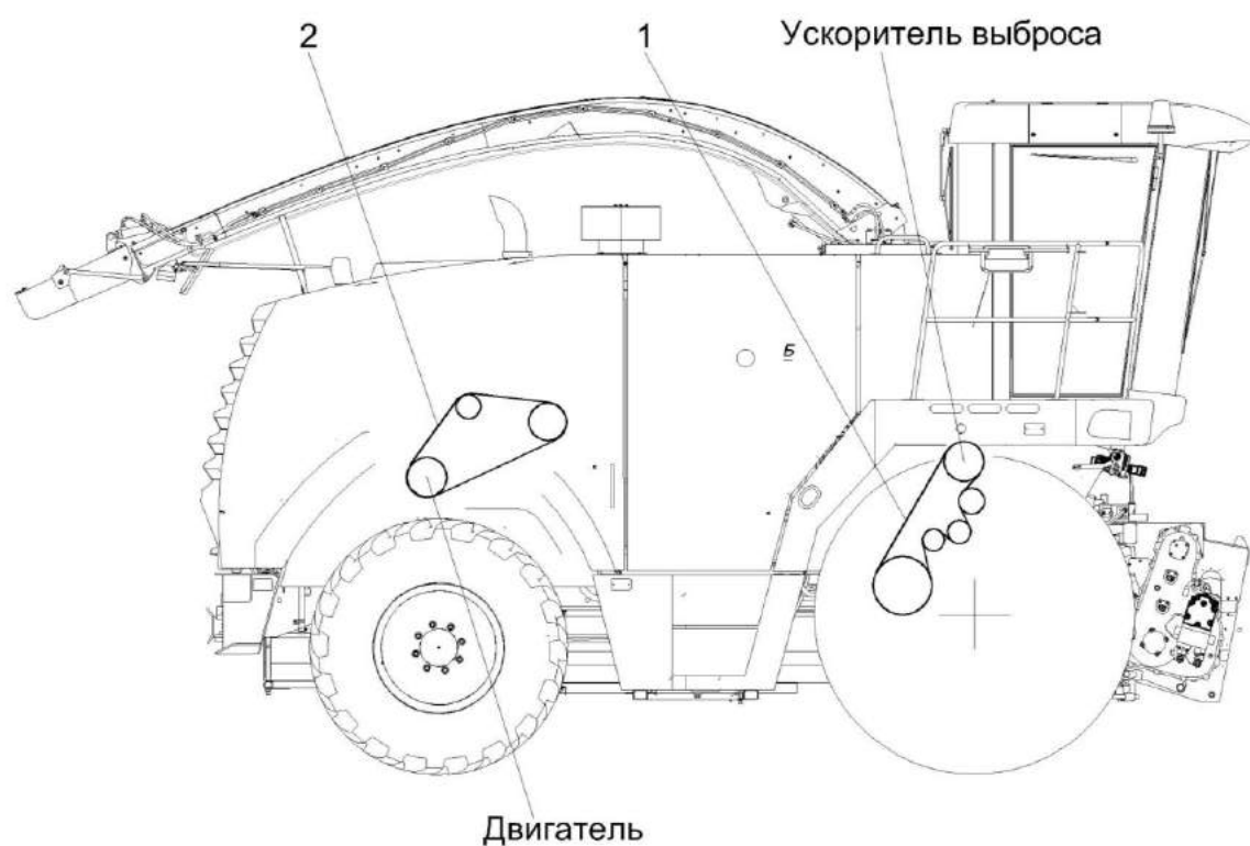
Рисунок Т.2 – Схема приводов измельчителя (вид справа)
