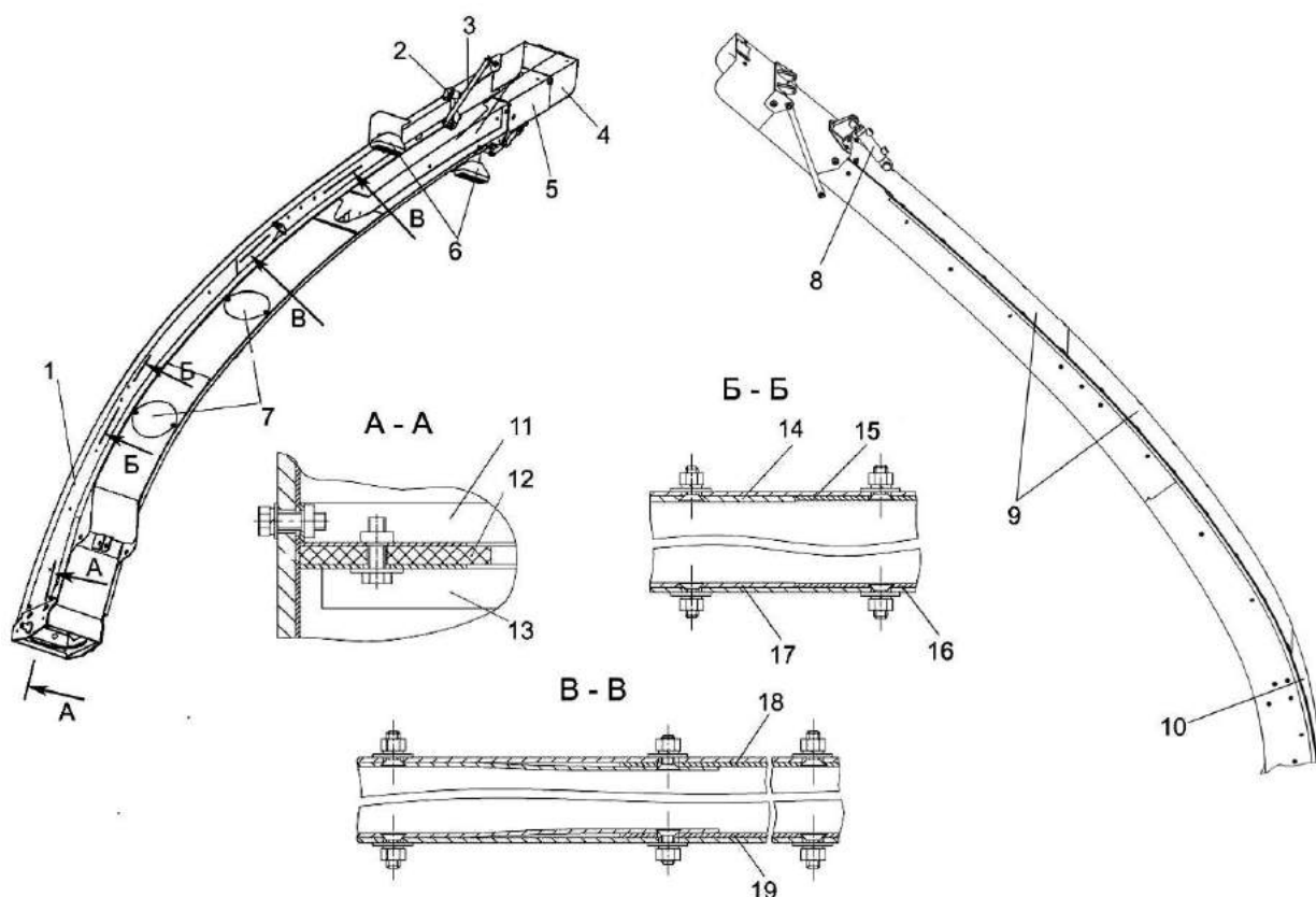
Рисунок 1.28 – Силосопровод с основанием силосопровода и механизмом поворота
