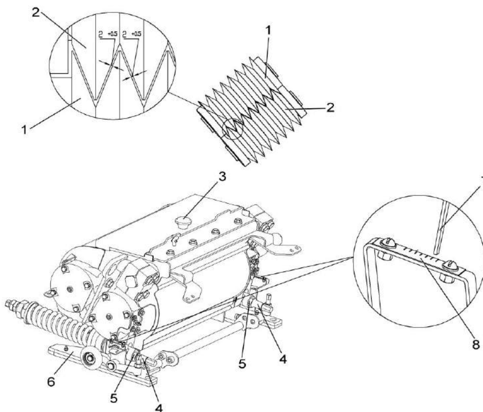
1 – валец задний, 2 – валец передний; 3 – ручка; 4 – тяга; 5 – гайка; 6 – корпус; 7 - указатель; 8 – шкала
