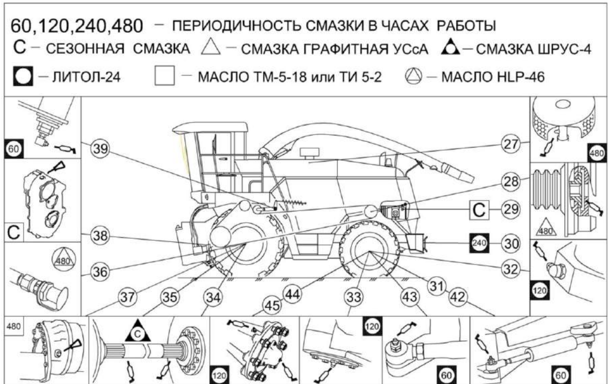
Рисунок 3.17 – Схема смазки измельчителя КВК 0100000-01 (вид слева)
