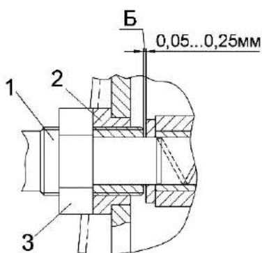
1, 2 – втулки; 3 – гайка
