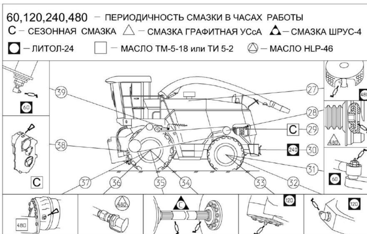
Рисунок 3.16 – Схема смазки измельчителя КВК 0100000 (вид слева)
