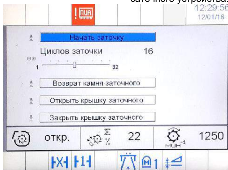
Рисунок Р.31 – Меню заточки ножей
