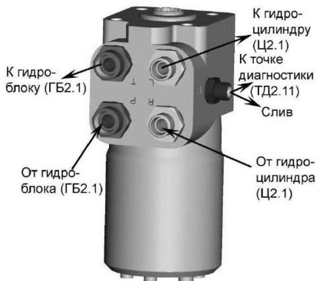
Рисунок 1.47 – Насос – дозатор (НД2.1)
