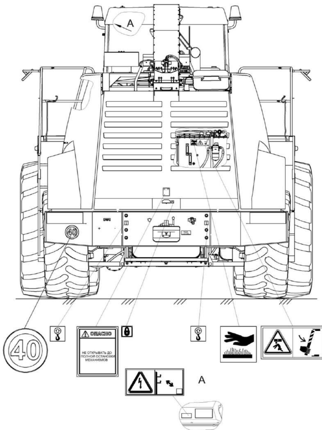
Знаки безопасности на измельчителе самоходном (вид сзади)
