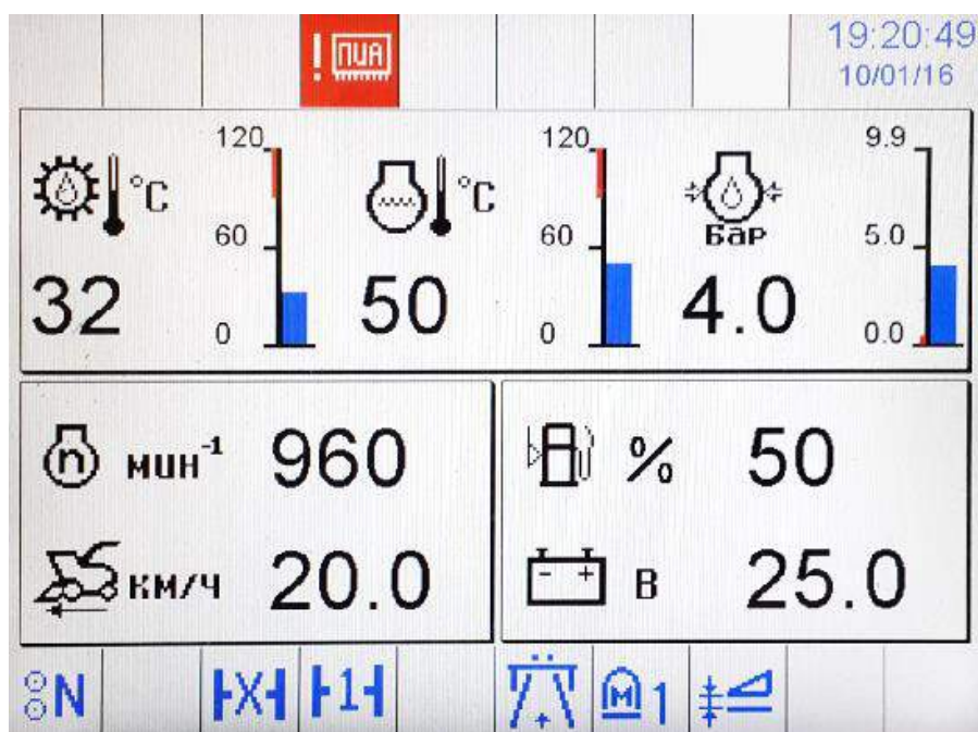
Рисунок Р.5 – Экран транспортирования
