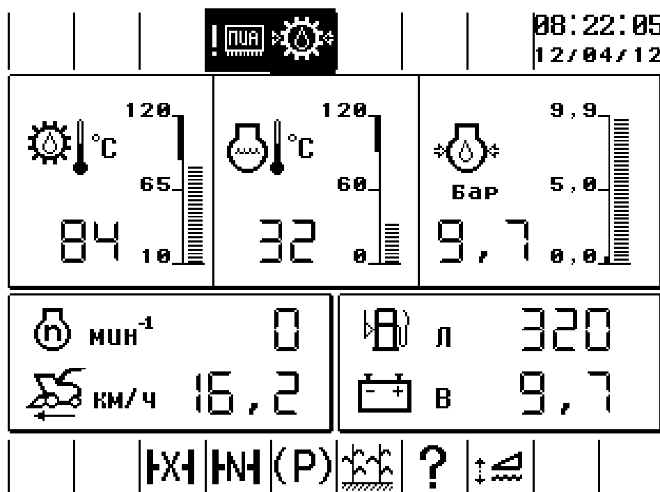
Рисунок Ж.5 – Экран транспортирования
