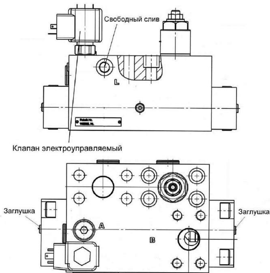
Рисунок 4.8 - Гидроблок экстренного останова
