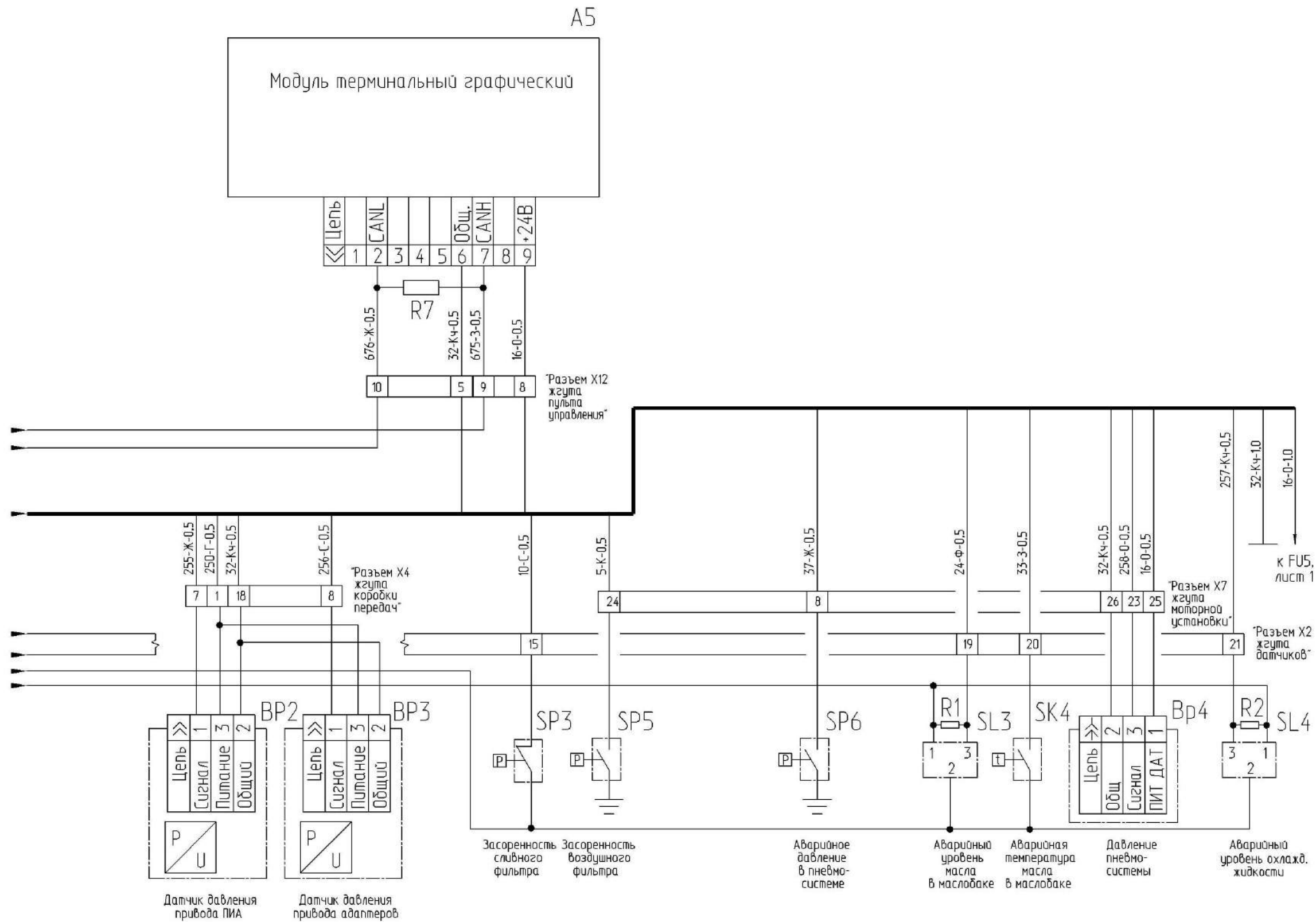
Рисунок В.5 - Схема электрическая принципиальная комплекса (лист 2)
