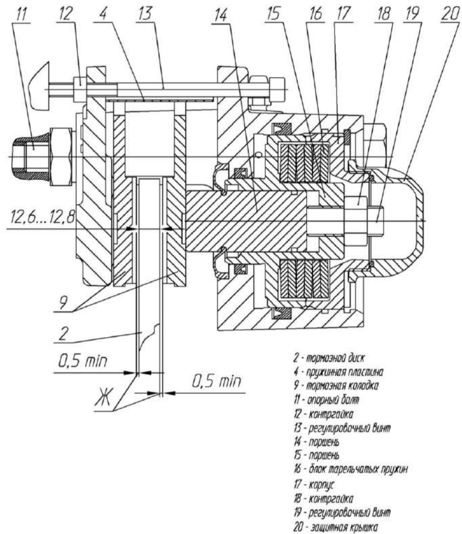
Рисунок С.5 – Монтаж тормоза на тормозном диске
