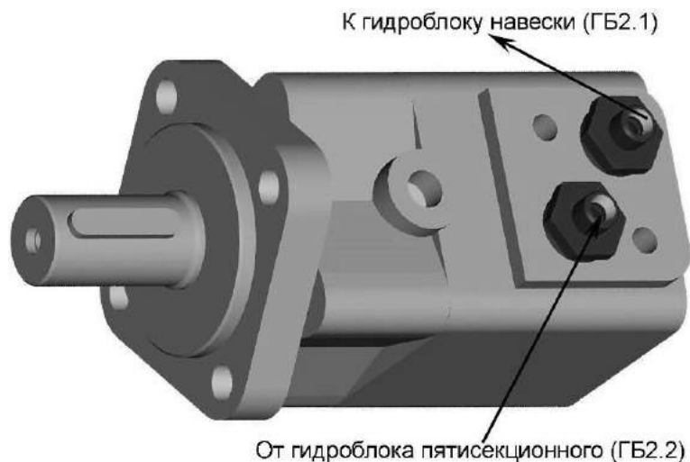
Рисунок 1.45 – Гидромотор заточного устройства (М2.2)
