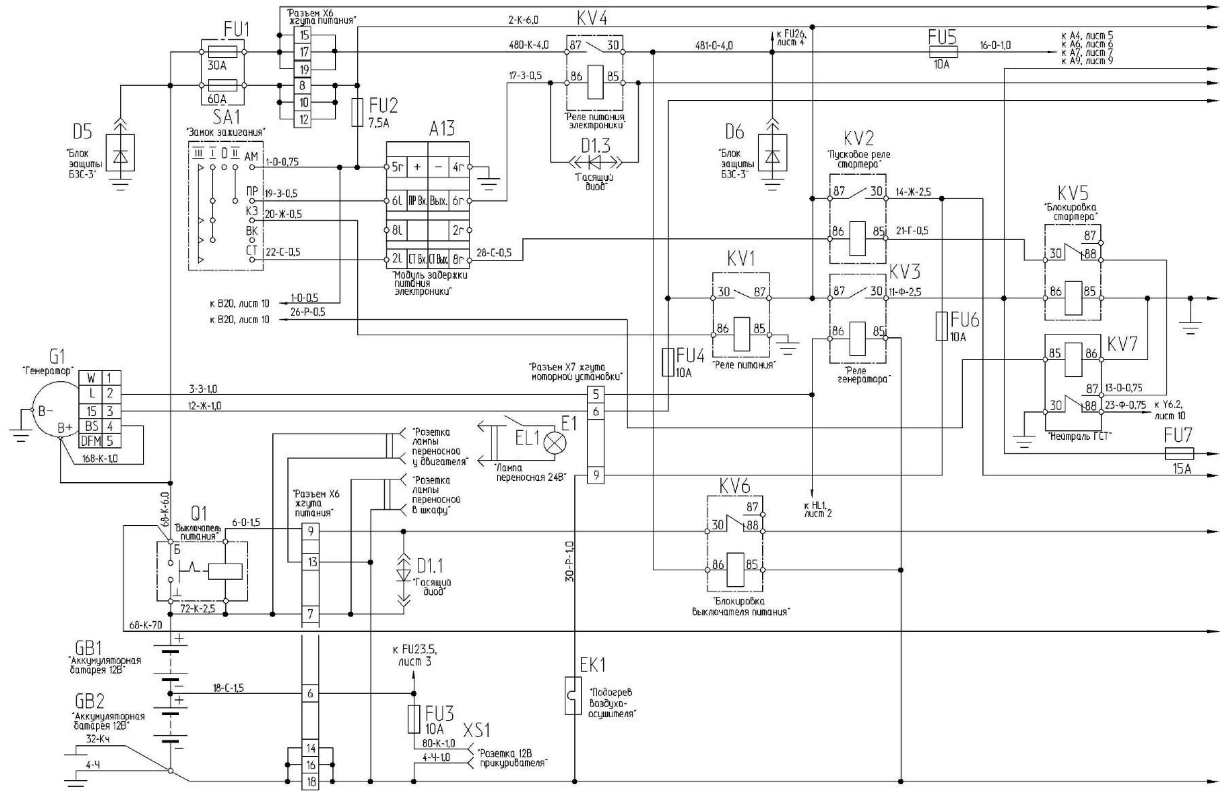
Рисунок В.1 – Схема электрическая принципиальная комплекса (лист 1)
