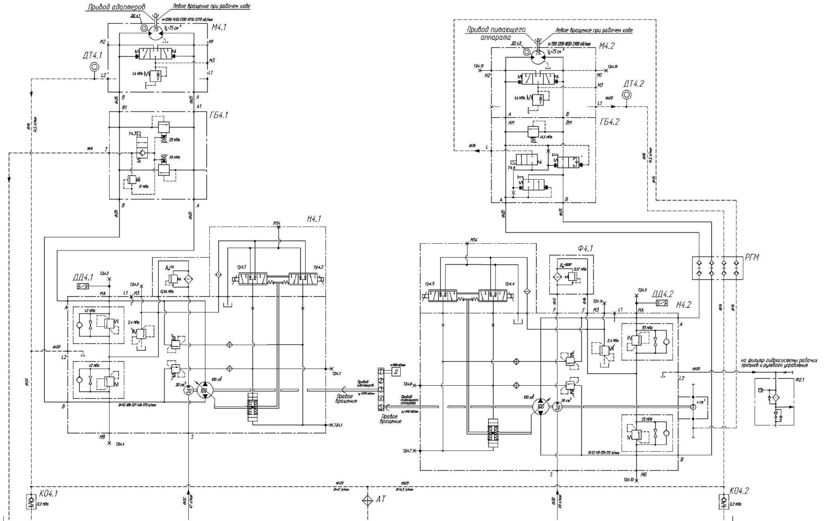
Рисунок А.3 – Схема гидравлическая принципиальная гидросистемы привода питающего аппарата и адаптеров (лист 1)
