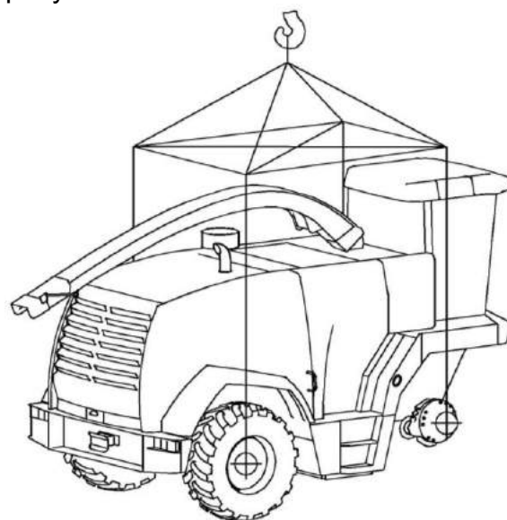
Рисунок 6.1 – Схема строповки
