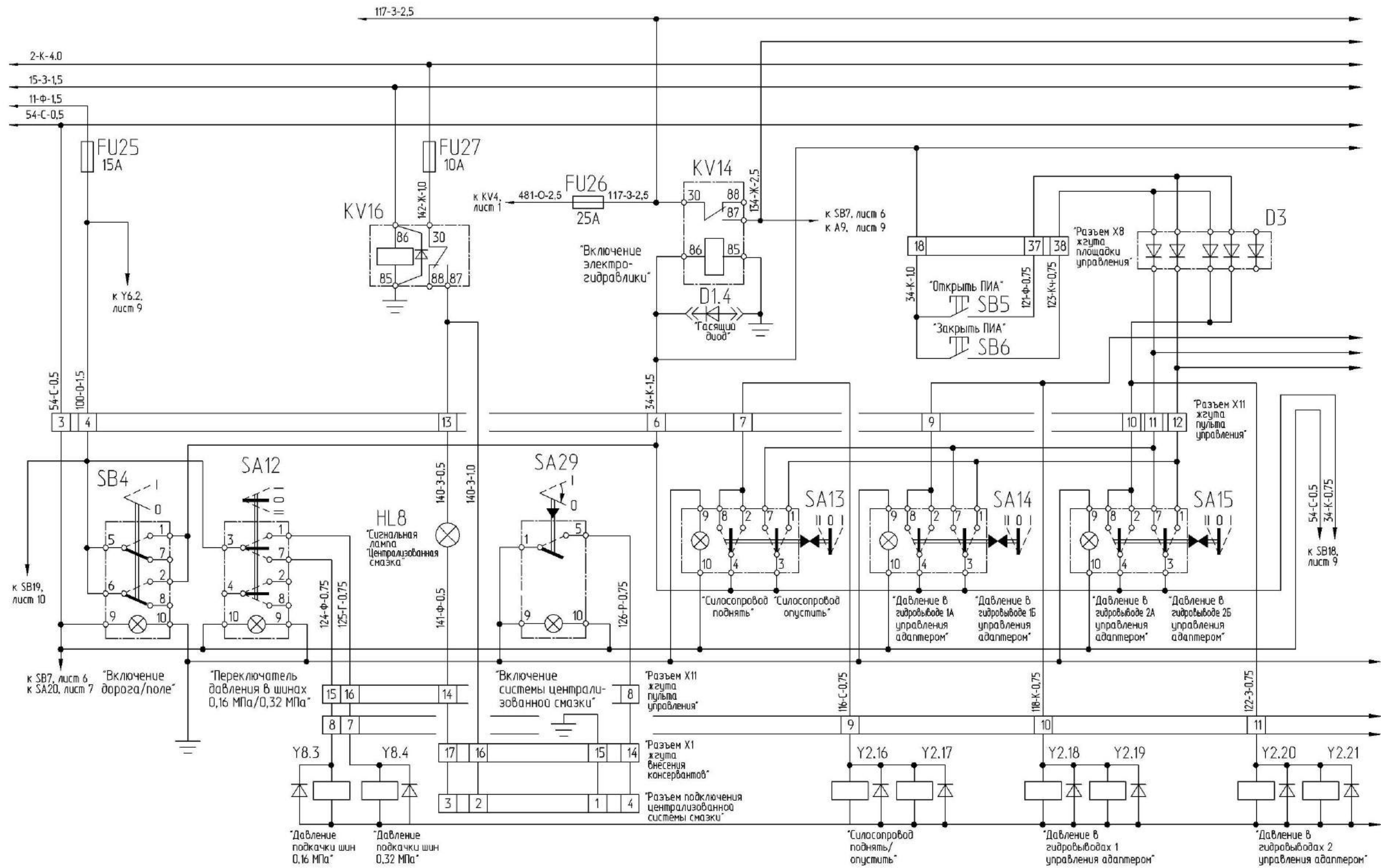
Рисунок В.4 – Схема электрическая принципиальная комплекса (лист 1)
