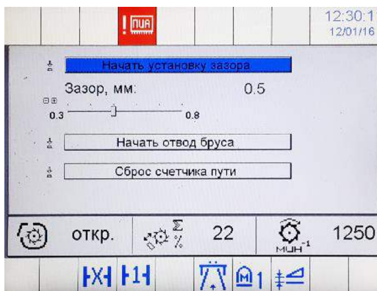
Рисунок Р.32– Меню установки зазора
