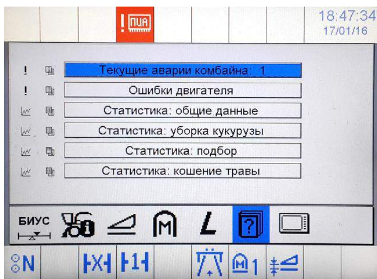
Рисунок Р.22 – «Экран прочих параметров»
