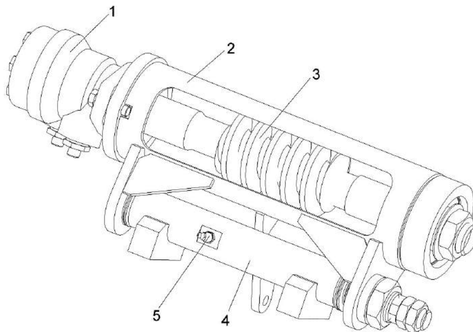
Рисунок 1.30 – Механизм поворота силосопровода
