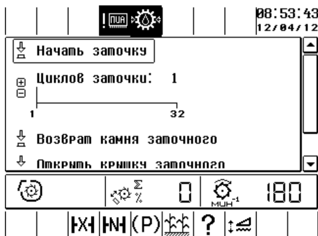
Рисунок 2.11 – Меню заточки ножей
