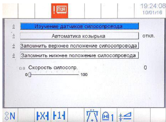
Рисунок Р.19 – Установки автоматике силосопровода
