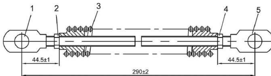
Рисунок 2.21 – Ременные передачи приводов вентилятора и компрессора
