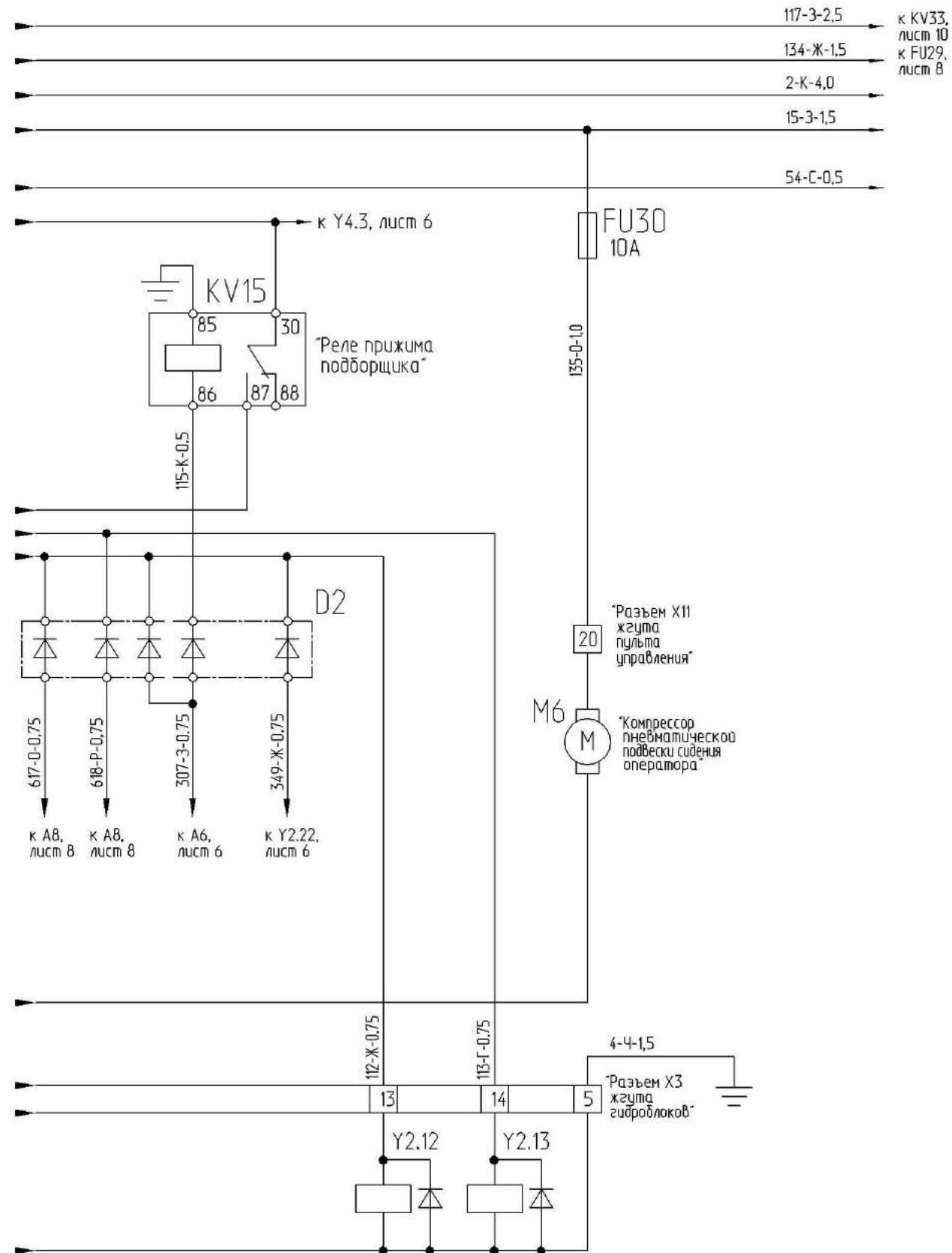
Рисунок В.4 – Схема электрическая принципиальная комплекса (лист 2)
