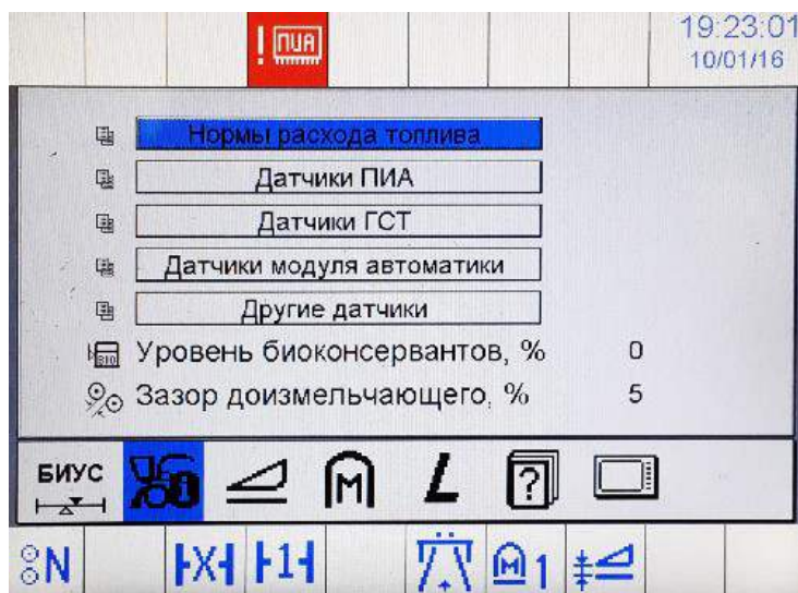
Рисунок Р.11 – Экран прочих параметров
