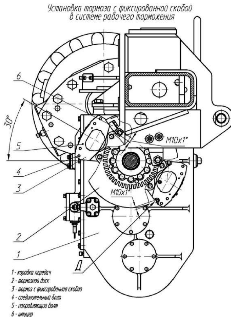
Рисунок С.1 – Схема установки
