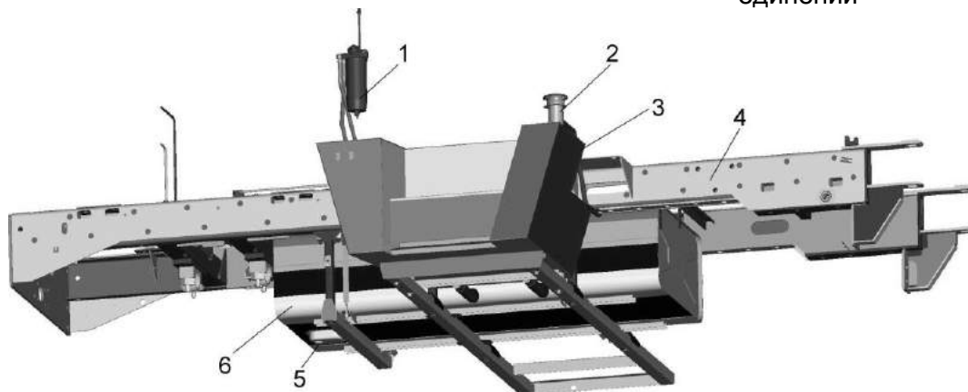
Рисунок 3.11 - Смазка ротационных соединений
