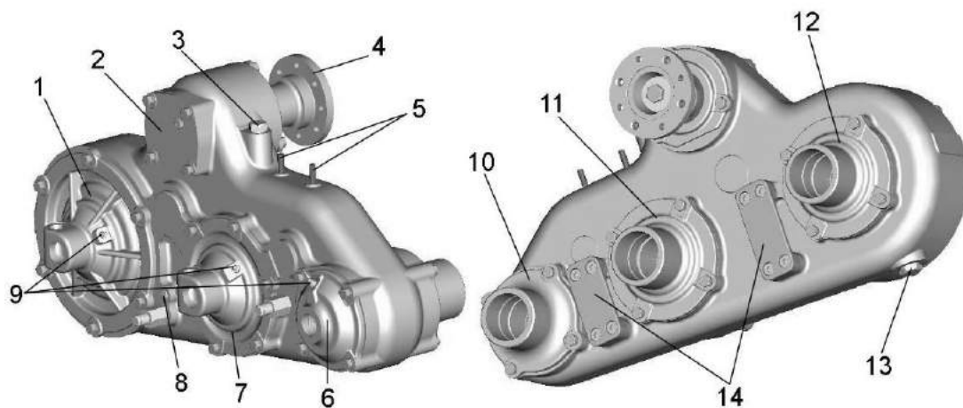
Рисунок 1.15 – Редуктор привода питающего аппарата
