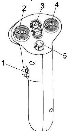
Рисунок 1.83 – Рукоятка управления скоростью движения (рукоятка ГСТ)
