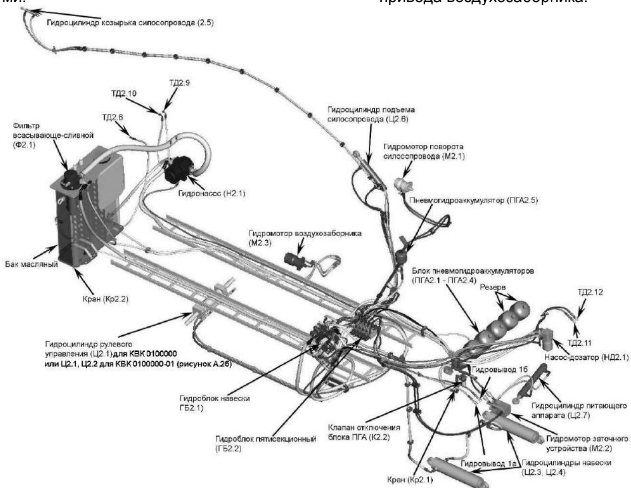
Рисунок 1.38 – Гидросистема рулевого управления и силовых гидроцилиндров
