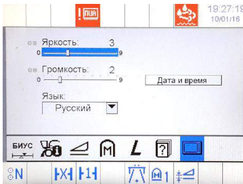
Рисунок Р.29 – Установки терминала
