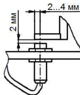
Рисунок 2.13 – Установка датчика положения бруска абразивного
