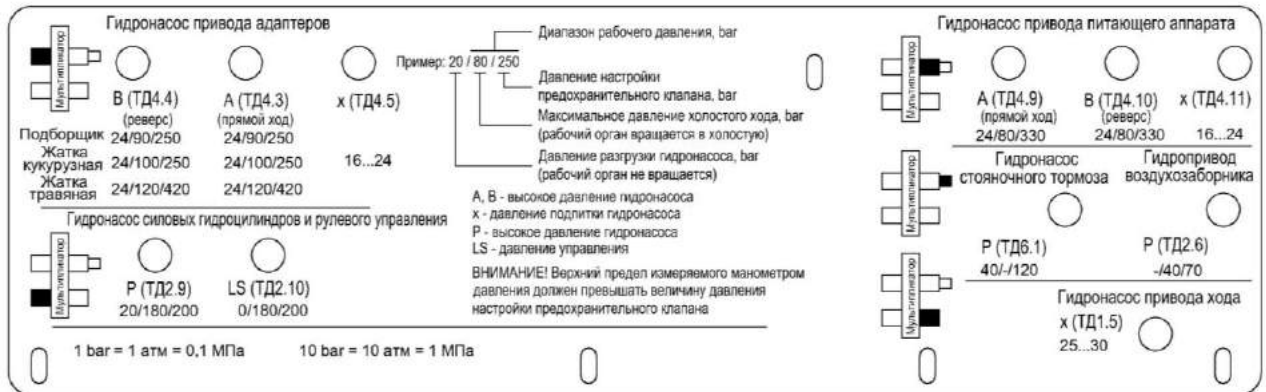
Рисунок 1.59 – Гидросистема привода питающего аппарата и адаптеров
