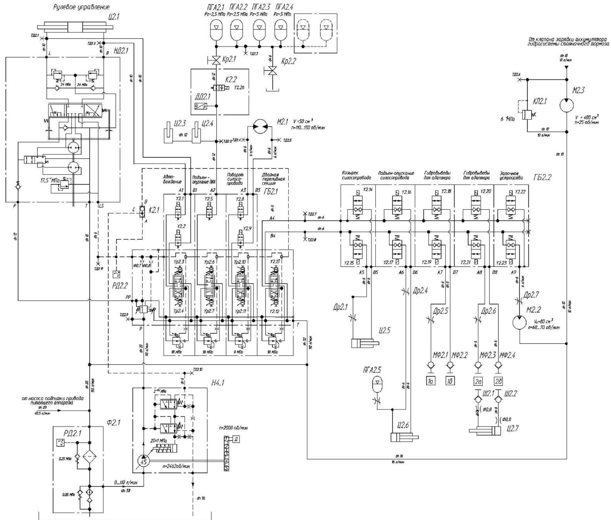
Рисунок А.2 – Схема гидравлическая принципиальная гидросистемы рулевого управления и силовых гидроцилиндров (лист 1)
