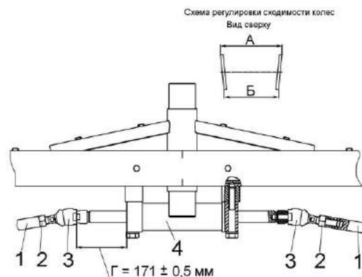
1 - тяги; 2 - гайки; 3 - шарниры; 4 - гидроцилиндр
