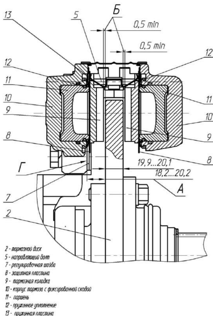
Рисунок С.2 – Монтаж тормоза
