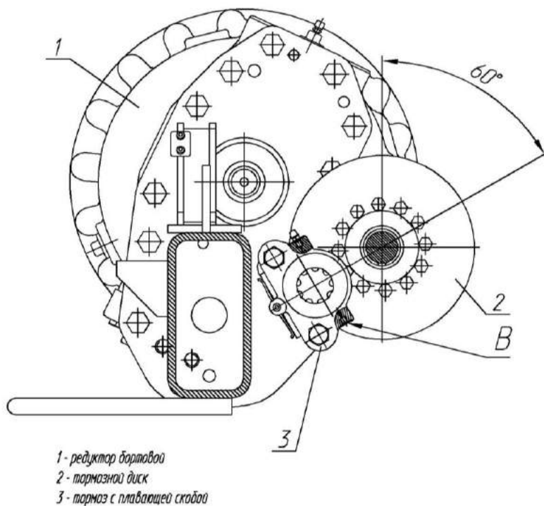
Рисунок С.3 – Схема установки
