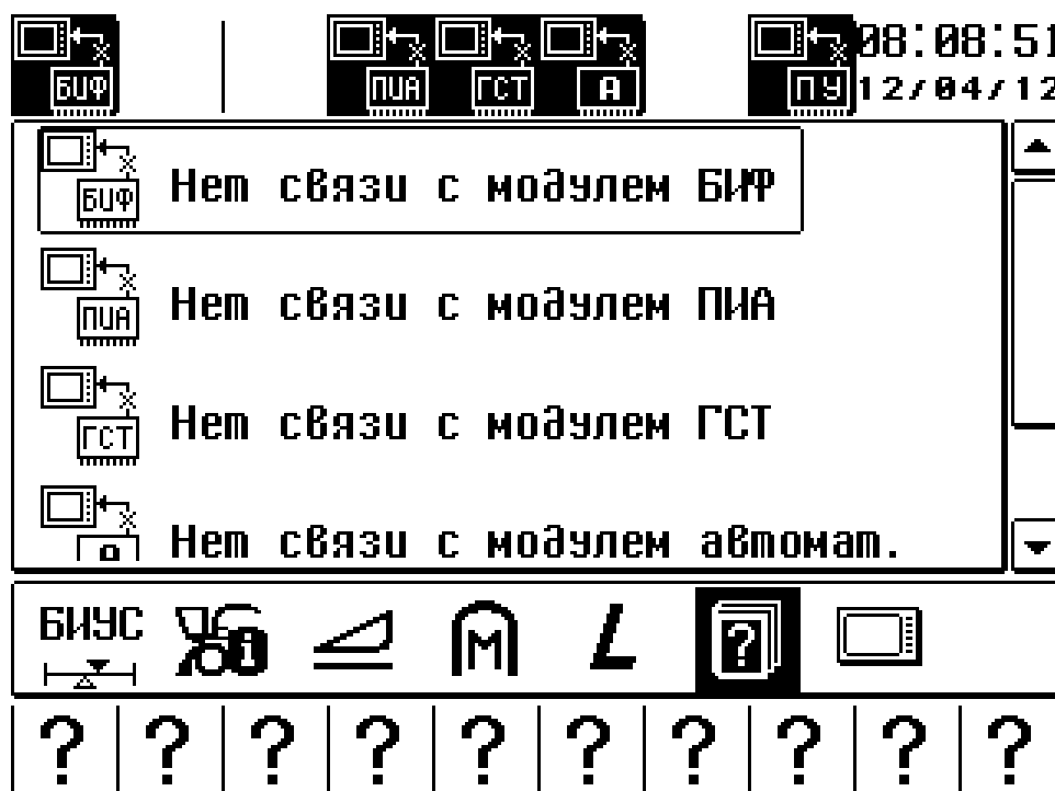
Рисунок Ж.17 – Текущие аварии и ошибки
