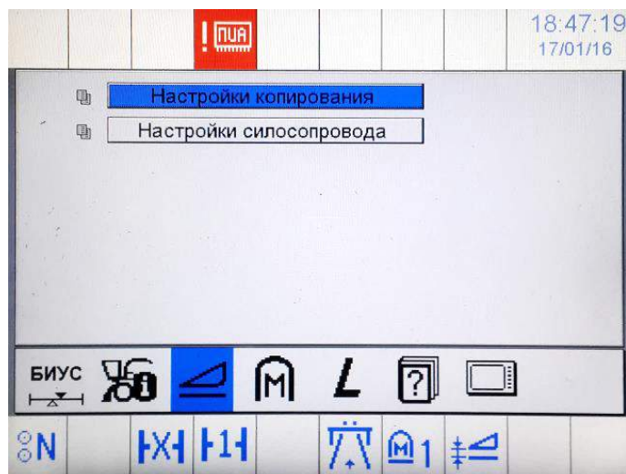
Рисунок Р.17 – Экран «Установки системы копирования и автоматики силосопровода»
