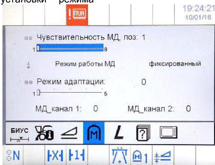
Рисунок Р.20 – Установки металлодетектора
