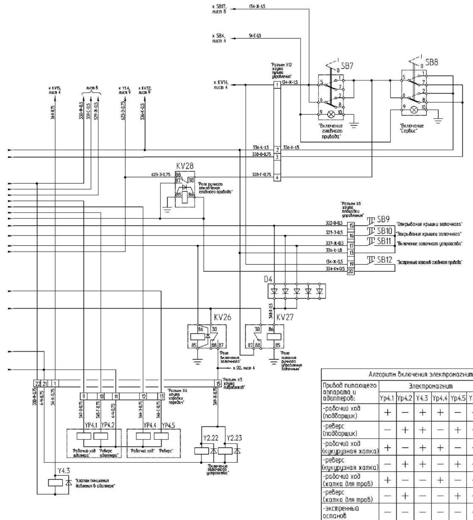
Рисунок В.6 – Схема электрическая принципиальная комплекса (лист 2)
