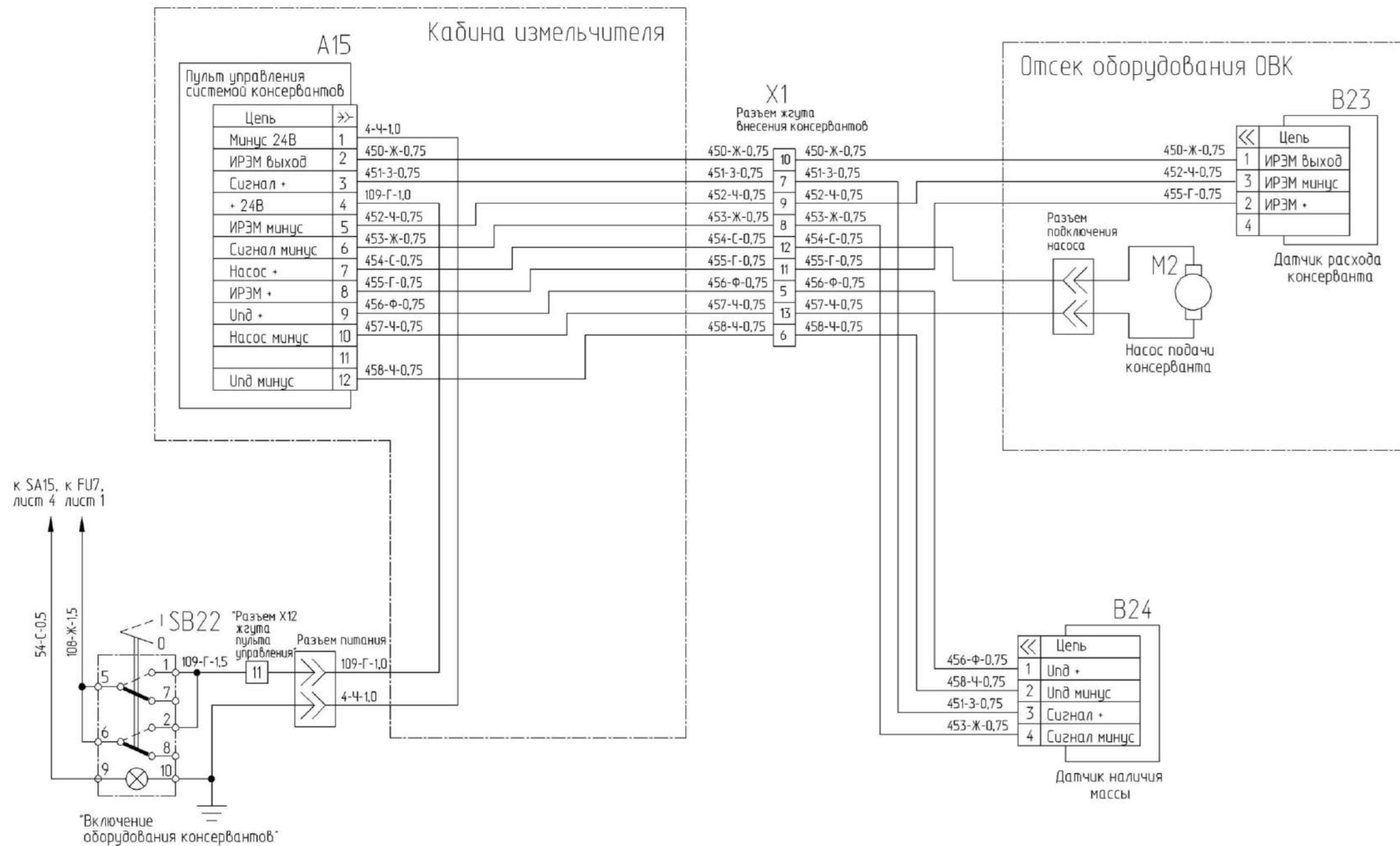
Рисунок В.10 – Схема электрическая принципиальная комплекса
