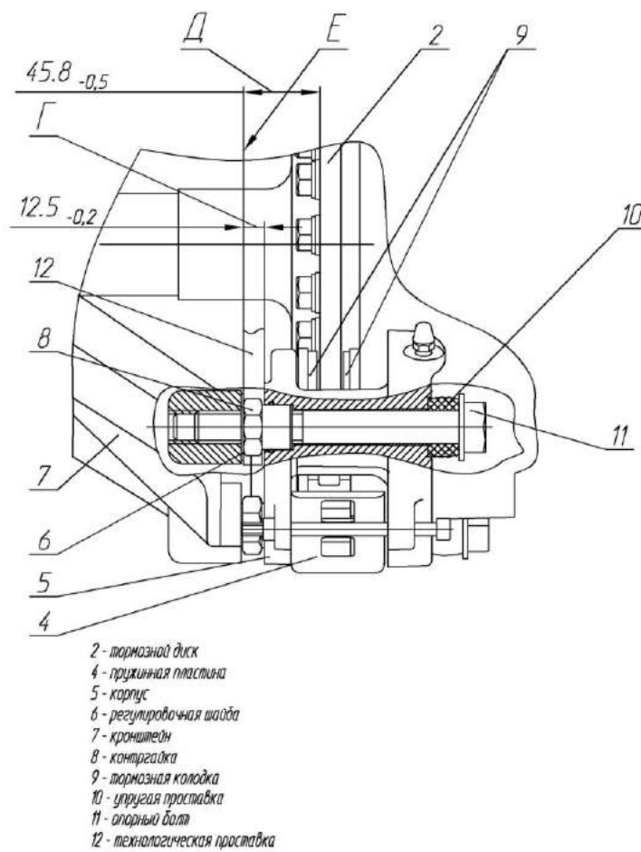
Рисунок С.4 – Монтаж тормоза на бортовом редукторе
