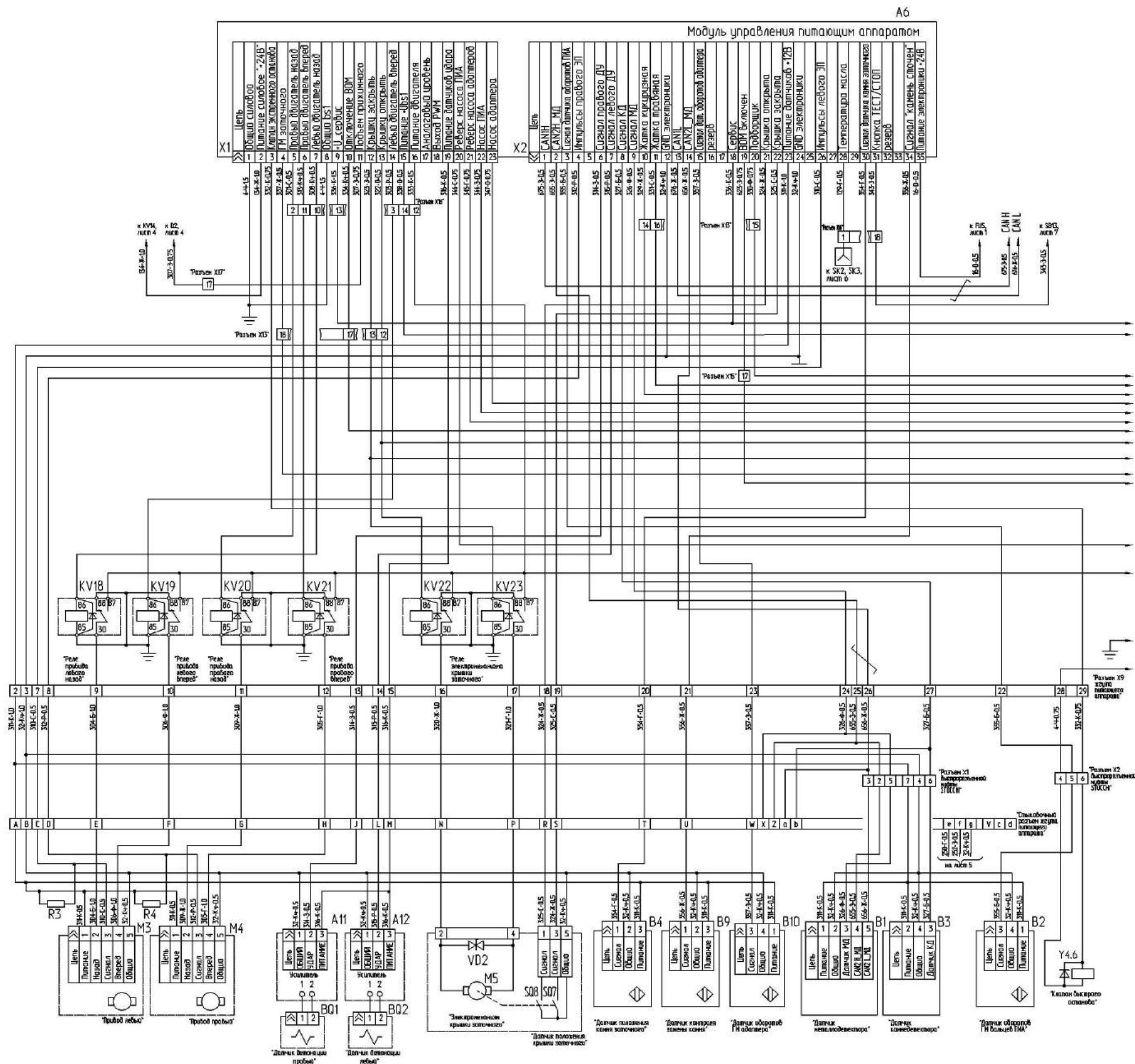
Рисунок В.6 – Схема электрическая принципиальная комплекса (лист 1)
