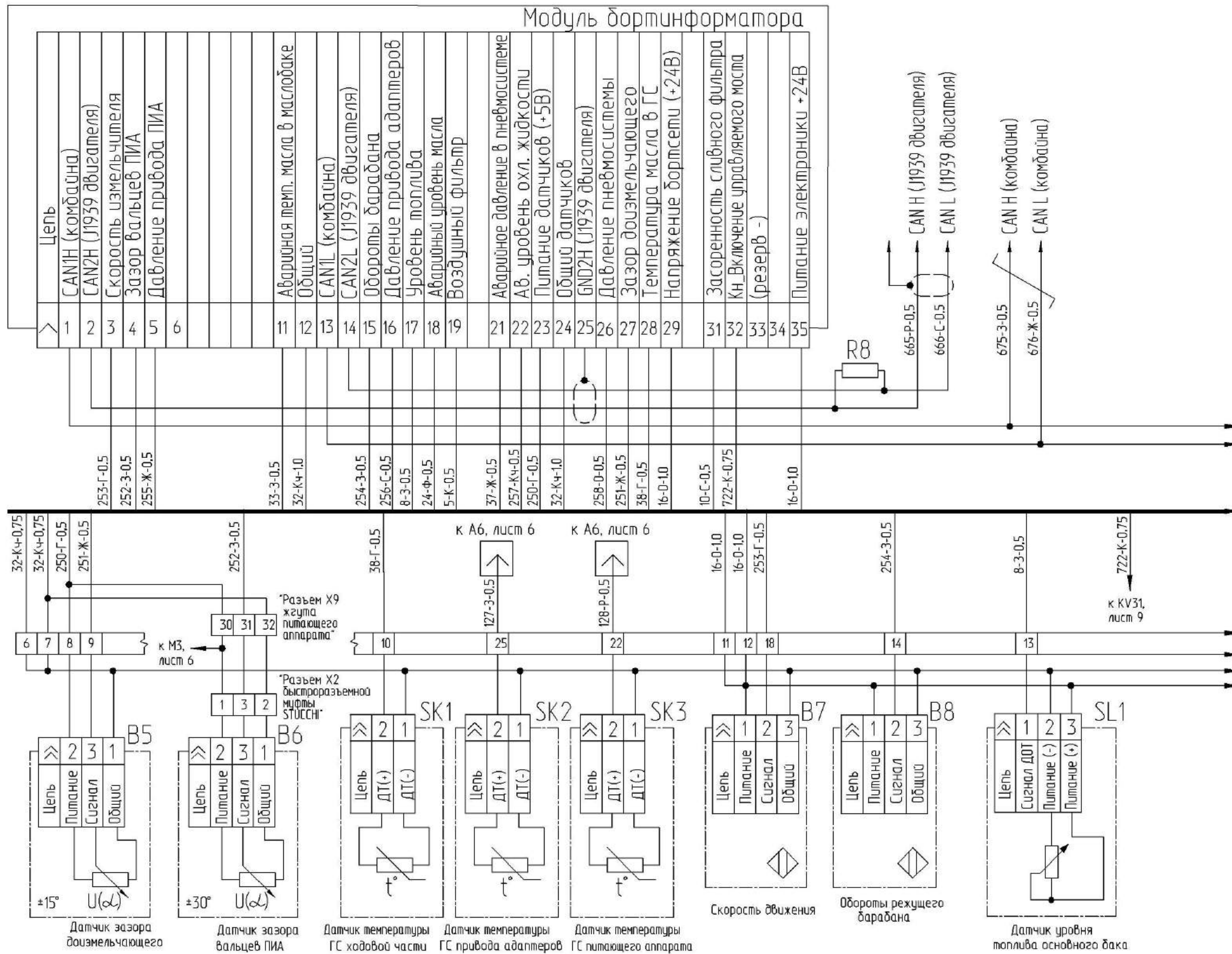
Рисунок В.5 - Схема электрическая принципиальная комплекса (лист 1)
