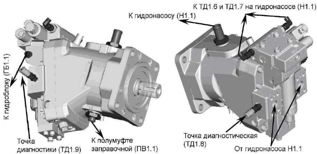
Рисунок 1.36 – Гидромотор привода ходовой части (М1.1)
