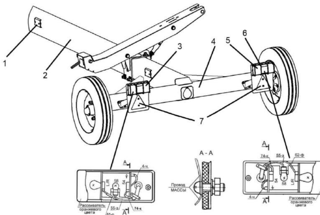
1, 7 - световозвращатели; 2 – рама тележки; 3, 5 - фонари; 4 – балка габаритная; 6 - решетка Условные обозначения цветов проводов: 3 – зеленый; К – красный; Р – розовый; Ф – фиолетовый; Ч - черный
