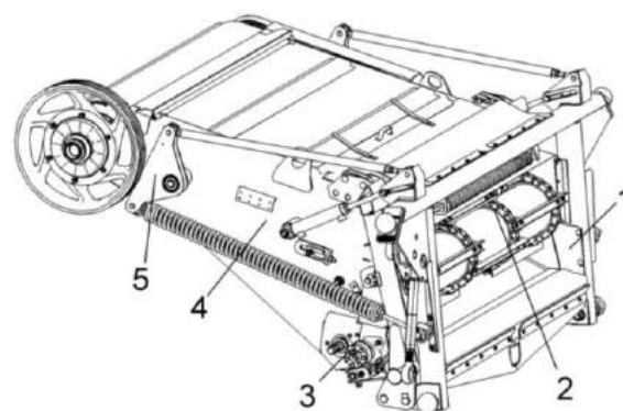
Рисунок 1.7 - Молотилка самоходная
