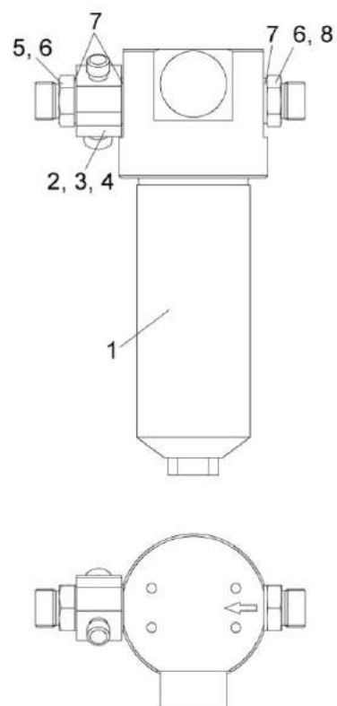
Рисунок 1.24 – Фильтр сливной
