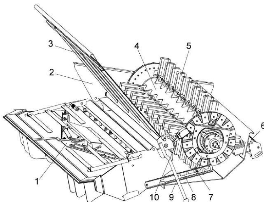
1 – дефлектор; 2 – корпус измельчителя; 3 – заслонка; 4 – ротор измельчителя; 5 – нож; 6 – ножевая опора; 7, 10 – гайки; 8 – полз; 9 - рукоятка сектора
