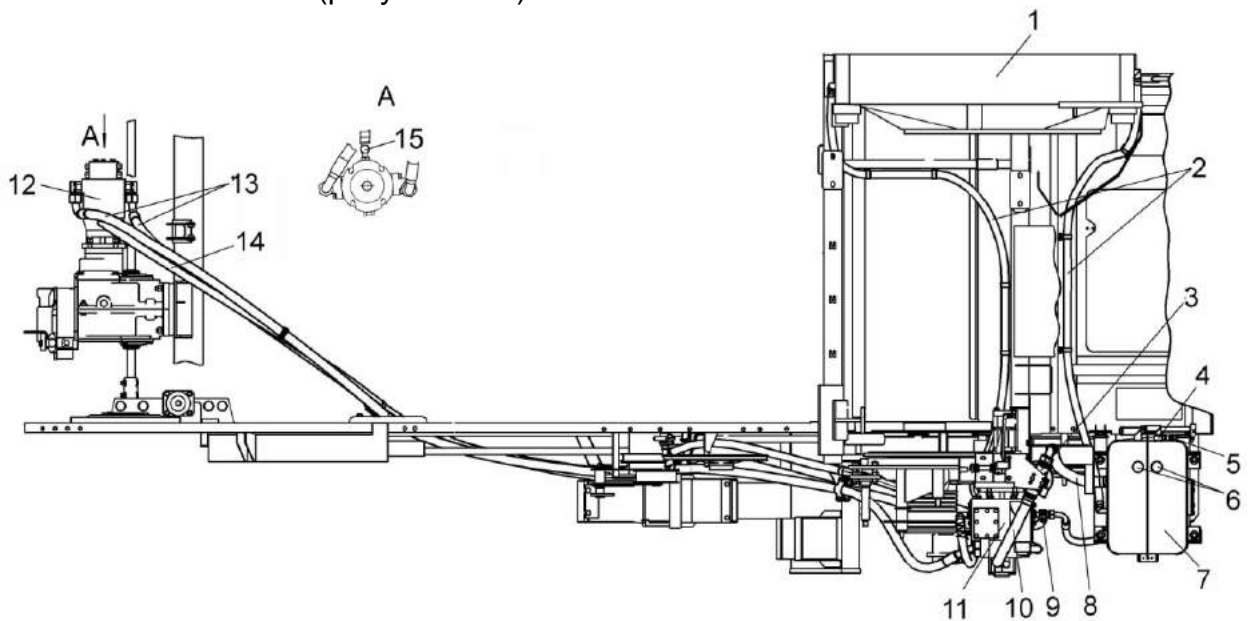
1 – блок радиаторов масляный; 2, 14 – рукава; 3 – фильтр всасывающий; 4 - маслоуказатель; 5 – датчик сигнализатора температуры; 6 – сапуны; 7 – бак масляный; 8, 10 – рукава всасывающие; 9 – датчик указателя температуры; 11 – насос аксиально–поршневой; 12 – гидромотор аксиально–поршневой нерегулируемый; 13 – рукава высокого давления; 15 – полумуфта заправочная
