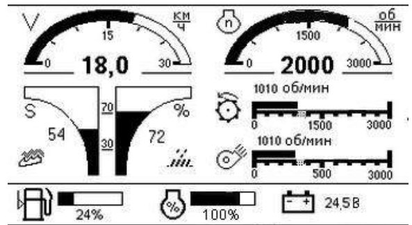
Рисунок 1.92 – Экран технологического режима уборки (комбайнирования)
