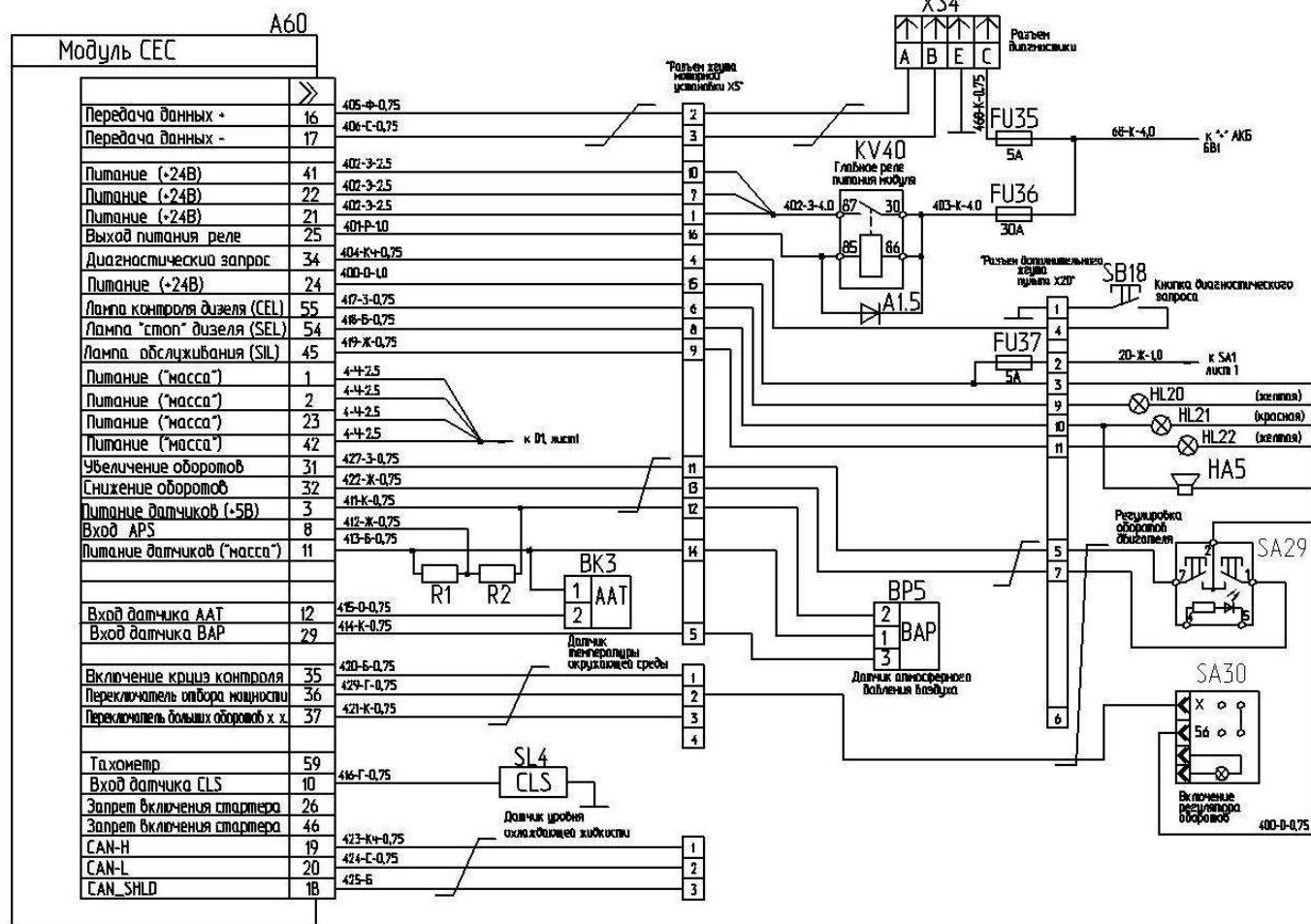
Схема для исполнения с двигателем NAVISTAR
