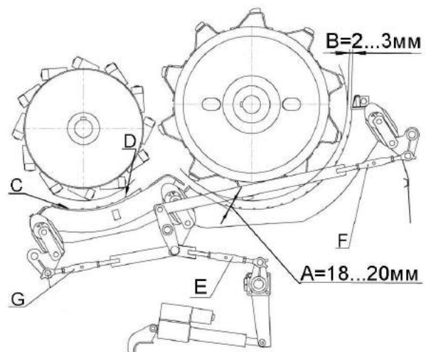
Рисунок 2.19 - Схема молотильного аппарата
