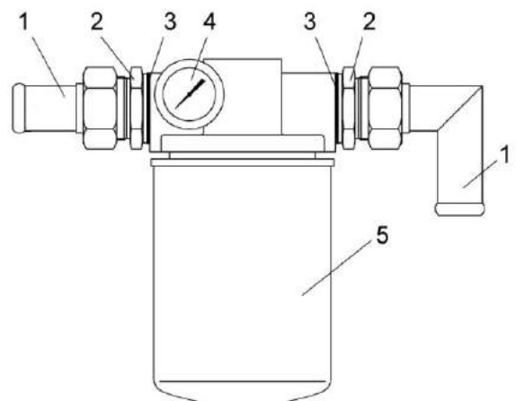
1 – хомут стяжной; 2 – штуцера; 3 – прокладки; 4 – вакуумметр; 5 – фильтр
