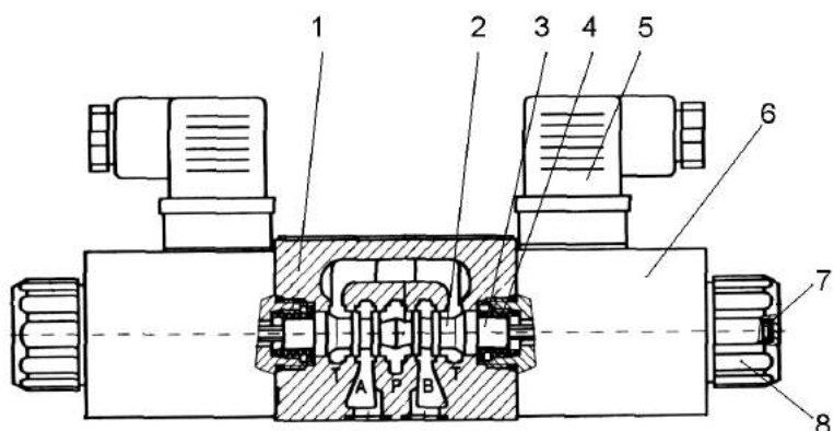
Рисунок 1.20 - Гидрораспределитель
