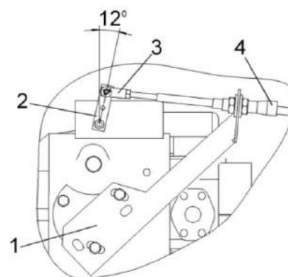
Рисунок 2.24 – Блок управления
