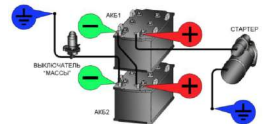
Подключение аккумуляторных батарей
