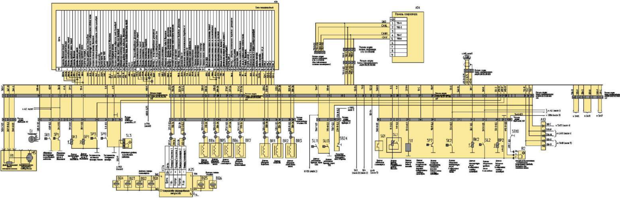
Вариант подключения компьютера бортового "Вулкан-04"
