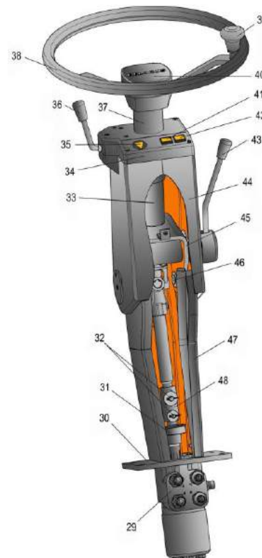
Рулевая колонка
