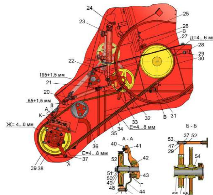
Привод выгрузки
