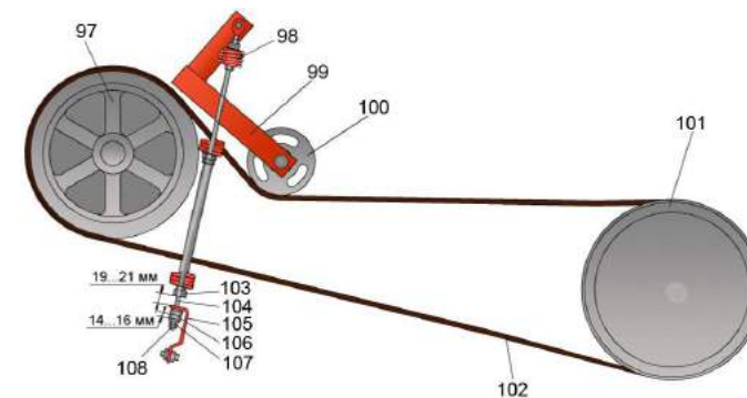
Привод отбойного битера
