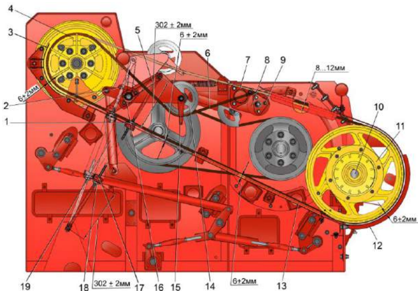
Привод наклонной камеры
