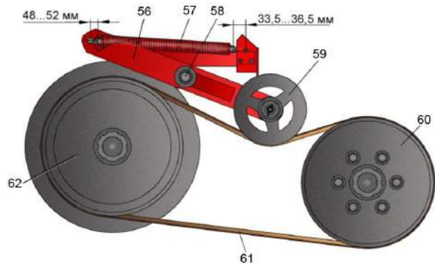
Привод ускоряющего барабана
