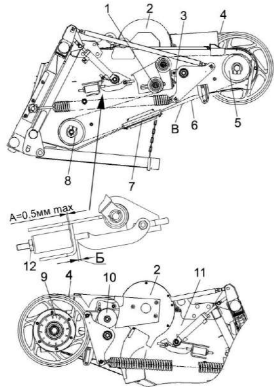
1, 5, 8 – звездочки; 2 – вентилятор; 3 – винт; 4 – ременная передача; 6 – цепная передача; 7 – успокоитель; 9 – муфта предохранительная; 10 – ролик натяжной; 11 – рама; 12 – гайка
