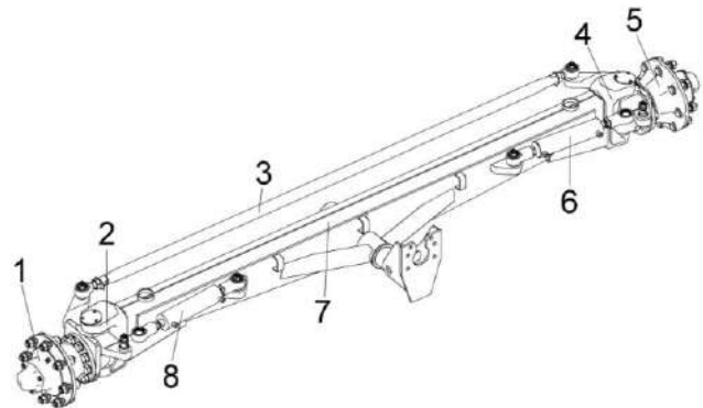
Рисунок 1.14 – Шасси
