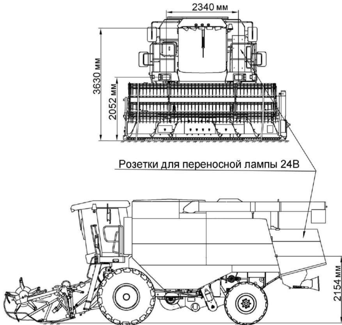
Рисунок 1.30 – Расположение наружного освещения и световой сигнализации комбайна
