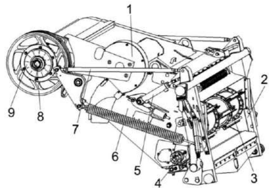
Рисунок 1.7 - Молотилка самоходная
