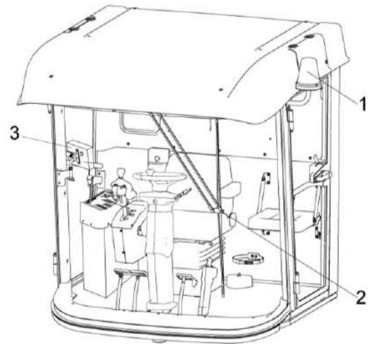
1 – проблесковый маяк; 2 – стеклоочиститель; 3 – модуль терминальный графический
