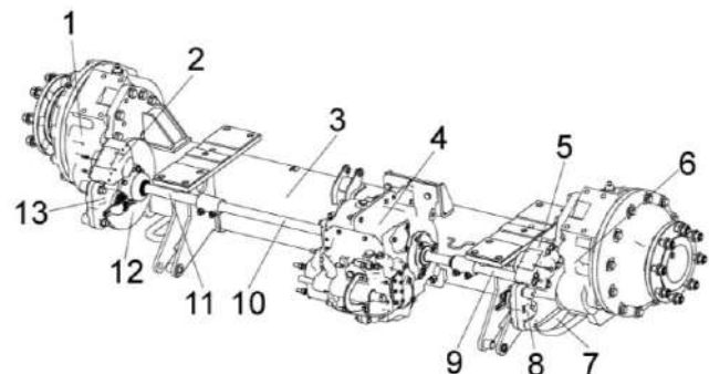
Рисунок 1.15 - Мост управляемых колес.
