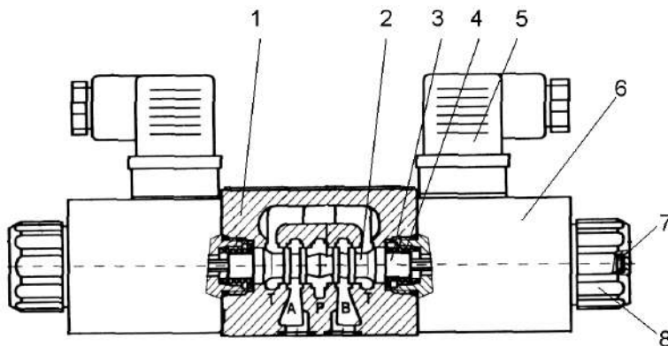
Рисунок 1.21 – Гидрораспределитель
