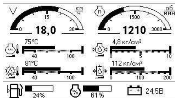
Рисунок 1.93 – Экран транспортного режима
