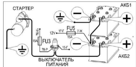
Рисунок 2.2 - Подключение аккумуляторных батарей
