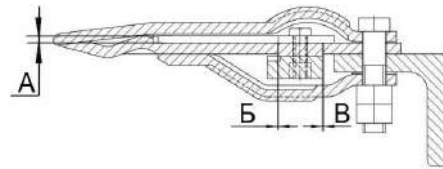
Рисунок 2.43 – Режущий аппарат
