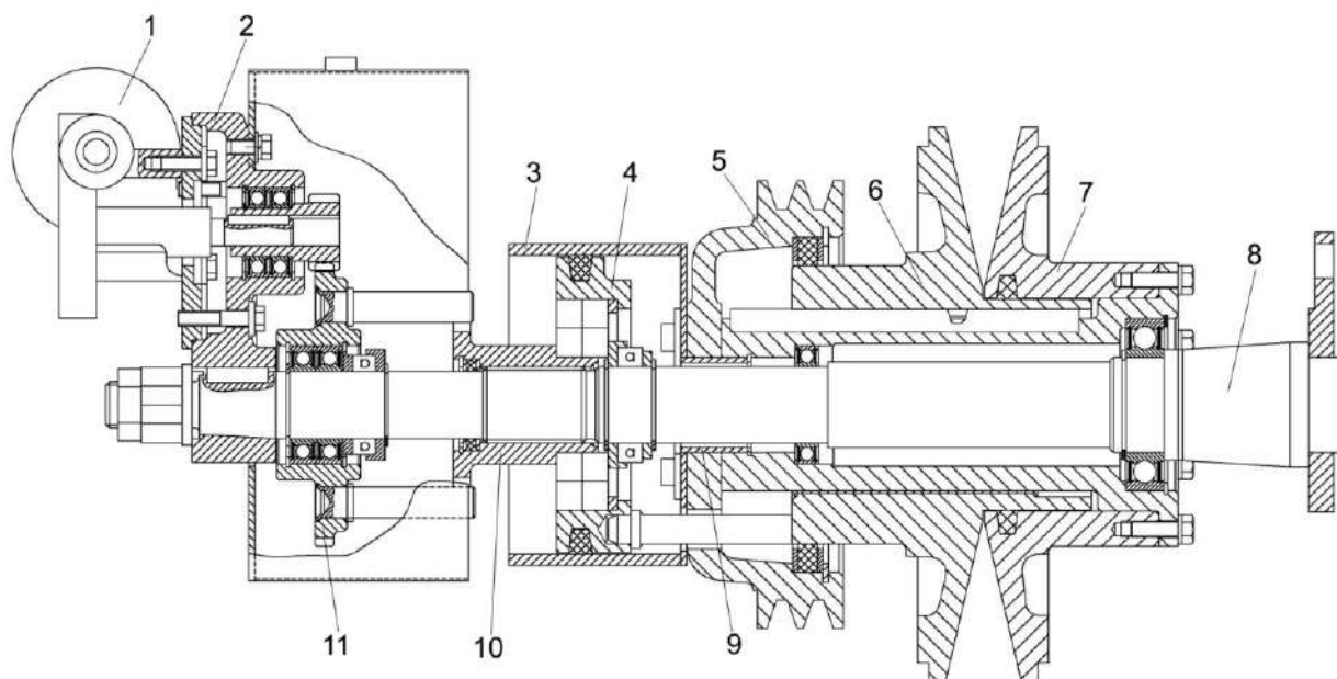
Рисунок 2.21 – Контрпривод вариатора
