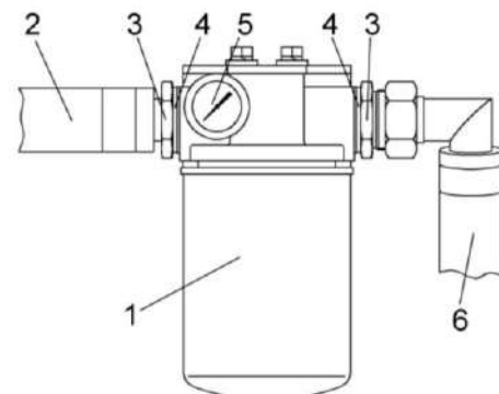
Рисунок 1.27 – Гидросистема привода ходовой части
