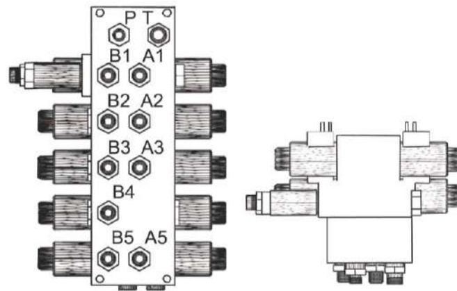
Рисунок 1.23 - Гидроблок пятисекционный
