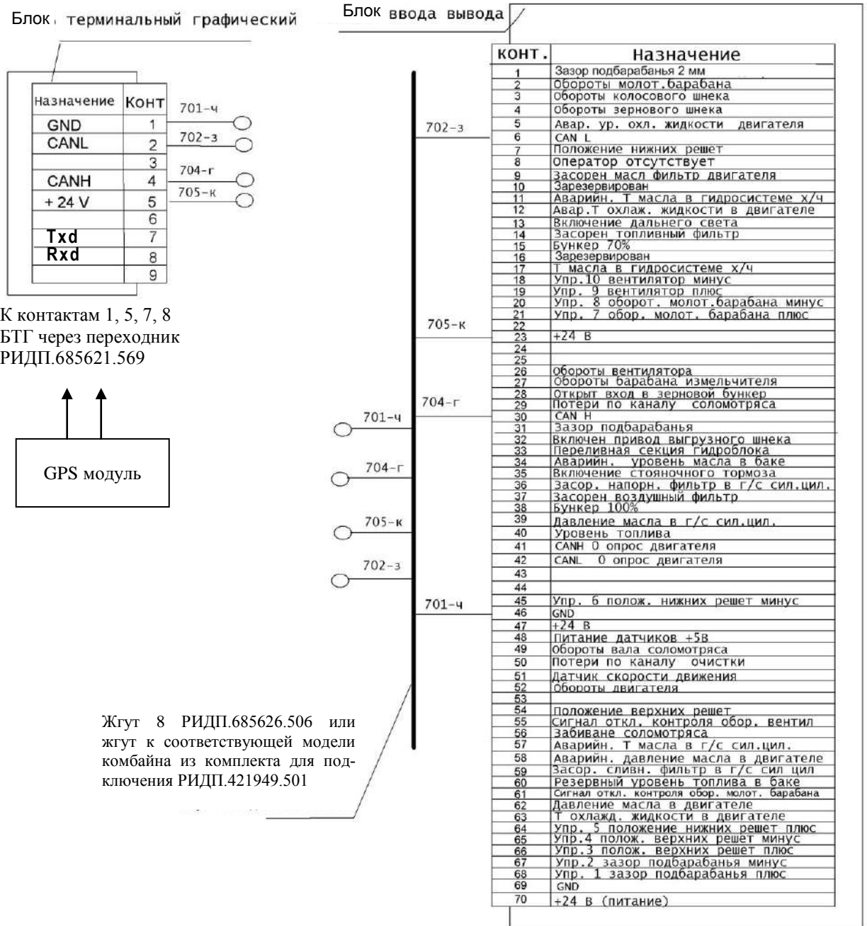
Рисунок 1.145 – Схема подключения БТГ, БВВ и GPS модуля комбайна
