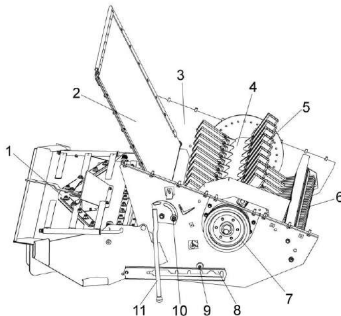
Рисунок 1.19 – Соломоизмельчитель
