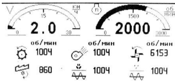
Рисунок 1.94 – Экран оборотов рабочих органов
