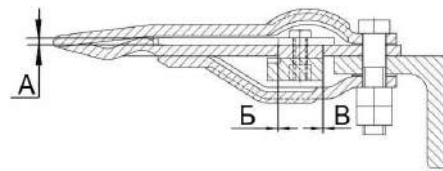
Рисунок 2.43 – Режущий аппарат
